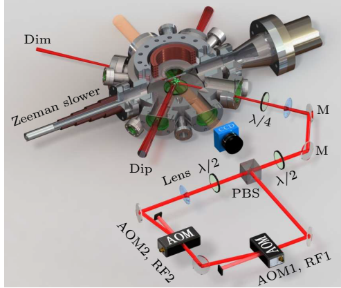
图 2 铯原子 BEC 实验装置与 Bragg 激光光路示意图. 实验中, 入射 Dim 光与其反射光被调整为完全重合, 图中第一台声光调制器驱动信号为 RF1(单频 80 MHz), 取+1 级衍射光出射. 第二台声光调制器驱动信号为 RF2(单频 80 \text{ MHz} - 5.3 \text{ kHz} ), 取-1 级衍射光出射. 在两台声光调制器作用下, 对射 Bragg 激光频率满足 |0\rangle 和 |1\rangle 动量态的共振跃迁频率. Dip, 偶极阱激光束; Dim, dimple 阱激光束; PBS, 偏振分束棱镜; AOM, 声光调制器; \lambda/4 , 四分之一波片; \lambda/2 , 二分之一波片; Lens, 平凸透镜; Mirror, 反射镜
