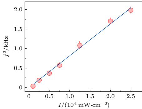
图4 双光子 Bragg 散射振荡频率平方 f^2 与 Bragg 激光光强 I 的对应关系, 实验上可通过控制声光调制器衍射效率实现 Bragg 激光光强的快速调节. 图中实线为正比例函数拟合曲线, 圆点为实验数据点, 误差棒为数据标准误差
