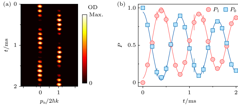
图3 双光子 Bragg 散射的动力学演化 (a) 相干振荡过程中, 动量为 0 和 2\hbar k 的原子团分布随 Bragg 脉冲时间 t 变化的吸收成像图; (b) 动量态 |0\rangle ( |1\rangle ) 分布概率 P_0 ( P_1 ) 随 Bragg 脉冲时间 t 的时间演化结果, 图中实线为数据拟合结果, 圆形和方形点为数据点, 误差棒代表标准误差. 实验中, 动量态之间的耦合强度为 J = \hbar \times 615 Hz, 通过拟合实验参数得到双光子振荡动力学相干时间为 4.1(2) ms
