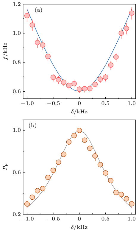
图 5 双光子 Bragg 散射振荡频率 f 和振荡幅值 P_F 与拉曼激光失谐 \delta 的对应关系, 当 \delta = 0 时, 通过控制 Bragg 激光光强, 设置动量态耦合强度为 J = \hbar \times 600 Hz, 图中实线为数值计算结果, 圆点为实验数据点, 误差棒为数据标准误差
