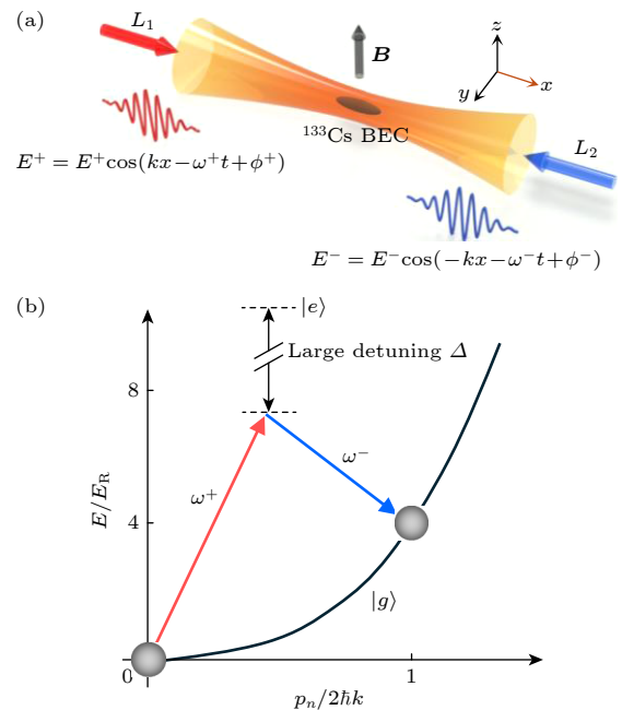
图 1 双光子 Bragg 散射实验方案 (a) 一对反向传播的单频红失谐激光场共同作用于 ^{133}\text{Cs} BEC, 其相位、频率及振幅均可独立调控; (b) 能量-动量色散关系. 拉曼激光与基态 |g\rangle 和激发态 |e\rangle 之间的原子共振频率远失谐. 双光子 Bragg 散射的共振条件满足二次型自由粒子色散关系, 其中 |g, 0\rangle 和 |g, 2\hbar k\rangle 动量态之间的频率失谐量 \Delta\omega = 4E_R/\hbar = 5.3 kHz
