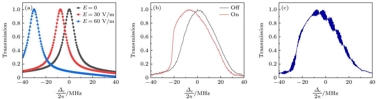
图 3 (a) 理论计算的 EIT 光谱, 外加电场强度分别是 0, 30 和 60 V/m; (b) 黑色曲线为射频电场关闭时的 EIT 光谱, 红色曲线为射频电场开启且 P = 15 \text{ dBm} 时的 EIT 光谱, EIT 光谱向左偏移约 8 MHz; (c) 同时施加本振场和信号场时的 EIT 光谱, 光谱信号由两个电场的拍频信号以 \Delta\omega = 100 \text{ kHz} 进行调制, 其中 f_{LO} = 10.1 \text{ MHz} , f_{sig} = 10 \text{ MHz} ; 图中的透射率已归一化
