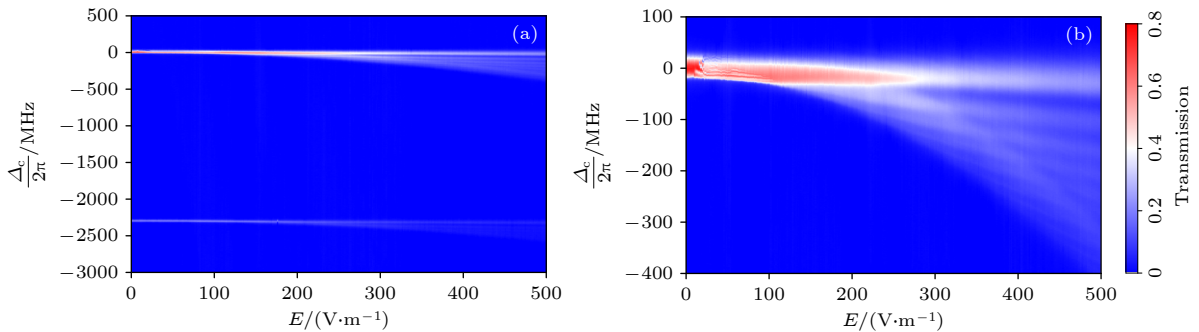
图 2 (a) 不同强度的 10 MHz 的正弦射频电场作用下 Rydberg 原子的 EIT 光谱; (b) 射频电场中 |49P_{3/2}\rangle 态 Rydberg 原子的 EIT 光谱特征
