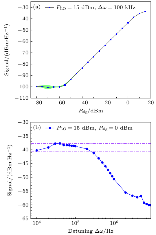
图 4 (a) 系统在 P_{\text{LO}} = 15 dBm 和 \Delta\omega = 100 kHz 时的动态范围, 在 65 dB 的范围内, 拍频信号强度与输入功率之间呈现线性关系; (b) 系统在 P_{\text{LO}} = 15 dBm 和 P_{\text{sig}} = 0 dBm 条件下的瞬时带宽. 随着信号场与本振场之间的失谐量逐渐增大, 拍频信号的强度持续减弱, 考虑到负失谐情况的基础上, 测得 3 dB 带宽为 0.6 MHz
