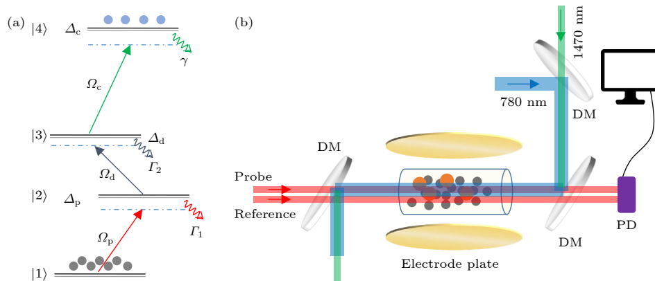
图 1 (a) 由 Cs 原子基态 |1\rangle , 两个低激发态 |2\rangle 和 |3\rangle , Rydberg 态 |4\rangle 构成的梯型四能级示意图; (b) 实验装置概况, 两块铜制电极板以 4 cm 间距平行置于铯泡两侧, 其中 DM 为二向色镜, PD 为光电探测器
