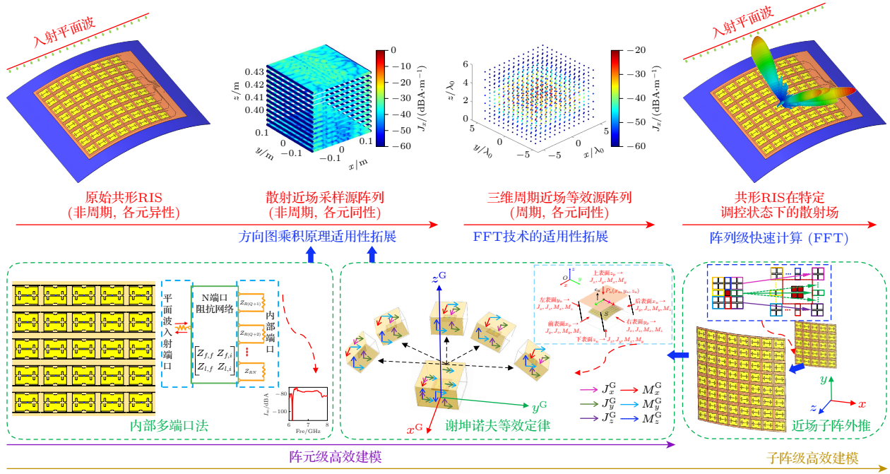
图 2 共形 RIS 的三维周期近场等效模型建模及分析方法示意图
