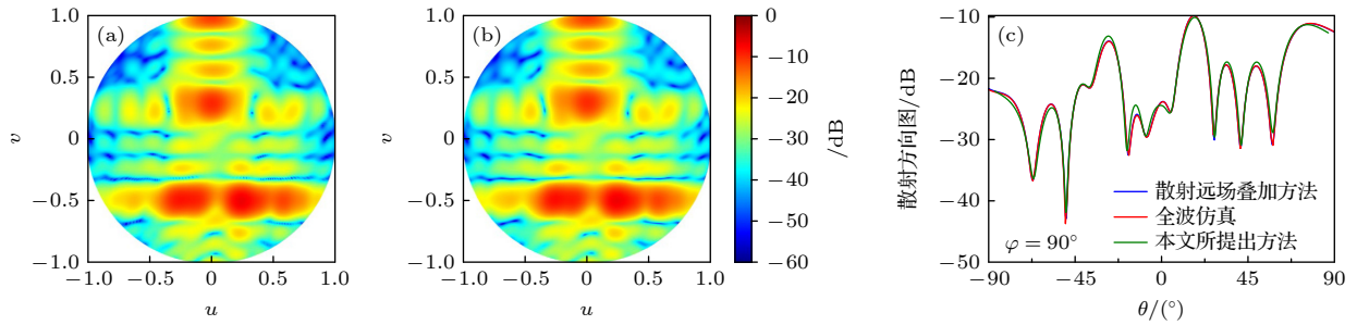
图 5 1-bit 64 元共形 RIS 的散射方向图 (a) 全波仿真结果; (b) 所提方法计算结果; (c) 剖面场分布
