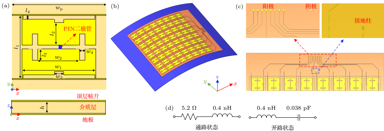
图 4 1-bit 64 元共形 RIS (a) 单元结构与 (b) 阵列布局; (c) 馈电网络; (d) PIN 二极管等效电路
