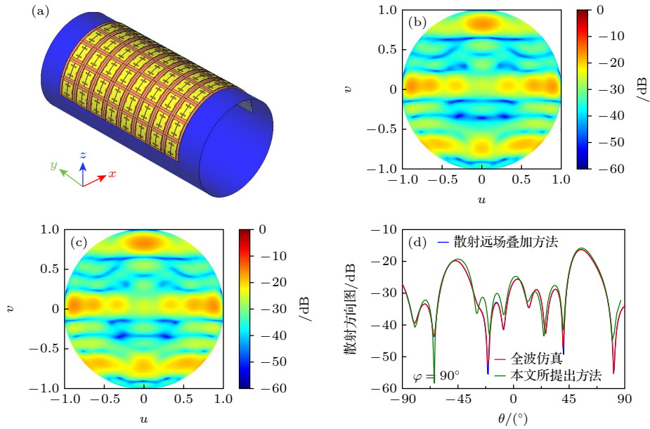
图 6 大曲率共形 RIS 结构及其散射方向图 (a) 结构示意图; (b) 全波仿真结果; (c) 所提方法计算结果; (d) 剖面场分布
