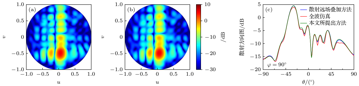
图 8 4-bit 64 元共形 RIS 的散射方向图 (a) 全波仿真结果; (b) 所提方法计算结果; (c) 剖面场分布
