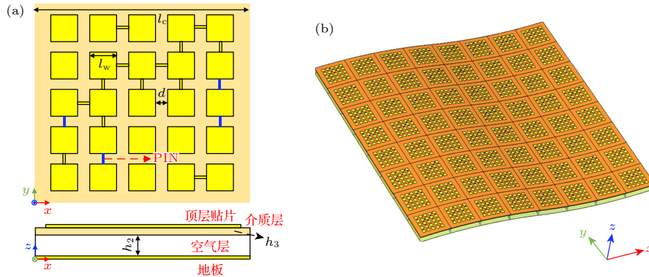
图 7 4-bit 64 元共形 RIS (a) 单元结构; (b) 阵列布局
