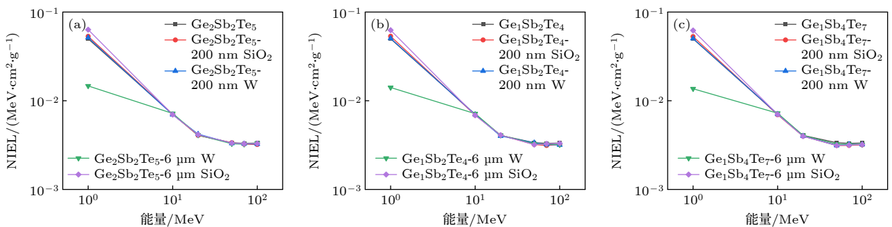
图 6 1—100 MeV 质子经屏蔽层后 GST 层的非电离能量损失值比较 (a) \text{Ge}_2\text{Sb}_2\text{Te}_5 ; (b) \text{Ge}_1\text{Sb}_2\text{Te}_4 ; (c) \text{Ge}_1\text{Sb}_4\text{Te}_7
