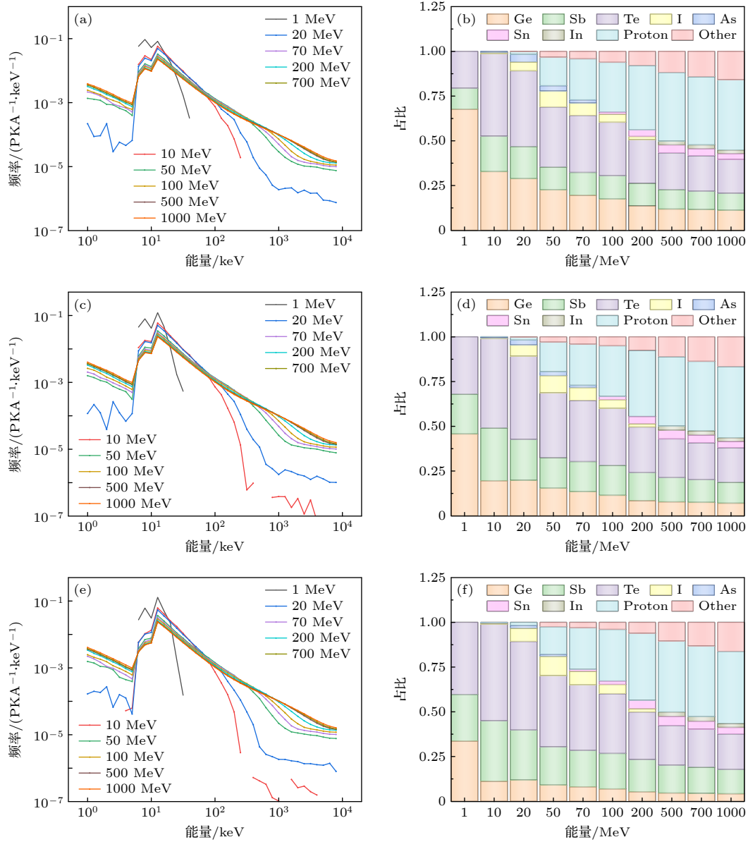
图3 PKA能量分布与种类占比 (a) \text{Ge}_2\text{Sb}_2\text{Te}_5 PKA能谱; (b) \text{Ge}_2\text{Sb}_2\text{Te}_5 PKA占比; (c) \text{Ge}_1\text{Sb}_2\text{Te}_4 PKA能谱; (d) \text{Ge}_1\text{Sb}_2\text{Te}_4 PKA占比; (e) \text{Ge}_1\text{Sb}_4\text{Te}_7 能谱; (f) \text{Ge}_1\text{Sb}_4\text{Te}_7 PKA占比
