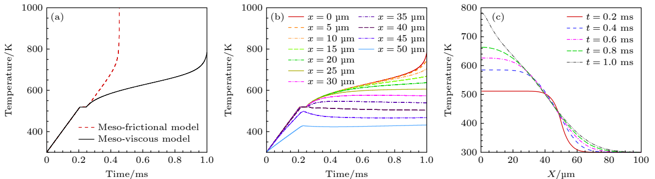
图 7 (a) P = 10 \text{ MPa} , v = 50 \text{ m/s} , h_c = 50 \mu\text{m} 裂纹中心单元的温度曲线对比图; (b) 裂纹中心附近单元的温度-时间曲线; (c) 不同时刻温度-位置曲线
