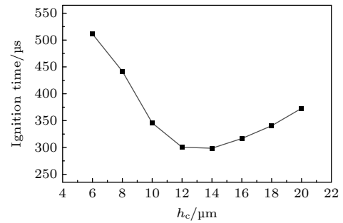
图 10 窄裂纹点火延迟时间曲线
