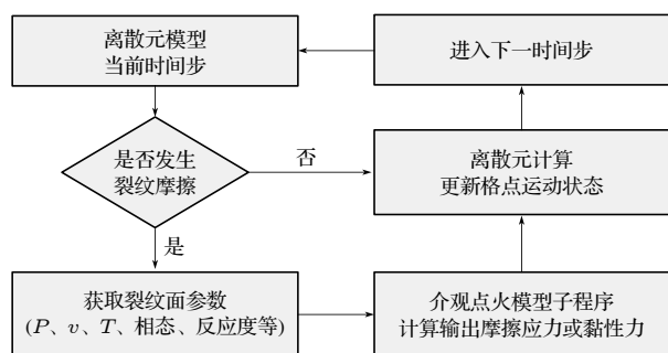
图 3 离散元宏-介观点火模型的迭代求解流程图
