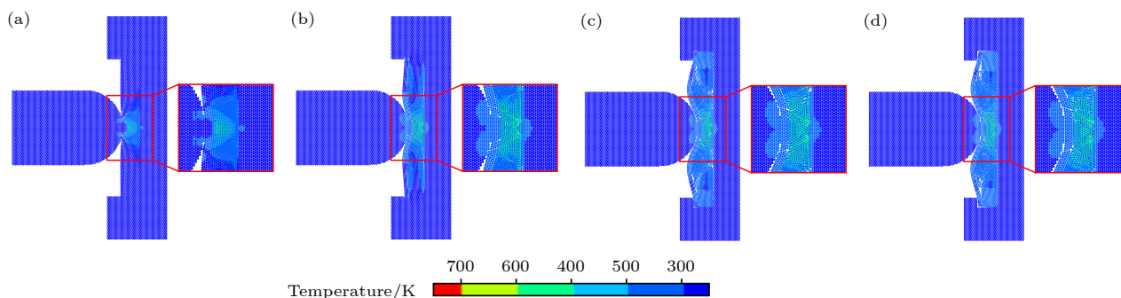
图 5 50 m/s 下的炸药温度场云图 (a) 40 \mu s; (b) 90 \mu s; (c) 180 \mu s; (d) 286 \mu s
