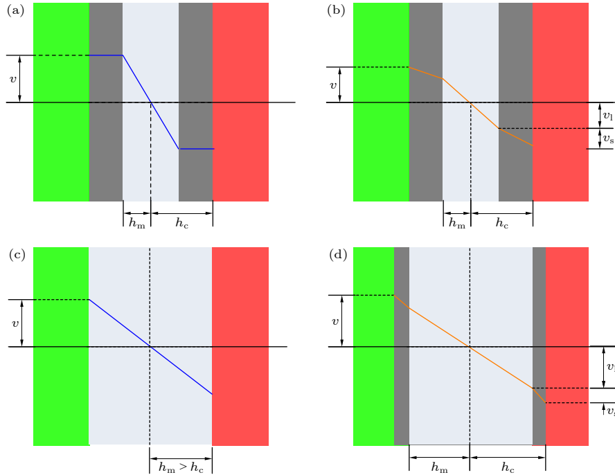
图 1 熔化后固液两相速度分配的示意图 (a) 剪切带不滑动; (b) 剪切带滑动; (c) 基体未剪切破坏; (d) 基体发生剪切破坏
