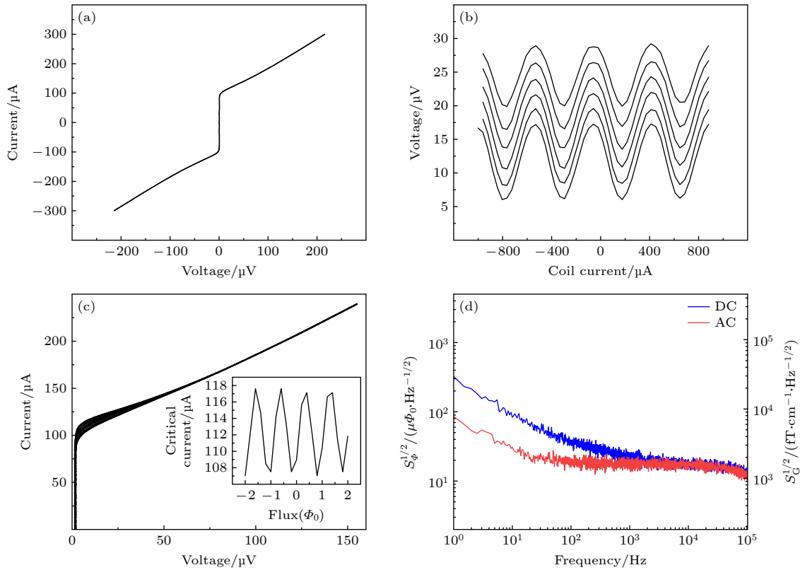
图 3 77 K 下高温超导平面梯度计的电学特性 (a) I - V 特性曲线; (b) V - \Phi 特性曲线; (c) I_c - \Phi 特性曲线; (d) 磁通及磁场噪声谱密度
