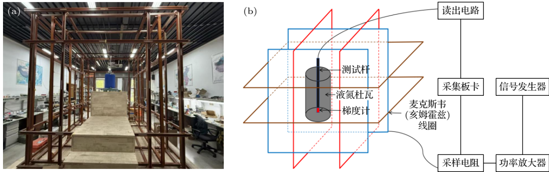
图 2 标定实验示意图 (a) 麦克斯韦 (亥姆霍兹) 线圈实物图; (b) 梯度计标定流程图
