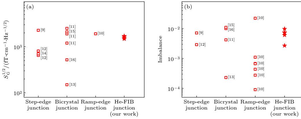
图 5 不同技术路线制备的器件性能对比 [9–16] (a) 磁场梯度分辨率对比; (b) 不平衡度对比
