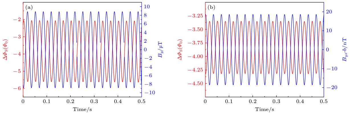
图 4 不平衡度的标定 (a) 梯度计对均匀磁场的差分磁通响应及对应的均匀磁场值; (b) 梯度计对梯度磁场的差分磁通响应及对应的梯度磁场值
