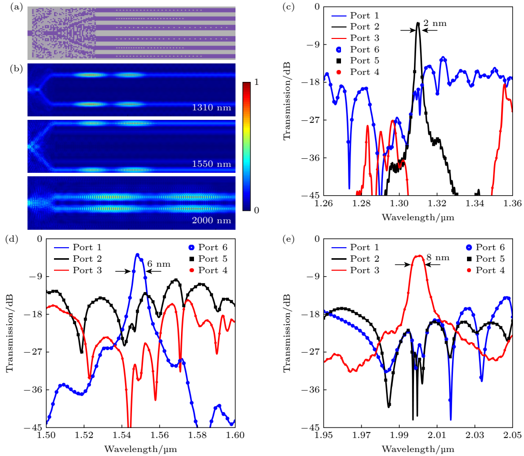
图 8 连接 PHC-BPF 的 3W-PSDM 的仿真结果 (a) 结构示意图; (b) 光场分布; (c)–(e) 透射光谱
