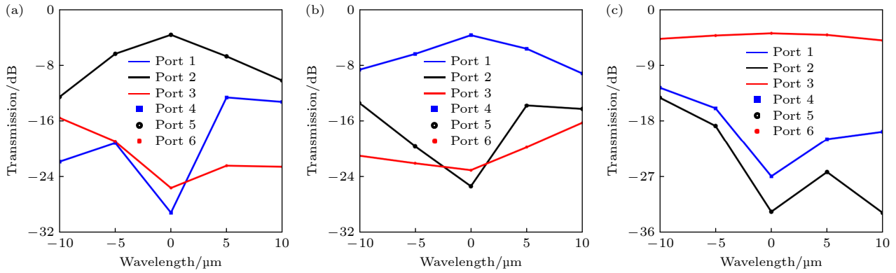
图 9 3W-PSDM 的加工容差分析 (a)–(c) 器件性能随像素单元大小的变化 Fig. 9. 3W-PSDM fabrication tolerances: (a)–(c) Device performance varies with pixel size.
