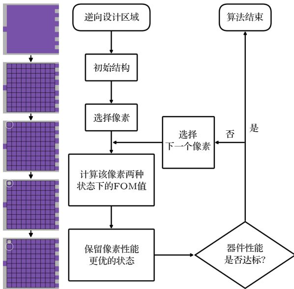
图 2 DBS 算法流程图
