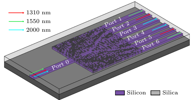
图 3 3W-PSDM 三维结构示意图
