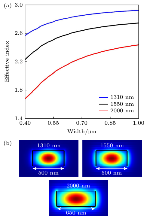
图 4 220 nm 厚的硅波导有效折射率 (a) 波长为 1310, 1550 和 2000 nm 时波导有效折射率; (b) 1310, 1550 和 2000 nm 波长的模场分布
