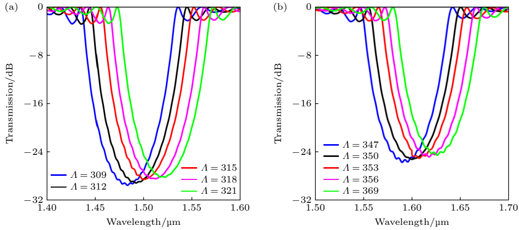
图 6 (a) 1500 nm 带阻 PHC 阵列的透射光谱; (b) 1600 nm 带阻 PHC 阵列的透射光谱
