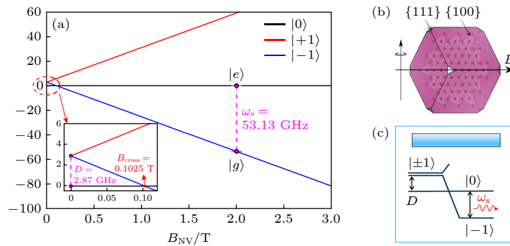
图 2 磁场对 NV 色心基态能级分裂的影响 (a) 基态能级分裂程度随磁场线性变化, 强磁场产生塞曼分裂使得 |-1\rangle 能级低于 |0\rangle 能级, 它们分别被编码为两能级原子的激发态 |e\rangle 和基态 |g\rangle . 图中小图展示较低磁场 (0—0.2 T) 情况下的基态能级分裂情况. (b) 金刚石色心晶向示意图, 静磁场 B 施加方向为 \{111\} 晶向 [17] . (c) 塞曼分裂下的金刚石色心结构图, 基态之外的能级简化为蓝色矩形
