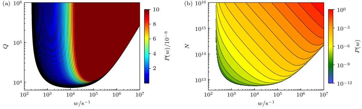
图 6 (a) 给定原子数目 N = 4 \times 10^{13} 时, 受激辐射输出功率随腔品质因素和泵浦速率参数的变化情况; (b) 腔品质因数 Q = 5 \times 10^4 的情况下, 受激辐射输出功率随原子个数 N 和泵浦速率的变化. 这里其他参数取为: \omega_c/2\pi = \omega_s/2\pi = 53.13 GHz, g/2\pi = 0.445 Hz, T_2^* \approx 0.5 \mu s
