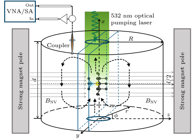
图 3 毫米波受激辐射系统原理图. 一块金刚石 NV 色心样品 (立方体) 被放置在高品质圆柱形 (半径 R , 高为 d ) 谐振腔中 d/2 处, 由 532 \text{ nm} 的光 (绿色曲线箭头所示) 进行激发; 毫米波信号由环形耦合天线导出 (褐色圆柱所示). 腔体两边磁极 (灰色长方体所示) 提供沿 NV 轴向 (即 111 晶向) 的均匀外磁场 B_{\text{NV}} , 该磁场与腔体轴向垂直记为 Z 方向
