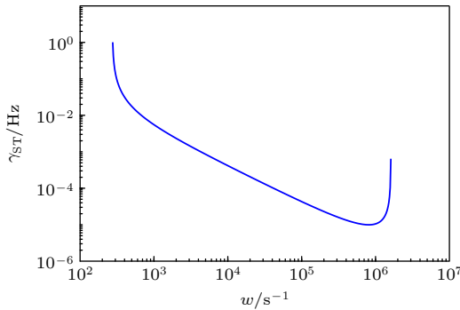
图 7 不同泵浦速率下的受激辐射放大线宽, 这里相关参数取为 Q = 5 \times 10^4 , \omega_c/2\pi = \omega_s/2\pi = 53.13 \text{ GHz} , g/2\pi = 0.445 \text{ Hz} , T_2^* \approx 0.5 \text{ } \mu\text{s} , N = 4 \times 10^{13}
