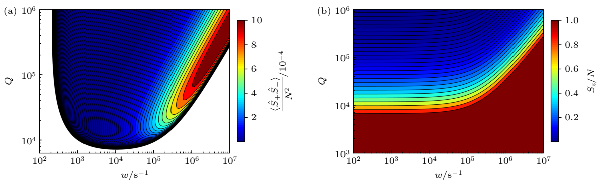
图 5 (a) 当 N = 4 \times 10^{13} 时, 不同泵浦速度下的原子相干性; 黑色线条是腔的阈值. 可见, 产生毫米波受激辐射需要腔的品质因数应大于其阈值. (b) 原子反转布居数 S_z/N 随泵浦速率和腔品质因数变化的行为, 可见在泵浦速率为 \omega_{\max}/2 时反转布居数达到最大 S_z = N/2 . 这里, 腔的品质因数取为 Q = 5 \times 10^4 .
