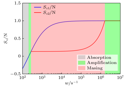
图 4 泵浦速度变化对粒子数反转的影响. 可见, 在低速泵浦时 ( w \sim w_{\text{th}} ) 参与受激辐射的反转数为 S_z/N = \kappa_s \kappa_c / 4g^2 \approx 0.13 . 图中, 由红线和蓝线所围成的区域为可获得受激辐射放大的参数范围. 这里, 其他参数取为: Q = 5 \times 10^4 , \omega_c/2\pi = \omega_s/2\pi = 53.13 \text{ GHz} , g/2\pi = 0.445 \text{ Hz} , T_2^* \approx 0.5 \text{ } \mu\text{s} , N = 4 \times 10^{13} .
