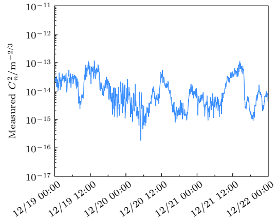
图 6 大气折射率结构常数测量结果
