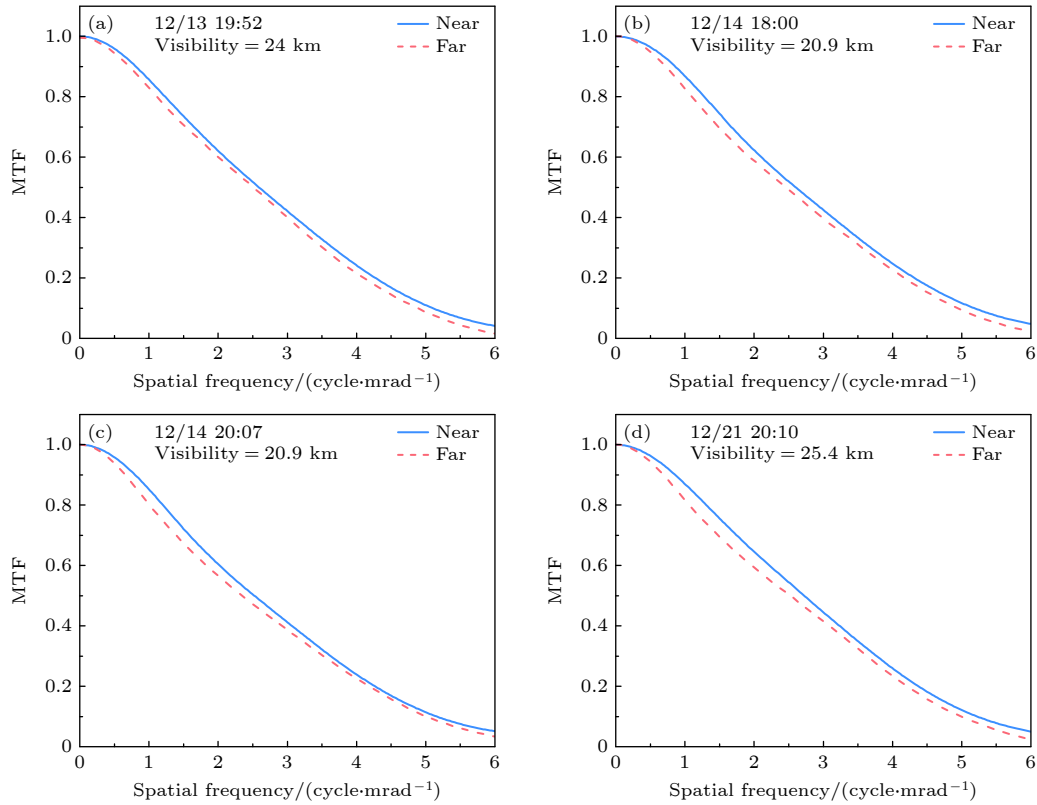
图 9 高能见度条件下, 基于近距离和远距离观测图像得到的 MTF
