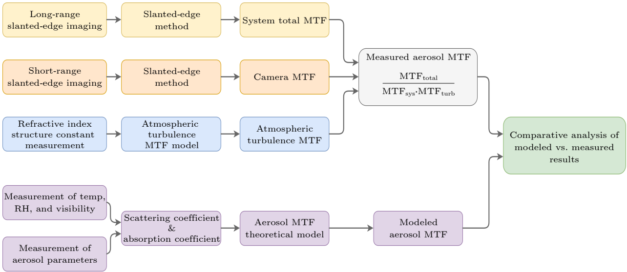
图 2 气溶胶 MTF 建模与测量方案
