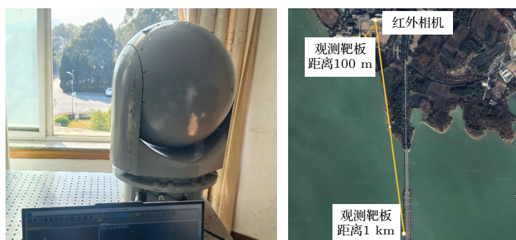
图3 试验场景与观测路径
