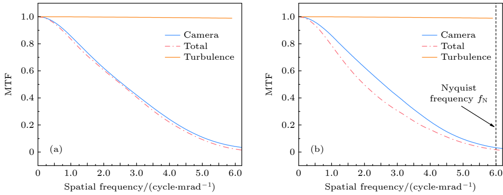
图 8 高能见度 (a) 和低能见度 (b) 条件下观测图像计算的各项 MTF
