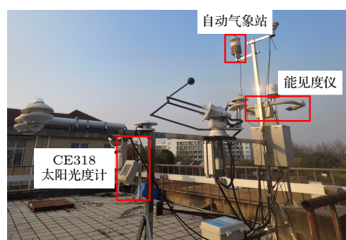
图5 同步气象参数观测设备
