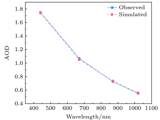
图 12 观测的 AOD 与由推导的气溶胶组成模拟的 AOD
