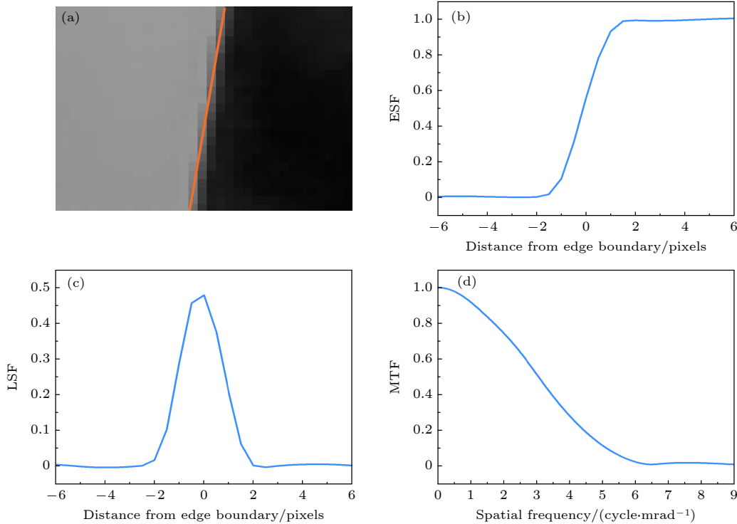
图 7 (a) 刃边区域图像; (b) ESF 计算结果; (c) LSF; (d) MTF
