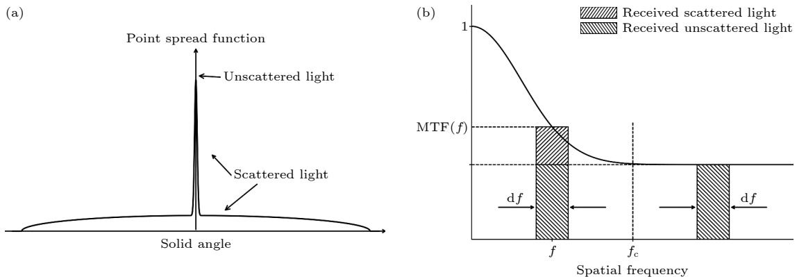
图 1 气溶胶散射对辐射能量分布及空间频率响应的影响机制 (a) 空间域的辐射角分布; (b) 频域的气溶胶调制传递函数衰减特性
