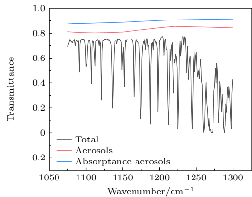
图 10 MODTRAN 计算得到的不同气溶胶相关透过率分量
