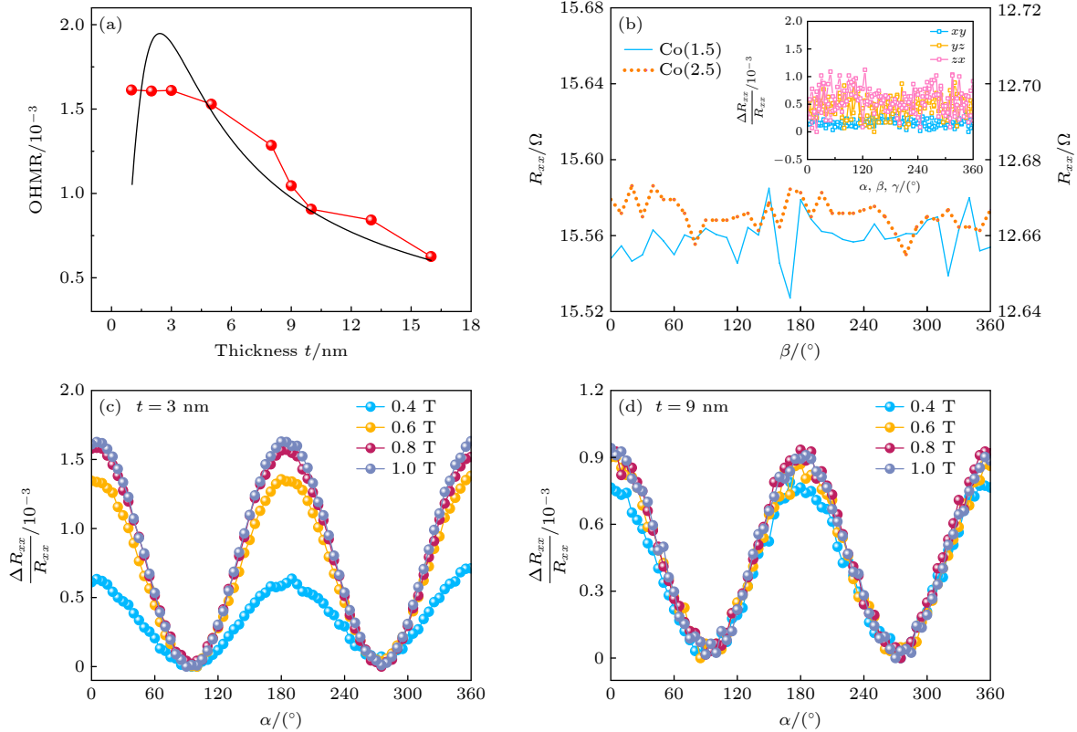
图 3 (a) \text{Cr}(t)/[\text{Co}/\text{Pt}]_3 样品中 OHMR 随 Cr 厚度的变化关系, 黑线为拟合曲线; (b) \text{Cr}/\text{Co}(1.5, 2.5)/\text{Cr} 霍尔巴结构的室温 R_{xx} 随扫描角 \gamma 的变化曲线, 插图为 5 nm 厚度单层 Cr 薄膜的磁电阻曲线; (c), (d) \text{Cr}(t)/[\text{Co}/\text{Pt}]_3 ( t = 3, 9 nm) 样品中 MR 随外磁场的变化
