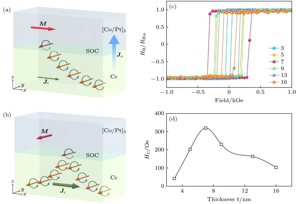
图 1 (a), (b) Cr( t )/[Co/Pt] 3 多层膜中 OHMR 物理机制示意图, 其中电荷流 J_c 沿 +x 轴方向施加; 该电荷流通过 OHE 在体系中产生一个沿 -y 轴极化 (橙色箭头) 的轨道流 J_o , 沿 +z 轴方向注入铁磁层; 当 [Co/Pt] 3 中磁矩 M (红色箭头) 与轨道流极化方向垂直 (a) 时体系为高电阻态, 与轨道流极化方向平行 (b) 时为低电阻态; (c), (d) Cr( t )/[Co/Pt] 3 多层膜的室温归一化反常霍尔曲线 (c) 和矫顽力随 Cr 厚度变化关系 (d)
