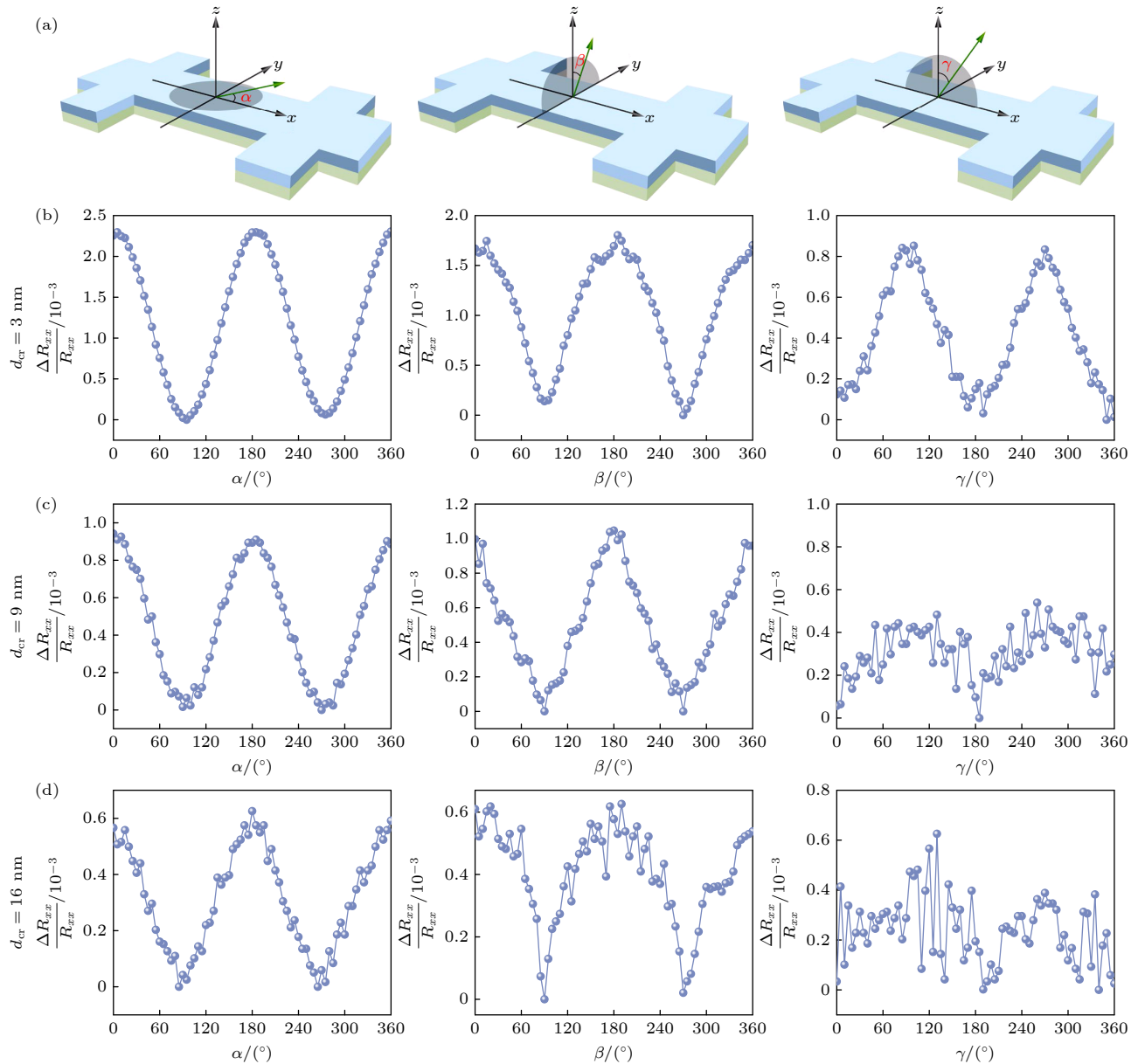
图 2 (a) 样品霍尔巴结构以及在 xy , yz 和 xz 平面内磁电输运测量示意图; (b)–(d) 不同 Cr 厚 \text{Cr}(t)/[\text{Co}/\text{Pt}]_3 ( t = 3, 9, 16 ) 多层膜中 \Delta R_{xx}/R_{xx} 随 \alpha , \beta 和 \gamma 扫描角的变化关系; 测试外磁场为 10 kOe, 测试温度为室温
