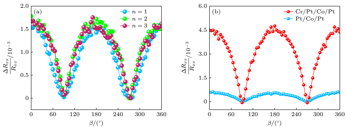
图 4 (a) [\text{Cr}(2)/[\text{Co}/\text{Pt}]_3]_n ( n = 1, 2, 3 ) 样品的室温 OHMR; (b) Pt/Co/Pt 和 Cr/Pt/Co/Pt 样品的室温 MR 曲线
