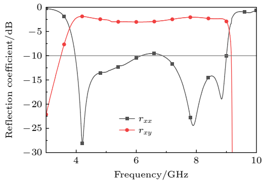
图 6 交叉极化与同极化反射系数曲线
