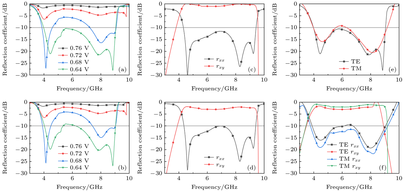
图 14 (a), (b) 不同偏置电压下 (a) TE 极化和 (b) TM 极化的反射系数; (c) TE 极化和 (d) TM 极化下的最佳交叉极化与同极化反射系数; (e) 60°入射时, TE, TM 极化下最佳反射系数; (f) 60°入射时, TE, TM 极化下最佳交叉极化与同极化反射系数
