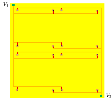
图 2 底部 2 \times 2 时的馈线分布
