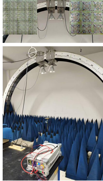
图 13 样件实物及实验测试平台
