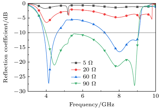
图 3 PIN 二极管在不同等效阻抗下超表面的反射系数曲线 Fig. 3. Reflection curves of metasurface with PIN diodes under different equivalent impedances.
