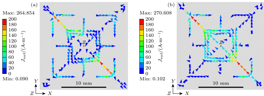
图 8 超表面的表面电流分布 (a) f_1 = 4.25 \text{ GHz} ; (b) f_2 = 8.25 \text{ GHz}
