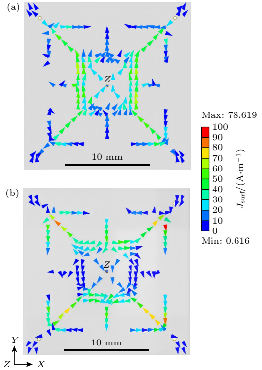
图 4 超表面的表面电流分布 (a) f_1 = 4.25 GHz; (b) f_2 = 8.25 GHz
