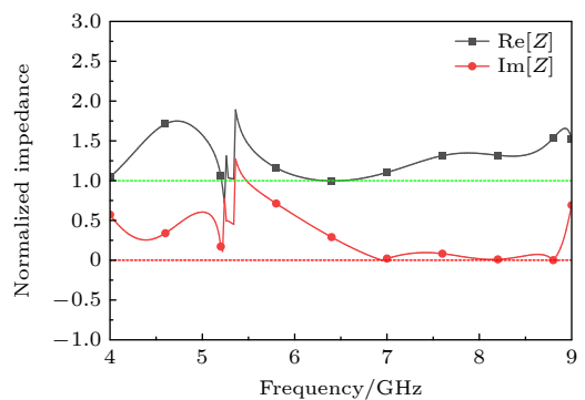
图 10 超表面的归一化阻抗 Fig. 10. Normalized impedance of metasurface.
