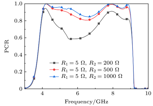
图 7 极化转换率曲线
