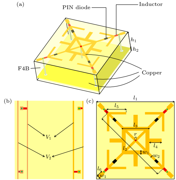
图 1 单元结构设计 (a) 三维结构; (b) 底部馈电层; (c) 俯视图
