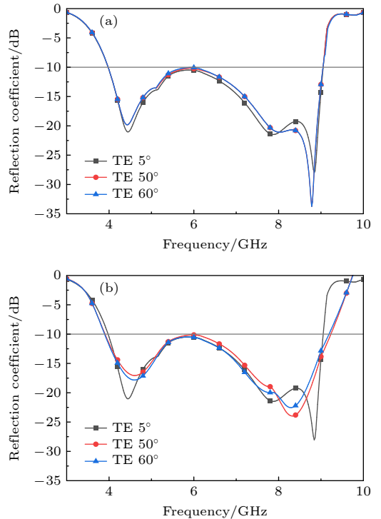
图 5 大入射角时超表面的反射系数 (a) TE 极化; (b) TM 极化
