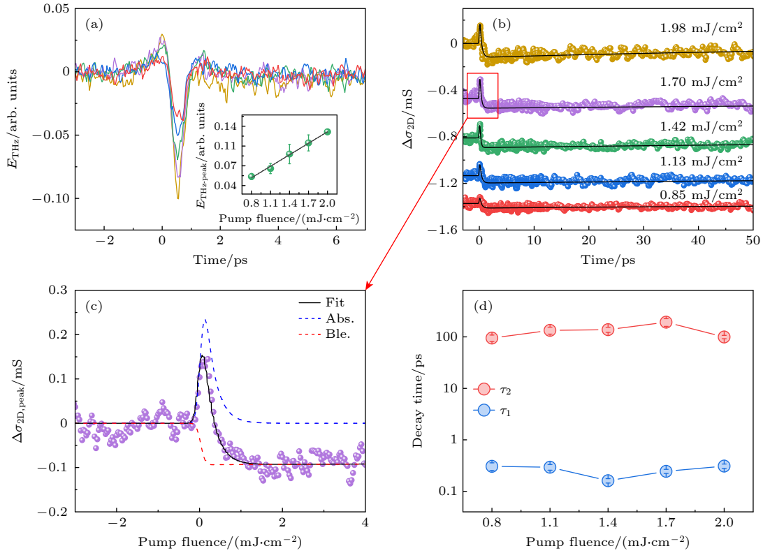
图 4 (a) 20 nm Co 2 MnAl 薄膜在不同泵浦光脉冲能量密度下的太赫兹辐射信号, 插图太赫兹信号峰-峰值幅值与泵浦脉冲能量密度的依赖关系; (b) 不同入射泵浦光脉冲能量密度下 Co 2 MnAl 薄膜面电导率 \Delta\sigma_{2D} 的动力学; (c) 短时间窗口内 Co 2 MnAl 薄膜在 1.70 mJ/cm 2 激光能量密度下的瞬态面电导率 \Delta\sigma_{2D} , 蓝色和红色虚线分别代表着正电导率分量 (光诱导吸收) 和负电导率 (光诱导漂白) 分量; (d) 弛豫时间常数随泵浦脉冲能量密度的依赖关系
