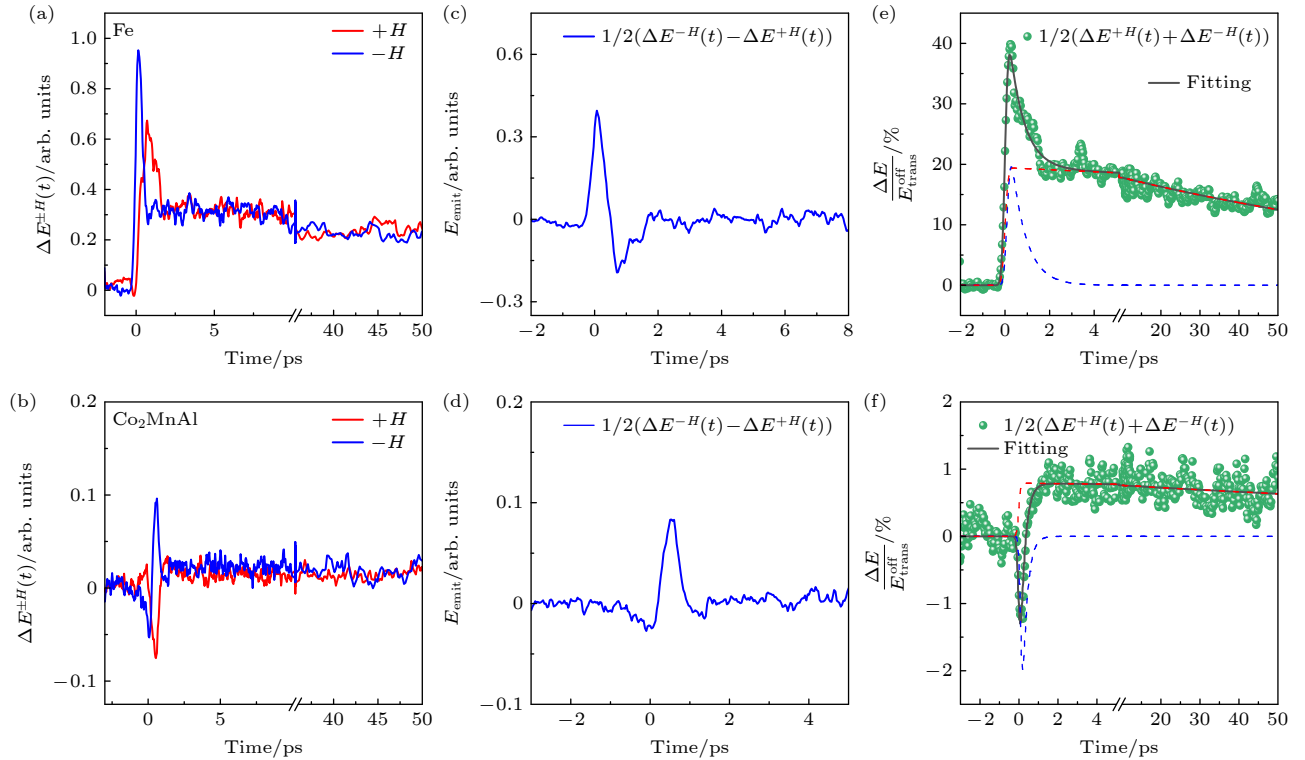
图 2 \pm H 磁场条件下测得 (a) 12 nm 的 Fe 薄膜和 (b) 20 nm 的 \text{Co}_2\text{MnAl} 薄膜的 OPTP 曲线 \Delta E^{\pm H}(t) , 泵浦激光能量密度为 1.70 \text{ mJ/cm}^2 ; 基于 (2) 式得到 (c) Fe 薄膜和 (d) \text{Co}_2\text{MnAl} 薄膜在外磁场条件下的太赫兹辐射信号 E_{\text{emit}}(t) ; 基于 (3) 式得到 (e) Fe 薄膜和 (f) \text{Co}_2\text{MnAl} 薄膜在泵浦光诱导下时间分辨太赫兹透射信号变化量 \Delta E(t)/E_{\text{trans}}^{\text{off}}
