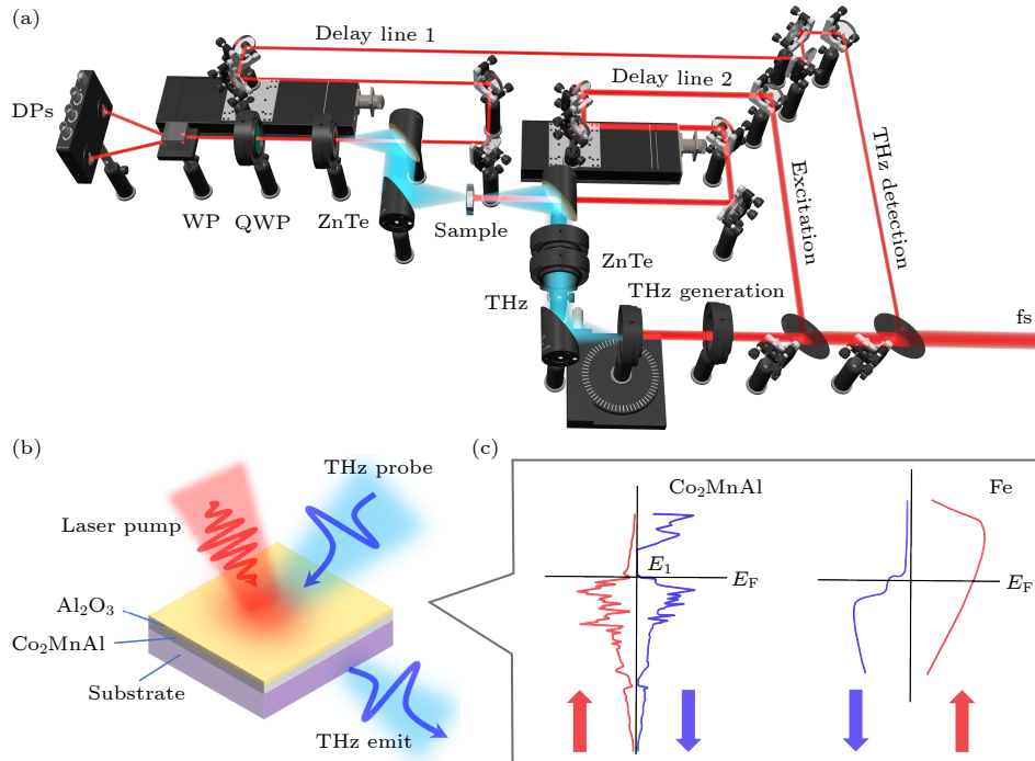
图 1 (a) 光泵浦-太赫兹探测光谱系统示意图; (b) \text{Co}_2\text{MnAl} 薄膜中太赫兹探测和太赫兹发射示意图; (c) \text{Co}_2\text{MnAl} 和 Fe 薄膜的能带结构示意图
