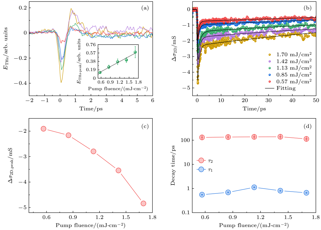
图 3 (a) 12 nm 的 Fe 薄膜在不同泵浦光脉冲能量密度下的太赫兹辐射信号, 插图为太赫兹信号峰-峰值与泵浦脉冲能量密度的依赖关系; (b) 不同入射泵浦光脉冲能量密度下 Fe 薄膜面电导率 \Delta\sigma_{2D} 的动力学; (c) \Delta\sigma_{2D} 的峰值电导率随脉冲能量密度的变化关系; (d) 弛豫过程时间常数随泵浦脉冲能量密度的依赖关系
