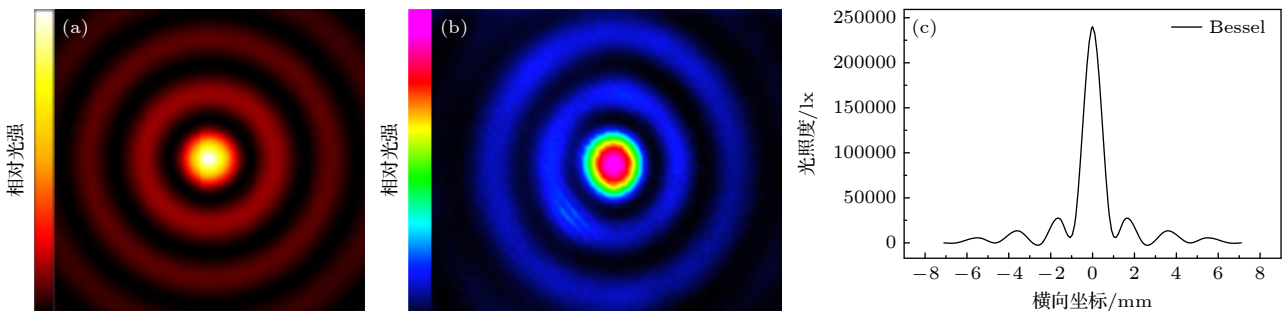
图 7 理想 Bessel 光场分布与实验实测结果对比 (a) 理想 Bessel 光束二维光强分布; (b) 本实验利用毛细管制备 Bessel 光束二维光强分布; (c) 本实验利用毛细管制备 Bessel 光束的一维光强分布曲线
