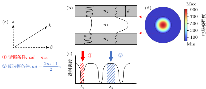
图 2 反谐振反射光波导示意图 [27–29] (a) 波导相关理论条件; (b) 反谐振反射光波导结构; (c) 其支持的传输谱; (d) 对应电场模强度分布
