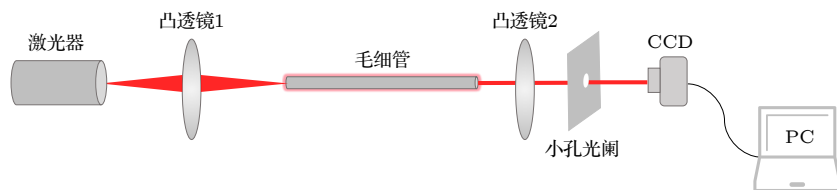
图 5 基于毛细管调制 Bessel 光束实验装置图
