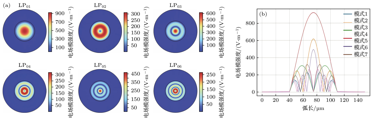
图 3 Comsol 模式分析图 (a) 模场仿真图; (b) 毛细管中不同模式间干涉分析图
