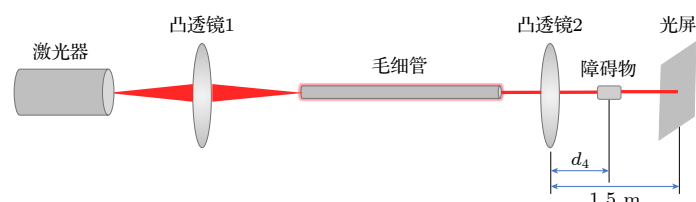
图 12 Bessel 光束自修复特性验证实验光路示意图
