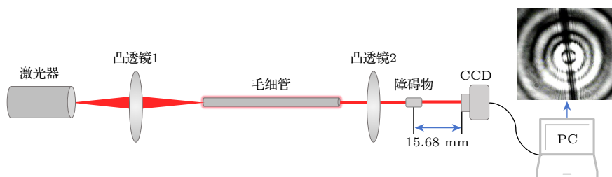
图 11 Bessel 光束断裂光斑近场观测实验示意图
