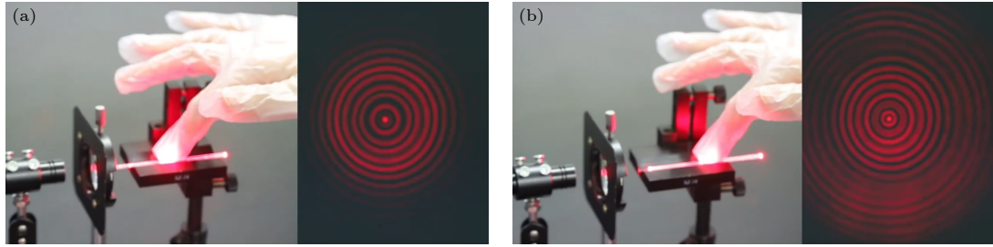
图 9 环数变化图 (a) 毛细管移动前; (b) 毛细管向后移动
