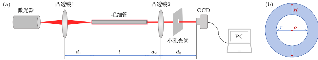
图 8 装置参数图 (a) 毛细管产生 Bessel 光装置各参数示意图; (b) 毛细管横截面图
