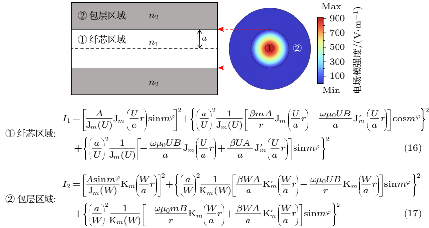
图 4 光纤横截面电场模强度空间分布仿真与理论模型对照
