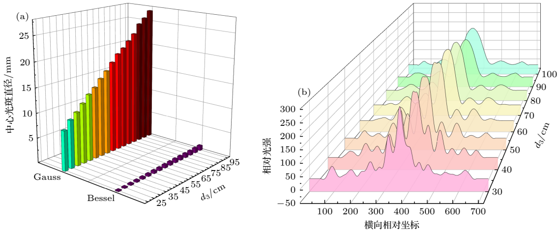
图 10 毛细管生成 Bessel 光束无衍射性展示 (a) Gauss 光束与 Bessel 光束随距离发散对比; (b) Bessel 光束横向光强分布随传输距离演化
