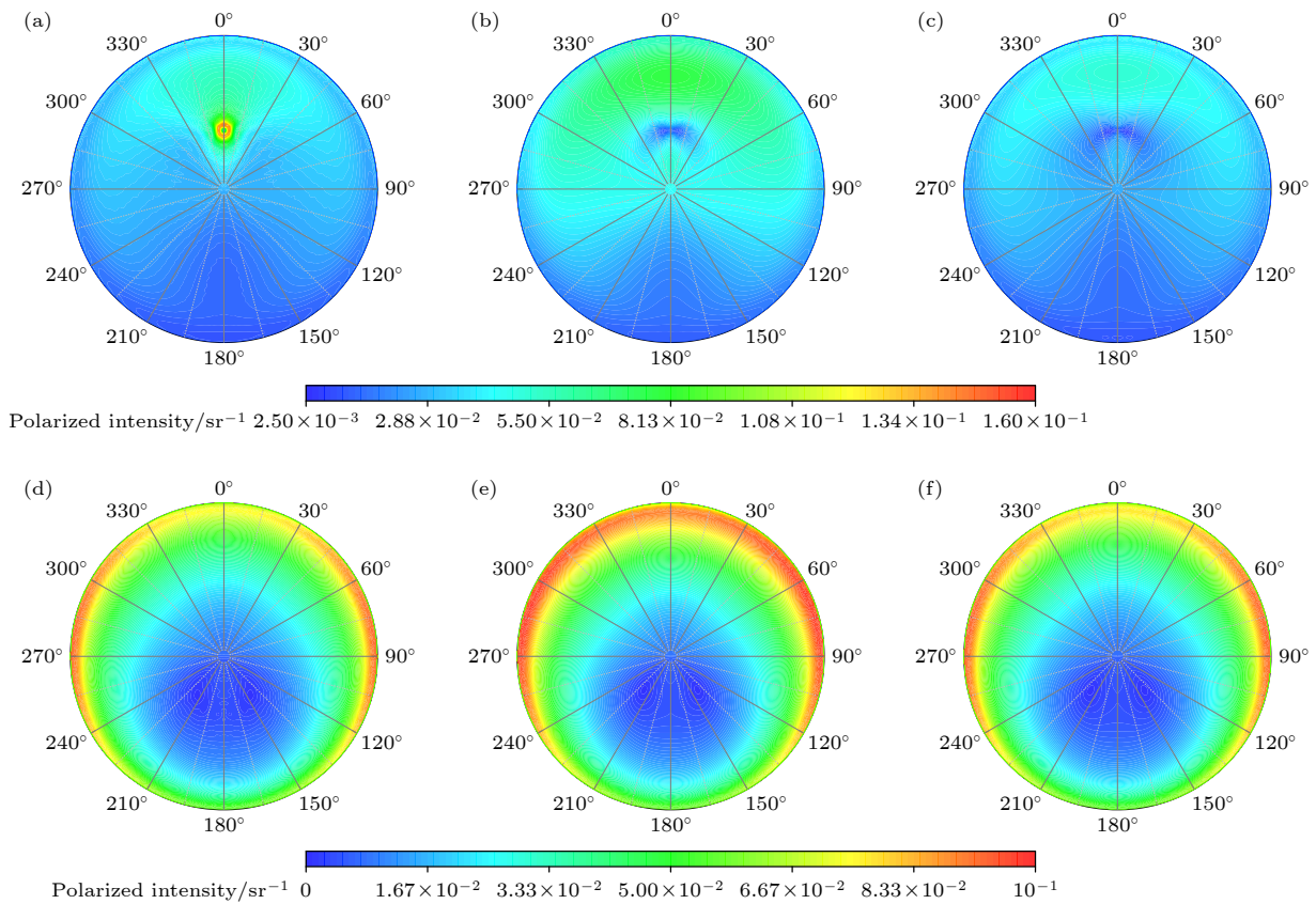
图 10 0.532\ \mu\text{m} 波长下不同形状模型对应的沙尘气溶胶线偏振度全天空分布 (a)–(c) 依次为大气底层球形、旋转椭球体及三轴椭球体模型结果; (d)–(f) 依次为大气顶层对应模型结果
