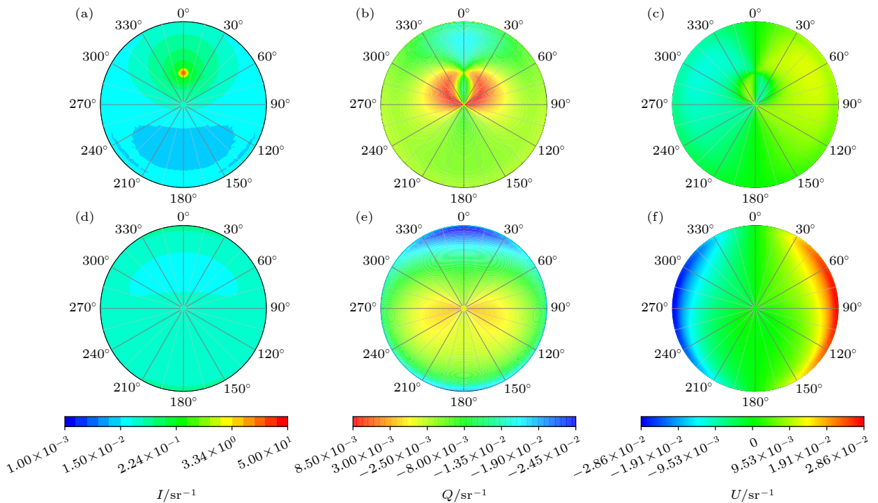
图6 0.532 \mu\text{m} 波长下模拟的三轴椭球形沙尘气溶胶大气漫射辐射斯托克斯参量的角分布 (a)–(c) 地表下行辐射场; (d)–(f) 大气层顶上行辐射场. 所有子图均展示了辐射量随相对方位角与观测天顶角的变化
