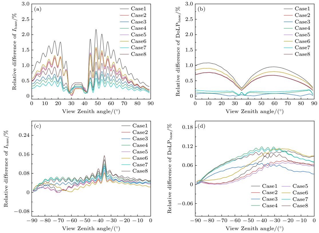
图 14 532 \mu\text{m} 波段沙尘气溶胶统计参数的敏感性分析 (a), (b) 分别为沙漠地表下行辐射强度与线偏振度相对基准值的变化百分比; (c), (d) 分别为大气层顶上行辐射强度与线偏振度相对基准值的变化百分比
