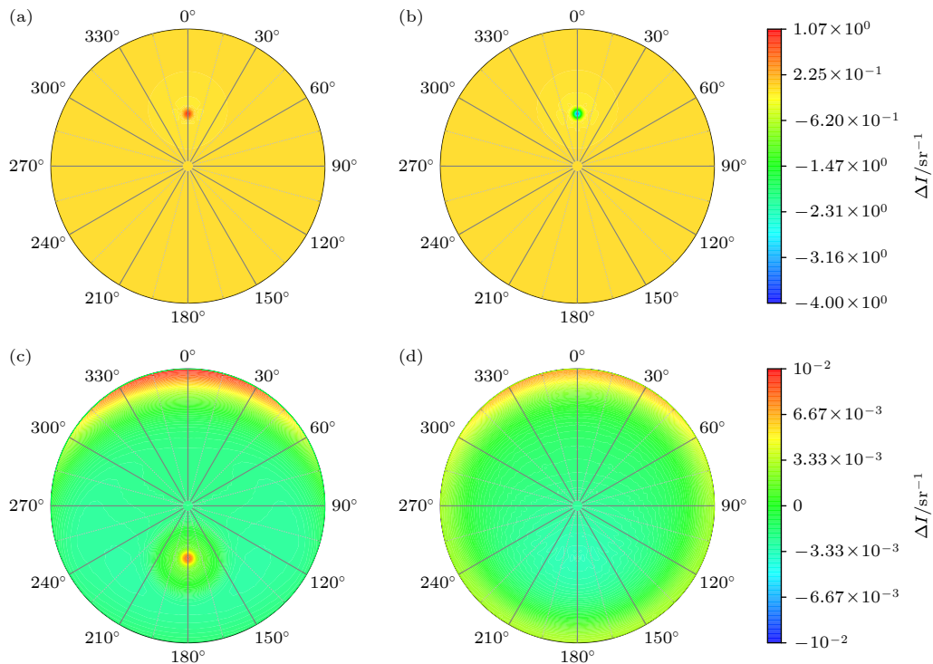
图 7 1.55 \mu\text{m} 波长下三轴椭球体沙尘气溶胶光谱辐射率 I 相对不同参考形状的相对偏差 (a) 大气层顶相对于球形模型; (b) 大气层顶相对于旋转椭球体模型; (c) 大气层底相对于球形模型; (d) 大气层底相对于旋转椭球体模型
