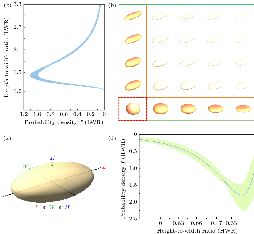
图 2 不同形状分布参数下的形态示意图 (a) 三轴椭球体三个特征轴的定义; (b) 红色虚线框包围的区域表示球形模型; 橙色实线框包围的区域对应旋转椭球体模型; 绿色实线框包围的区域对应本研究所采用的三轴椭球体模型; (c), (d) 蓝色阴影区域与绿色阴影区域分别表征 LWR 与 HWR 的概率密度分布曲线
