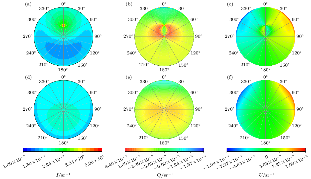
图5 1.55 \mu\text{m} 波长下模拟的三轴椭球形沙尘气溶胶大气漫射辐射斯托克斯参量的角分布 (a)–(c) 地表下行辐射场; (d)–(f) 大气层顶上行辐射场. 所有子图均展示了辐射量随相对方位角与观测天顶角的变化
