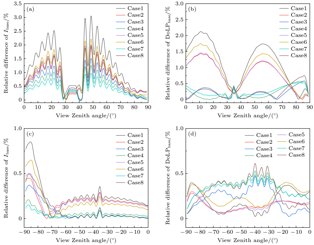
图 13 1.550 \mu\text{m} 波段沙尘气溶胶统计参数的敏感性分析 (a), (b) 分别为沙漠地表下行辐射强度与线偏振度相对基准值的变化百分比; (c), (d) 分别为大气层顶上行辐射强度与线偏振度相对基准值的变化百分比
