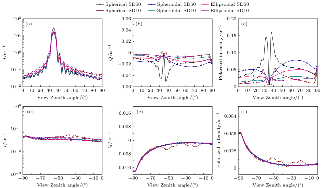
图 12 0.532\ \mu\text{m} 波长下, 考虑 SD10 与 SD50 两种粒径分布, 球形、旋转椭球体及三轴椭球体沙尘粒子的辐射场斯托克斯分量 I , Q 与线偏振度分布 (a)–(c) 沙漠地表下行辐射; (d)–(f) 大气层顶上行辐射
