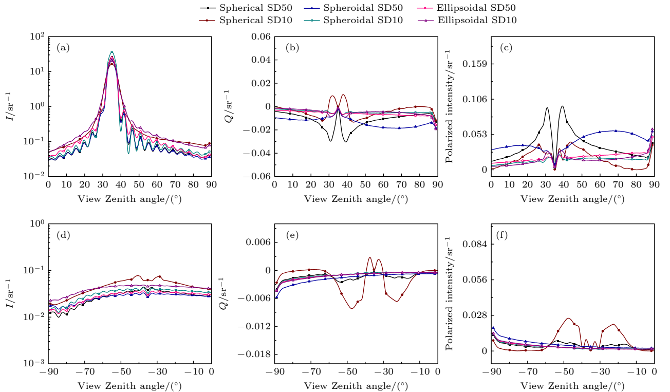
图 11 1.55\ \mu\text{m} 波长下, 考虑 SD10 与 SD50 两种粒径分布, 球形、旋转椭球体及三轴椭球体沙尘粒子的辐射场斯托克斯分量 I 、 Q 与线偏振度分布 (a)—(c) 沙漠地表下行辐射; (d)—(f) 大气层顶上行辐射
