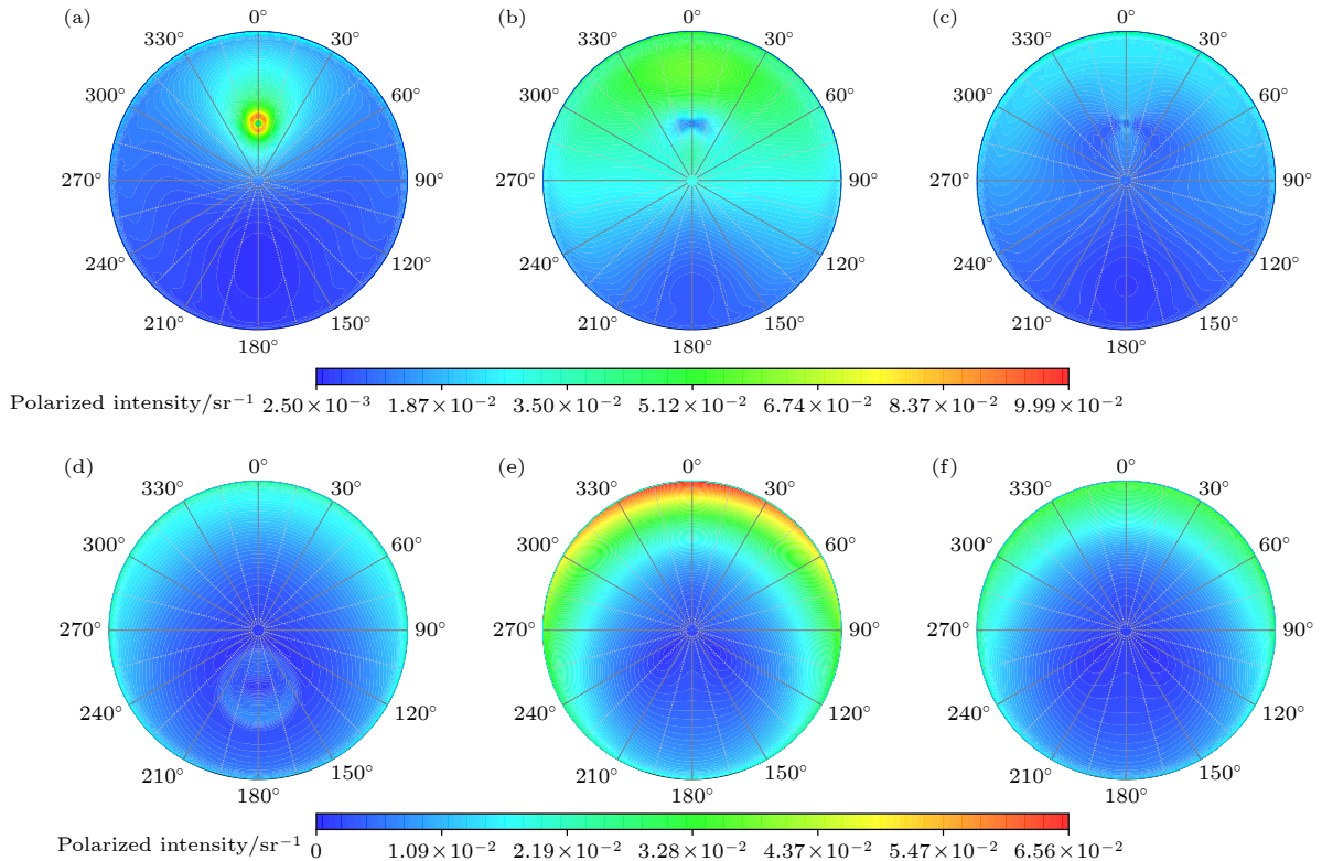
图 9 1.55\ \mu\text{m} 波长下不同形状模型对应的沙尘气溶胶线偏振度全天空分布 (a)–(c) 依次为大气底层球形、旋转椭球体及三轴椭球体模型结果; (d)–(f) 依次为大气顶层对应模型结果
