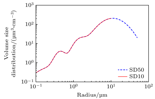
图 1 Fennec 实验期间观测到的沙尘颗粒体积粒径分布平均对数拟合曲线. 其中, 最大半径可达 50\text{ }\mu\text{m} 的“SD50”体积粒径分布以蓝色呈现, 最大半径可达 10\text{ }\mu\text{m} 的“SD10”体积粒径分布以红色呈现
