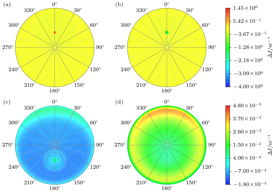
图 8 0.532\ \mu\text{m} 波长下三轴椭球体沙尘气溶胶光谱辐射率 I 相对不同参考形状的相对偏差 (a) 大气层顶相对于球形模型; (b) 大气层顶相对于旋转椭球体模型; (c) 大气层底相对于球形模型; (d) 大气层底相对于旋转椭球体模型
