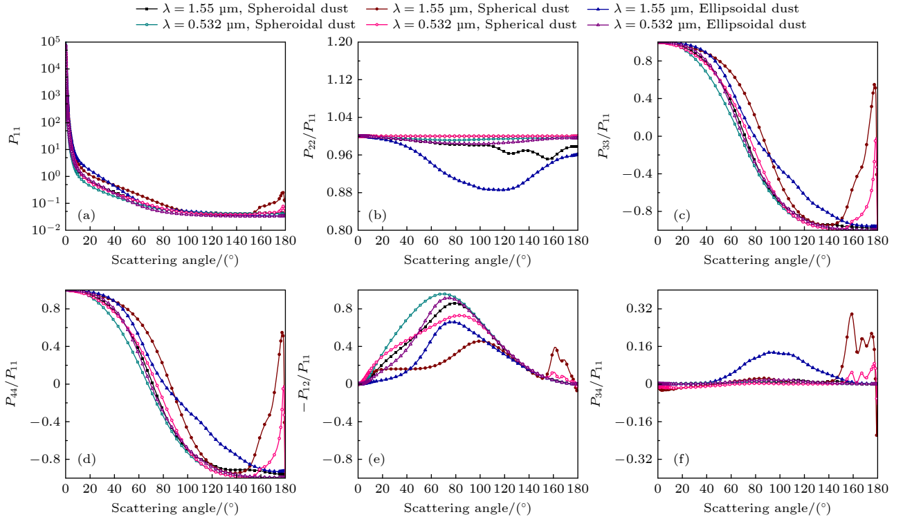
图 4 1.55 μm 和 0.532 μm 波长下球体、旋转椭球体与三轴椭球体模型的散射相矩阵元素对比
