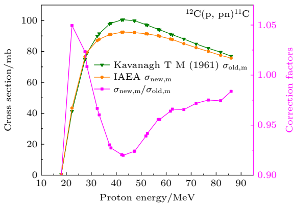
图 3 Kavanagh 和 Bell (1961) [14] 使用的 ^{12}\text{C}(\text{p}, \text{pn})^{11}\text{C} 监测截面修正因子
