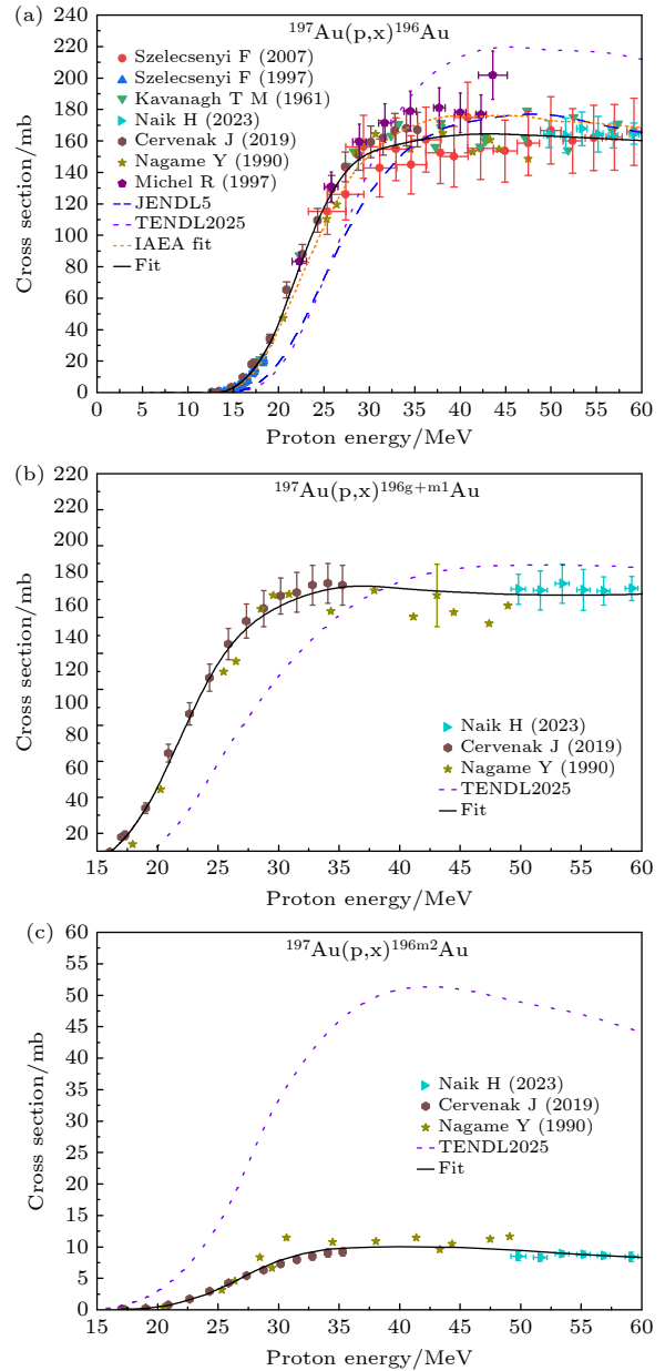
图 5 ^{197}\text{Au}(\text{p}, \text{x})^{196}\text{Au} 反应截面经修正与筛选后的实验截面数据、评价库数据及本工作评价推荐值汇总 (a)–(c) 分别为 ^{197}\text{Au}(\text{p}, \text{x})^{196}\text{Au} , ^{197}\text{Au}(\text{p}, \text{x})^{196(\text{g}+\text{m}1)\text{Au}} 和 ^{197}\text{Au}(\text{p}, \text{x})^{196\text{m}2}\text{Au} 反应道
