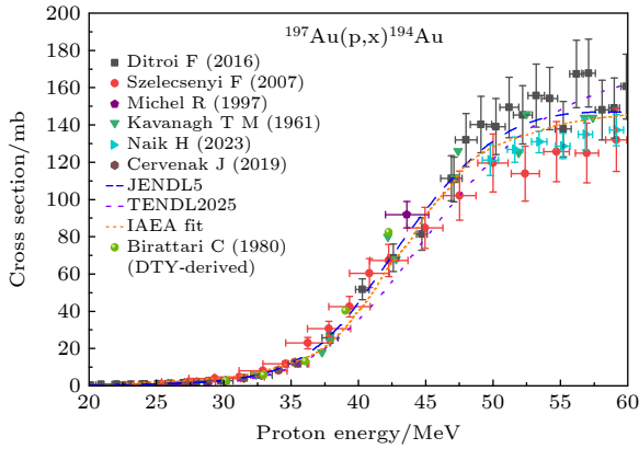
图 6 ^{197}\text{Au}(\text{p}, \text{x})^{194}\text{Au} 反应截面实验数据、评价库数据及微分厚靶产额反算截面汇总
