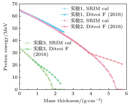
图 4 Ditroi et al. (2016) [8] 三组叠层靶中质子降能曲线的 SRIM 计算结果
