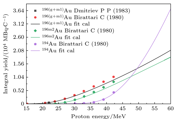
图 8 ^{197}\text{Au}(\text{p}, \text{x})^{196(\text{g+m1})}\text{Au} , ^{196\text{m2}}\text{Au} 和 ^{194}\text{Au} 厚靶产额的计算值与实验测量值对比
