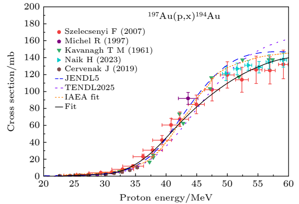
图 7 ^{197}\text{Au}(\text{p}, \text{x})^{194}\text{Au} 反应截面经修正与筛选后的实验截面数据、评价库数据及本工作评价推荐值汇总
