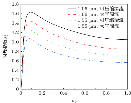
图 5 不同波长修正可压缩湍流谱与传统大气湍流基准谱计算得到的高斯光束闪烁指数比较
