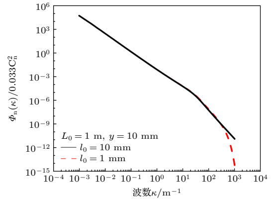
图 2 不同内尺度下的修正可压缩湍流谱
