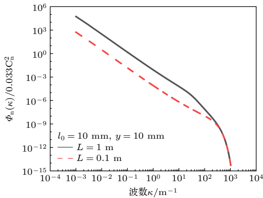
图 1 不同外尺度下的修正可压缩湍流谱
