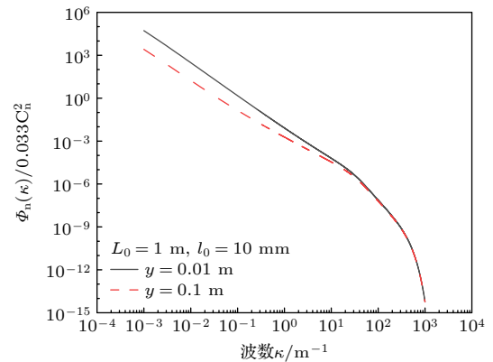
图 3 不同壁面距离下的修正可压缩湍流谱
