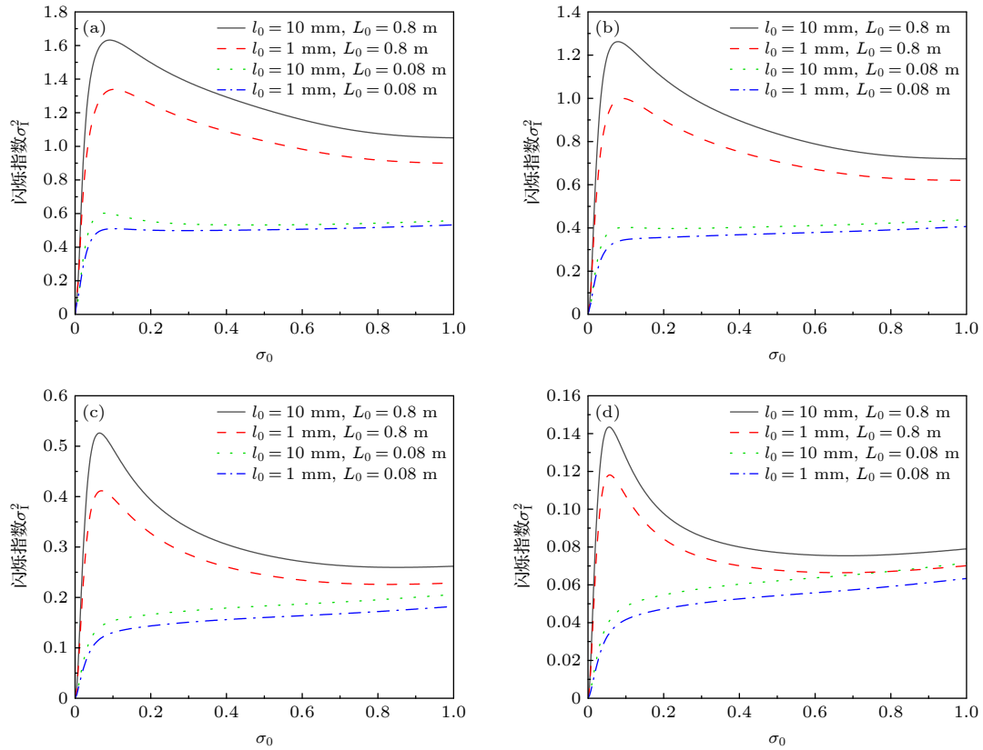
图 4 考虑内、外尺度时不同波长下的激光波束的闪烁指数 (a) \lambda = 1.06 \mu\text{m} ; (b) \lambda = 1.55 \mu\text{m} ; (c) \lambda = 3.8 \mu\text{m} ; (d) \lambda = 10.6 \mu\text{m}
