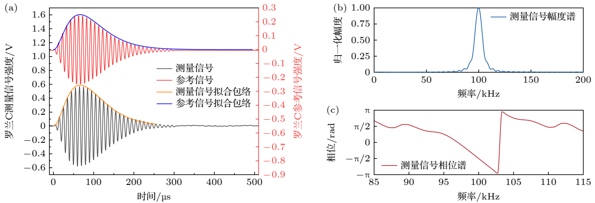
图 3 里德伯罗兰-C 信号的时域与频域分析
