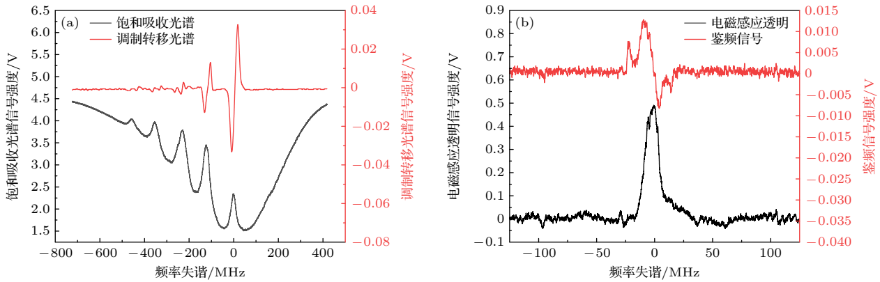
图 2 MTS-EIT 光谱信号及鉴频信号
