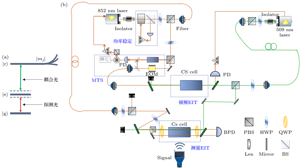
图 1 系统装置及能级图
