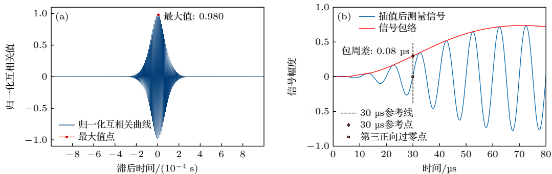
图4 里德伯信号的保真度与包周差
