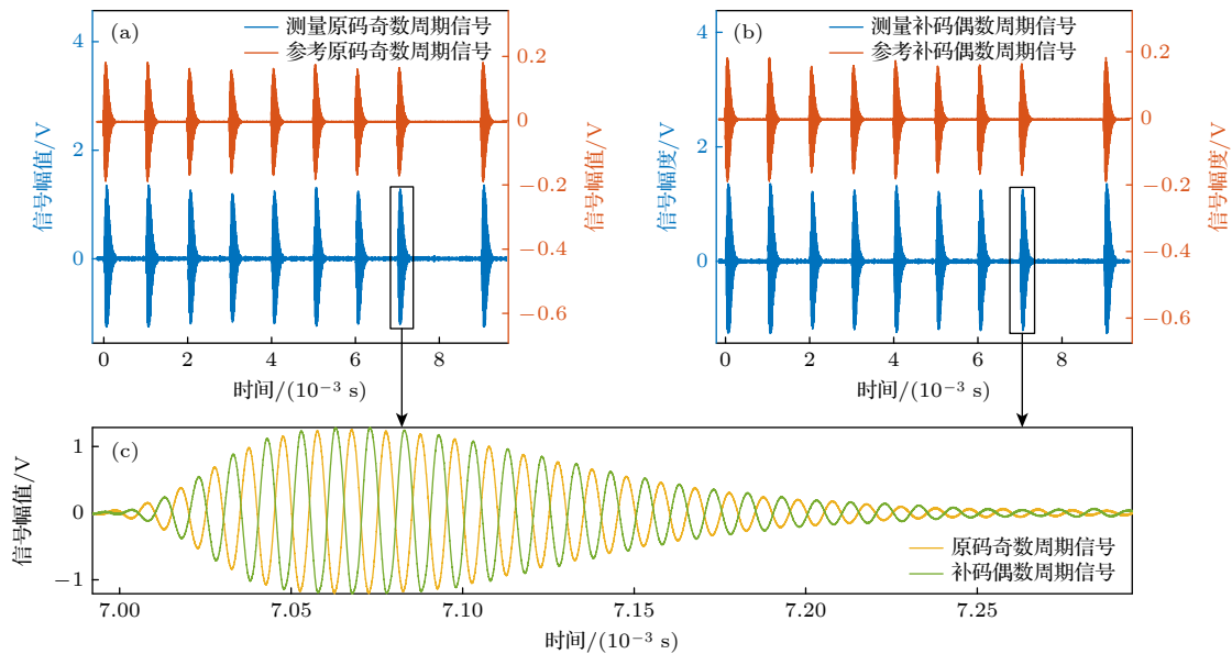
图5 原码奇数周期与补码偶数周期时域信号对比
