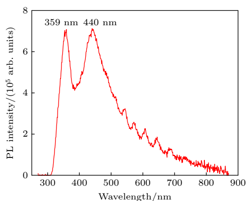
图 2 NaCl:Cu 样品在 250 nm 激发下的 PL 发射光谱
