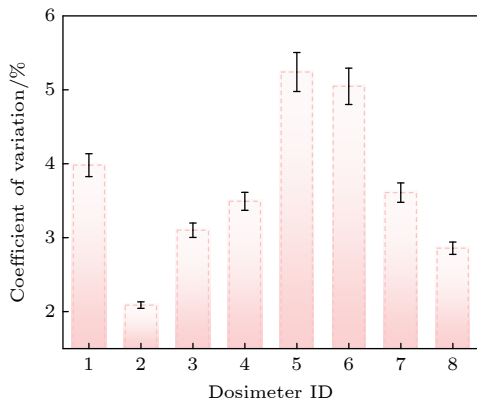
图 4 NaCl:Cu 元件重复测读过程中的变异系数
