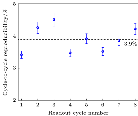
图 5 NaCl:Cu 元件在多次循环读出次数下的批内一致性
