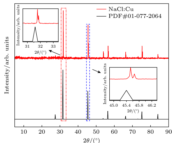
图 1 Cu 离子注入制备的 NaCl:Cu 的 XRD 图
