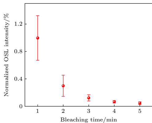
图 3 NaCl:Cu 样品的光漂白特性
