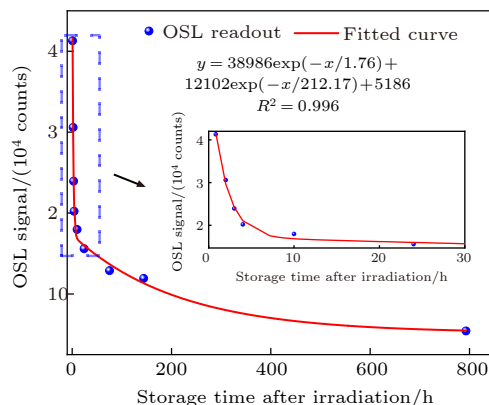
图 7 NaCl:Cu 样品光释光信号储存衰减曲线及双指数拟合结果
