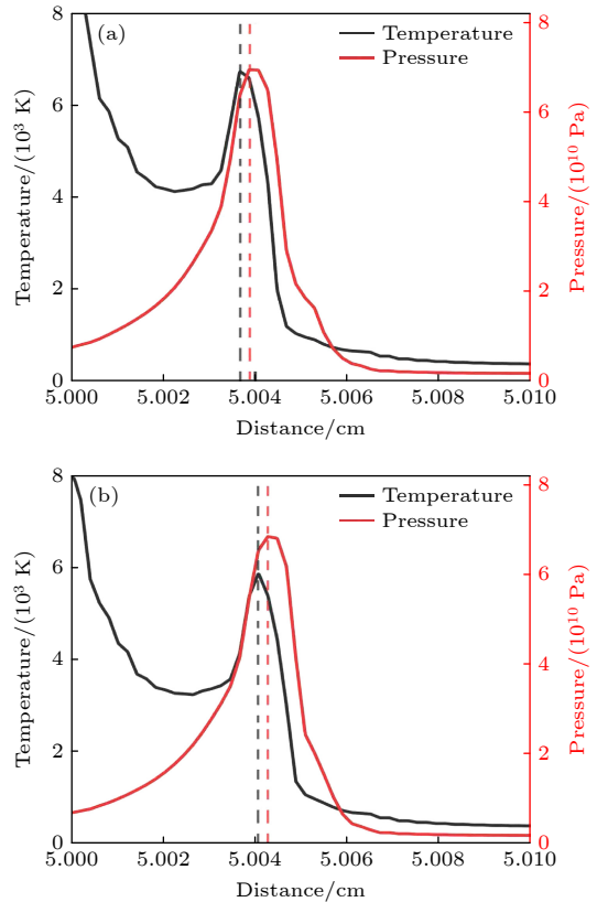
图5 第二阶段温度压力图像(黑线为物质离子温度,红线为物质压强,由辐射预热温度与冲击波共同影响出现了明显的物质温度峰与压强峰错位现象)(a) 4.4 ns 温度与压力图像;(b) 4.8 ns 温度与压力图像
