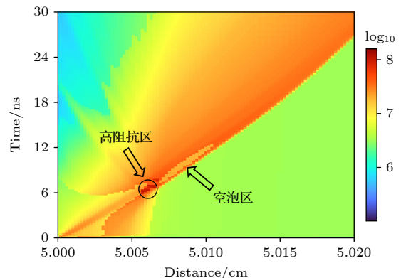
图6 阻抗随时间和位移的分布图像,图中由蓝到红为阻抗从低至高,出现了明显的高阻抗区域与阻抗“空泡区”
