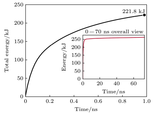
图 2 辐射源的辐射能量随时间演化图像. 主图为初始 1 ns 内的能量曲线, 1 ns 时总能量达到 221.8 kJ, 占总能量的 85%, 突显了该阶段能量的快速增长, 放大图为总的能量曲线
