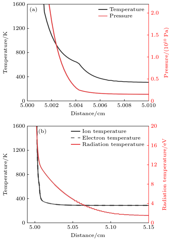
图 3 第一阶段靶受辐照区域物性图像 (a) 0.2 ns 靶物质温度压力图像, 黑线为靶物质离子温度随位移的变化, 红线为靶物质压力随位移的变化; (b) 0.2 ns 靶物质三温图像, 黑线为离子温度与电子温度, 红线为辐射温度, 离子温度与电子温度基本一致
