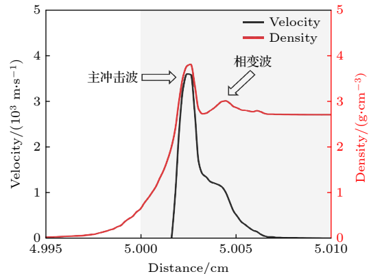
图 4 第 2 阶段初期波系分布. 灰色阴影区域为靶目标, 在 X 射线辐射后形成主冲击波与相变波两个峰; 主冲击波是由于软 X 射线沉积表面反冲动量产生, 相变波则源于辐射预热能量向前传播的热压缩波; 由于固液相变发生在预热区, 改变了材料的声阻抗, 进而影响相变波与主冲击波之间的分离
