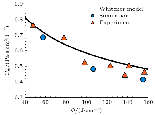
图 9 软 X 射线冲量耦合系数对比图, 蓝色圆点为本文模拟结果, 红色三角形为林鹏等 [9] 实验结果, 黑色曲线为 Whitener 模型结果
