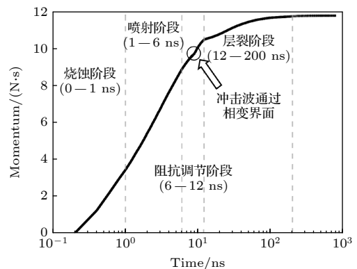
图 8 动量随时间演化图像, 在动量增长过程中第 2 阶段为主要贡献, 圈出区域表明第 3 阶段出现相变界面影响动量增长速度
