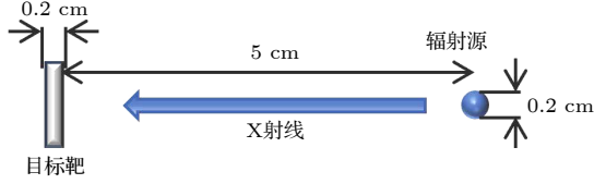
图 1 辐射流体程序模拟示意图. 辐射源中心到目标靶距离为 5 cm; 辐射源离子温度与电子温度为 19 MK、辐射温度为 300 K, 辐射过程自行演化; 目标靶三温温度均为 300 K
