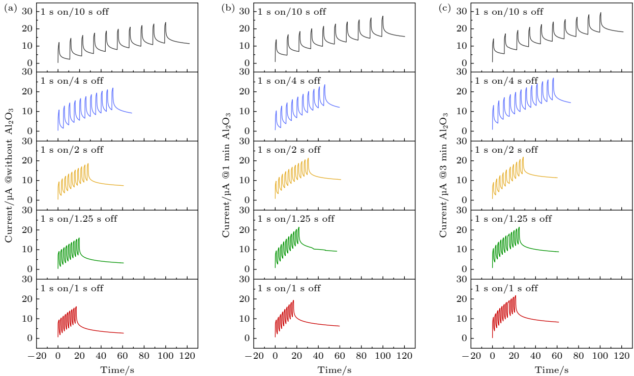
图 7 \text{CuO}/\text{Al}_2\text{O}_3/\text{ZnO} 器件在不同脉冲周期条件下的 I - T 曲线 (测试中光功率密度均为 360 \mu\text{W}/\text{cm}^2 , 单个脉冲宽度均为 1 s, 脉冲个数为 10) (a) 关光时长 0 min \text{Al}_2\text{O}_3 ; (b) 关光时长 1 min \text{Al}_2\text{O}_3 ; (c) 关光时长 3 min \text{Al}_2\text{O}_3
