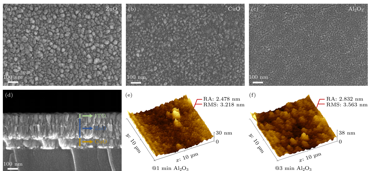
图 2 (a) ZnO 薄膜表面, (b) CuO 薄膜表面, (c) \text{Al}_2\text{O}_3 薄膜表面和 (d) 器件横截面的 SEM 形貌; 沉积 (e) 1 min 和 (f) 3 min \text{Al}_2\text{O}_3 薄膜的 AFM 形貌
