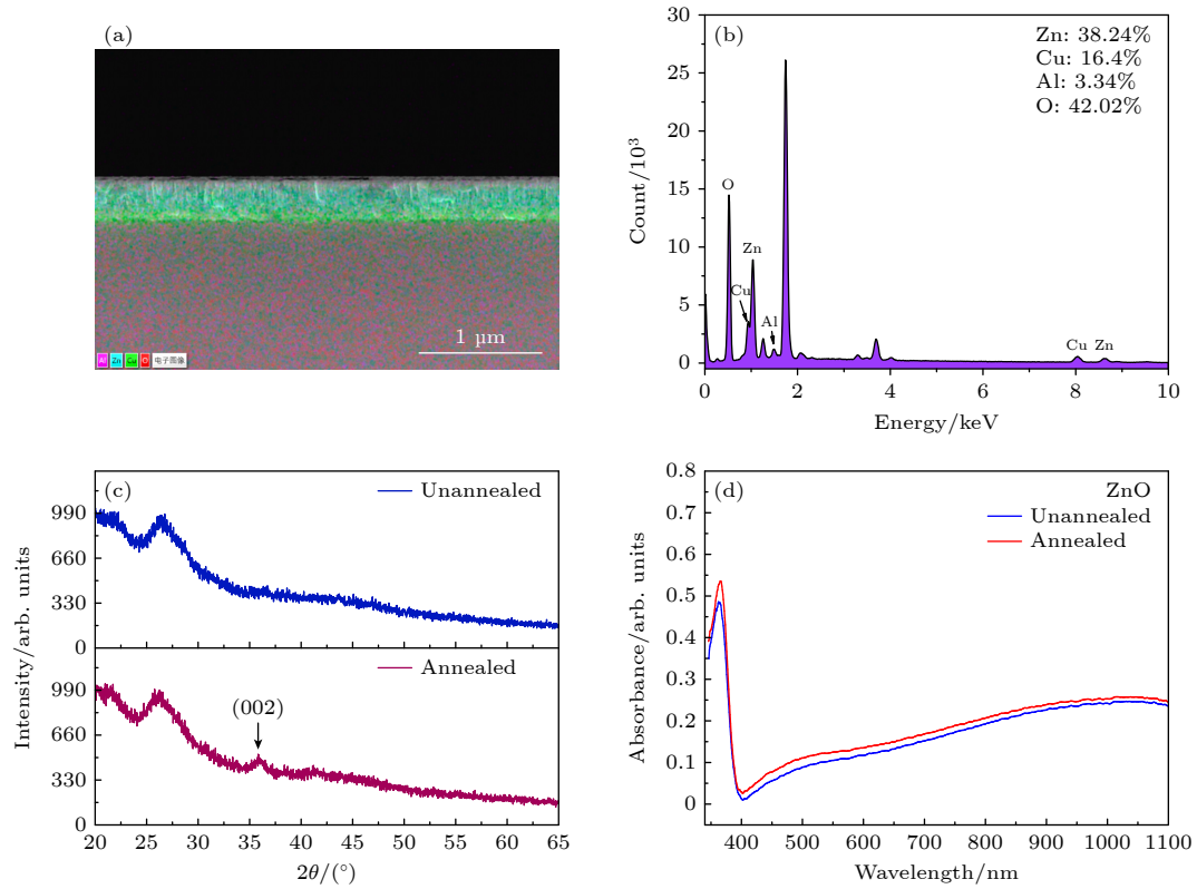
图3 (a) CuO/Al 2 O 3 /ZnO 异质结器件横截面 EDS 形貌及其 (b) 对应区域的 EDS 能谱; ZnO 薄膜退火前后的 (c) XRD 谱和 (d) 吸收光谱
