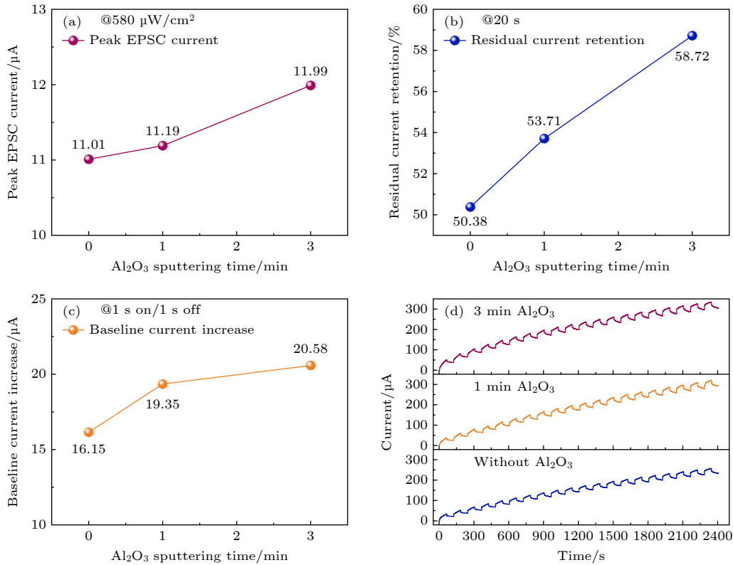
图 8 \text{Al}_2\text{O}_3 间隔层对 \text{CuO}/\text{Al}_2\text{O}_3/\text{ZnO} 器件关键突触参数及循环重复性的影响 (a) 580 \mu\text{W}/\text{cm}^2 , 1 s 紫外光脉冲下 3 种器件的峰值兴奋性突触后电流; (b) 360 \mu\text{W}/\text{cm}^2 , 20 s 光照条件下 50 s 时 3 种器件的残余电流保持率; (c) 360 \mu\text{W}/\text{cm}^2 , 1 s on/1 s off 脉冲条件下 3 种器件的基线电流抬升量; (d) 360 \mu\text{W}/\text{cm}^2 , 1 min 光照/1 min 黑暗循环条件下 3 种器件的重复性测试
