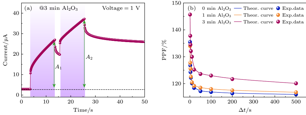
图 9 CuO/Al 2 O 3 /ZnO 器件的成对脉冲促进特性 (a) 3 min Al 2 O 3 器件在两次紫外脉冲刺激下的兴奋性突触后电流响应, A_1 和 A_2 分别为第 1 和第 2 脉冲峰值; (b) 3 种器件的配对脉冲促进随脉冲间隔 \Delta t 的变化 (球形点) 及双指数拟合曲线 (实线)
