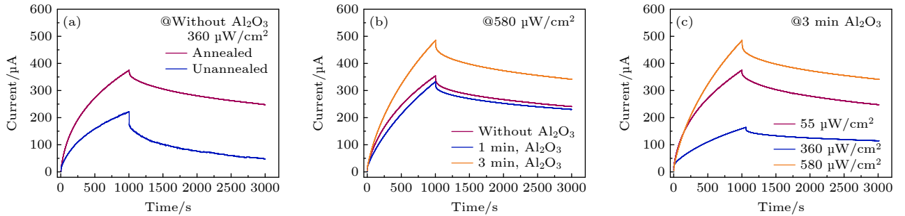
图5 CuO/Al 2 O 3 /ZnO 器件在紫外照射下的 I - T 变化曲线 Fig. 5. I - T curves of CuO/Al 2 O 3 /ZnO devices under UV irradiation.
