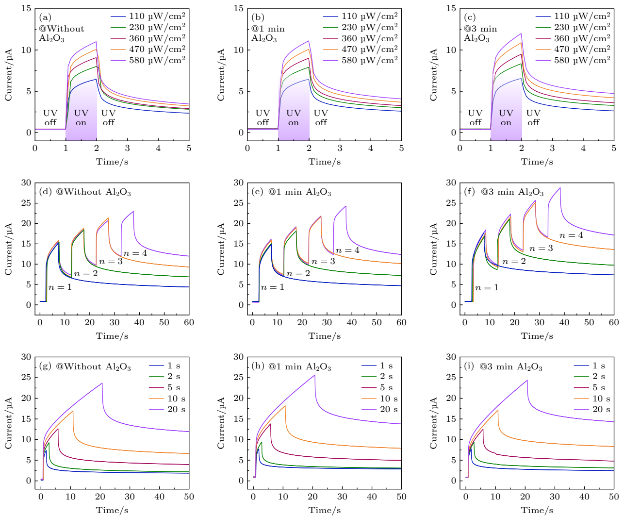
图 6 CuO/Al 2 O 3 /ZnO 器件的类突触学习与记忆行为 (a)—(c) 不同紫外光功率密度下 1 s 单脉冲诱导的兴奋性突触后电流; (d)—(f) 360 \mu\text{W}/\text{cm}^2 , 5 s 光照/5 s 黑暗循环脉冲下, 兴奋性突触后电流随脉冲次数的演化; (g)—(i) 360 \mu\text{W}/\text{cm}^2 下, 不同单脉冲照射时长 (1, 2, 5, 10, 20 s) 诱导的兴奋性突触后电流响应
