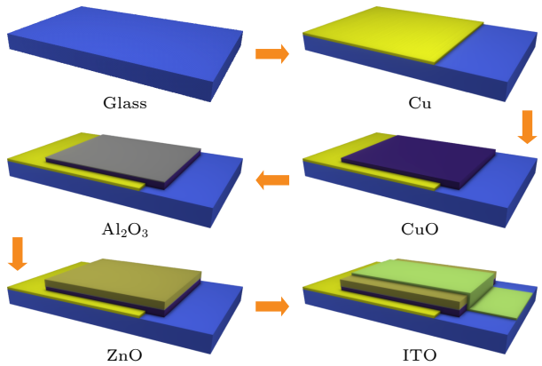
图 1 CuO/Al 2 O 3 /ZnO 异质结器件的制备过程与结构示意图
