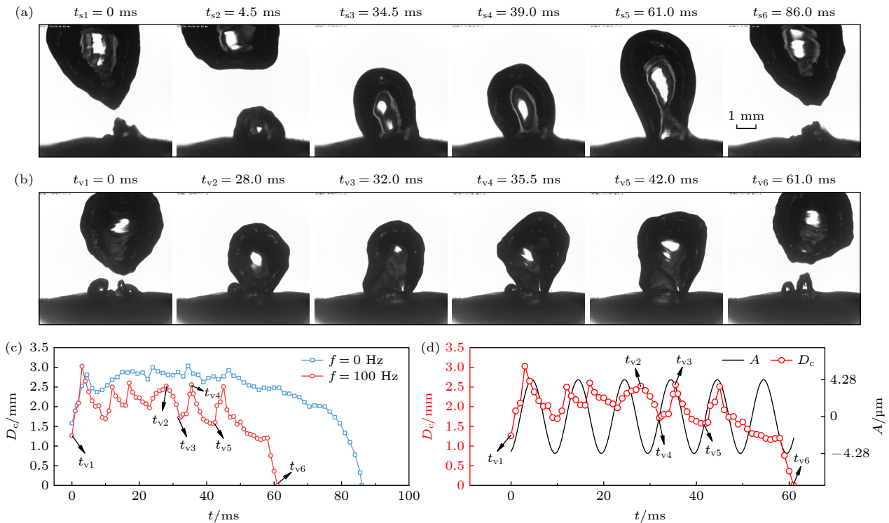
图 7 q = 700 \text{ kW/m}^2 时的气泡动力学 (a) 无振动时气泡脱离图像; (b) f = 100 Hz 时气泡脱离图像; (c) 气泡基圆直径; (d) 气泡基圆直径与柔性板振幅耦合
