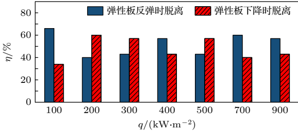
图 8 气泡脱离时柔性板状态比例
