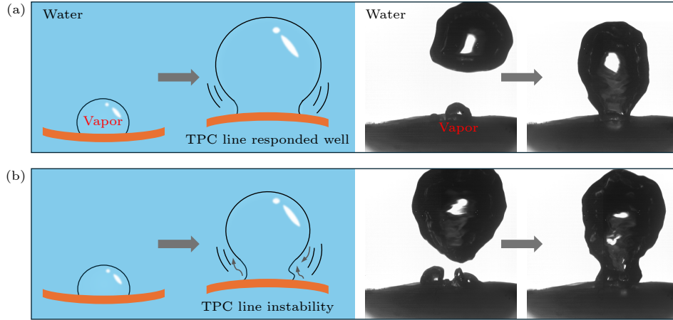
图 5 气泡脱离类型 (a) 浮力主导脱离; (b) 柔性板振动主导脱离
