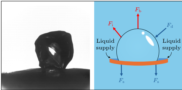
图 11 柔性板下降时强化气泡脱离机理
