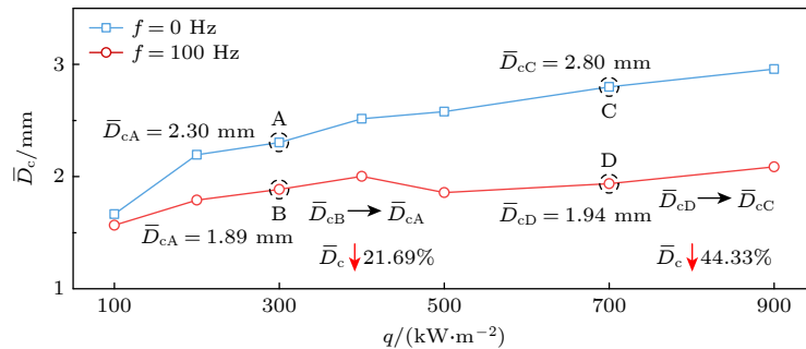
图 4 热流密度与平均基圆直径关系
