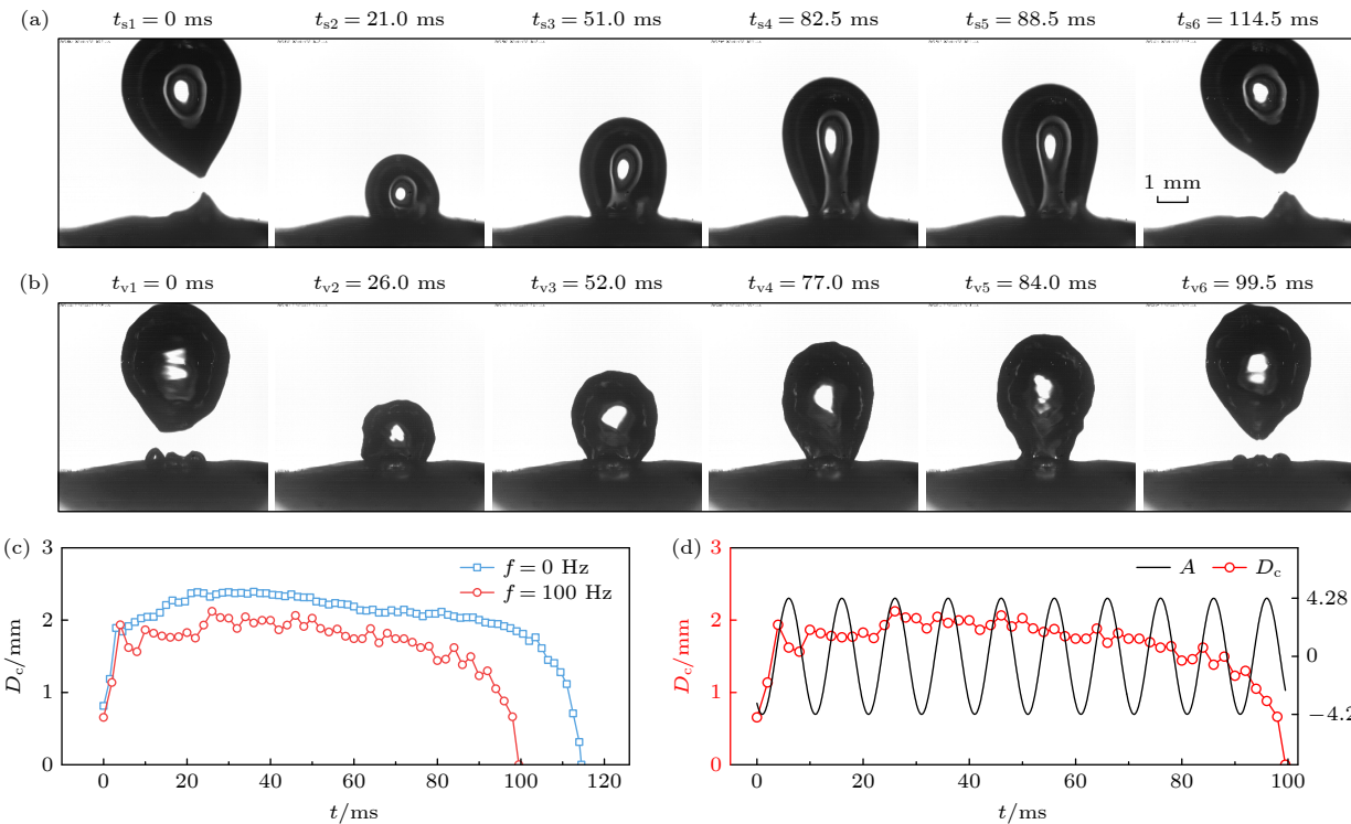
图 6 q = 300 \text{ kW/m}^2 时的气泡动力学 (a) 无振动时气泡脱离图像; (b) f = 100 \text{ Hz} 时气泡脱离图像; (c) 气泡基圆直径; (d) 气泡基圆直径与柔性板振幅耦合
