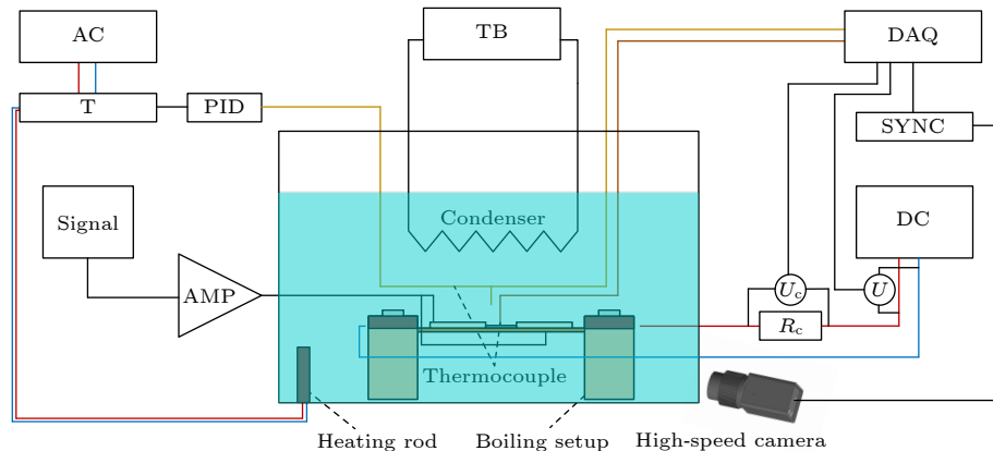
图 1 实验系统
