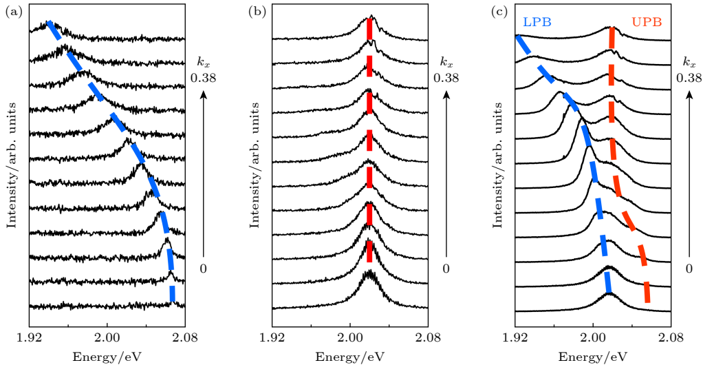
图 3 (a) 纯 PC, (b) 单层 \text{WS}_2 , (c) \text{WS}_2/\text{PC} 器件归一化 PL 谱, 动量从 k_x = 0 到 k_x = 0.38 。图中数据提取自相应的光谱, 蓝色虚线为激子极化激元下支, 红色虚线为激子极化激元上支
