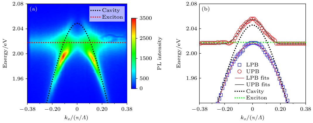
图 2 (a) 单层 \text{WS}_2 -PC 复合器件的动量分辨 PL 谱, 显示出明显的反交叉极化激元模式; (b) 激子极化激元上下两支色散曲线实验 (从图 (a) 获得) 和拟合结果
