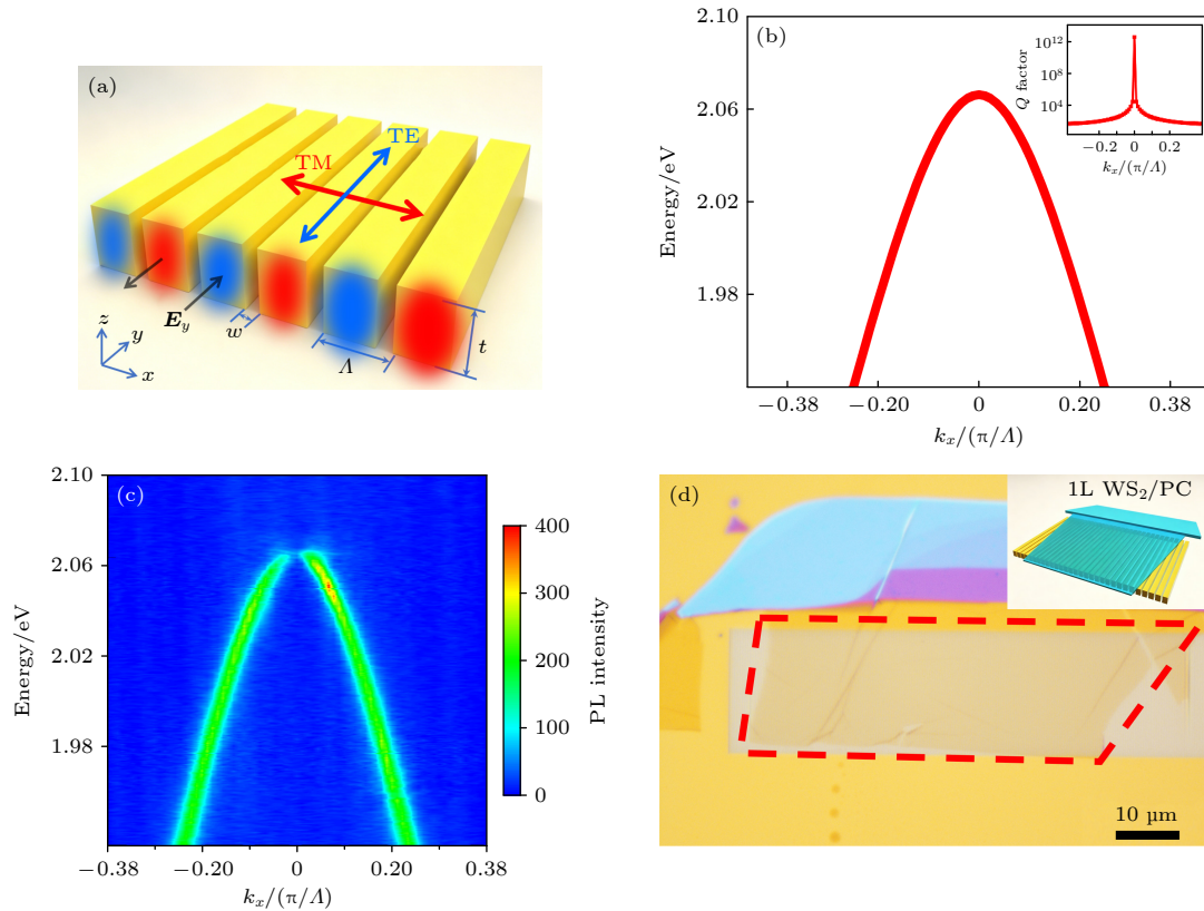
图 1 (a) SiN x 光栅结构和 TE 模式电场分布示意图, 电场 E_y 的方向由红色和蓝色表示, 分别沿着 y 轴方向和 -y 轴方向; (b) SiN x 光栅光子晶体的光子色散和品质因子 (插图) 模拟结果; (c) SiN x 光栅光子晶体的光子色散测量结果; (d) 100 倍显微镜下单层 WS 2 转移到 SiN x 光栅表面的光学照片, 以及单层 WS 2 /SiN x PC 复合器件示意图 (插图)
