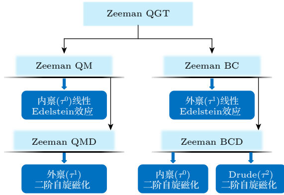
图 2 自旋磁化的塞曼量子几何理论框架
