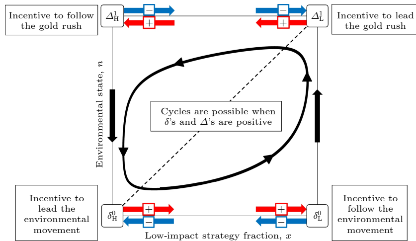
图 2 参数对于相空间周期振荡动力学的影响示意图, 详细信息请见参考文献 [18] . 依据 CC BY 4.0 许可使用
