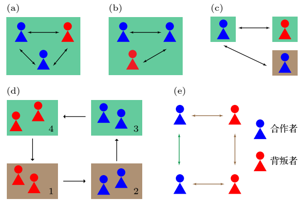
图1 环境反馈博弈示意图,其中蓝色个体为合作者,红色个体为背叛者,个体间的双向箭头示意存在交互连边,绿色背景(连边)为丰裕环境,棕色背景(连边)为贫瘠环境
