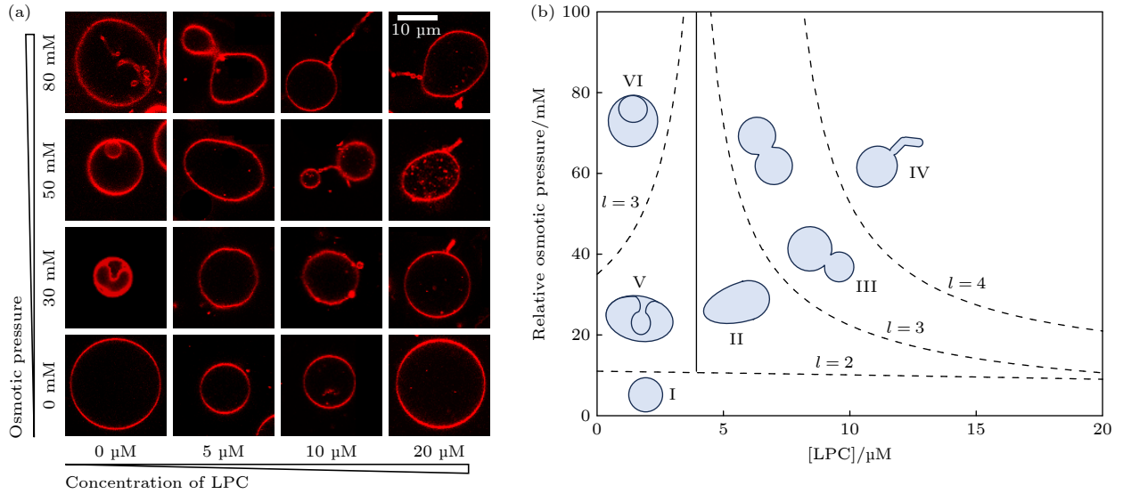
图4 LPC浓度与渗透压差对囊泡形变稳态形貌的协同调控 (a) 不同参数组合下囊泡的共聚焦形变稳态图像; (b) 形态相图, 随LPC浓度(横轴)和渗透压差(纵轴)变化的形貌分区(I–VI). 图中分区边界为根据实验数据点的统计结果绘制的指导性曲线, 相邻数据点之间的实际转变区间存在由参数采样分辨率和形态分布涨落引入的不确定性
