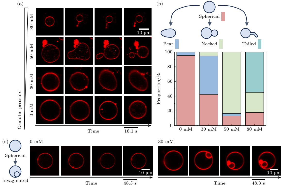
图3 自发曲率符号调控渗透压诱导的囊泡形变图 (a) 正自发曲率囊泡在不同跨膜渗透压差下的形变示意图; (b) 对应 (a) 中不同渗透压差下囊泡稳定后的形态统计; (c) 负自发曲率囊泡在低渗透压差下的形变图
