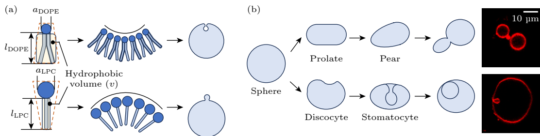
图 1 不同混合磷脂构成的不同曲率囊泡及通过渗透压差调控约化体积的囊泡形态变化示意图 (a) 分子形状控制自发曲率; (b) 体积减小时囊泡的形变, 正曲率下为长椭球到梨形, 负曲率下为盘形到内凹口形
