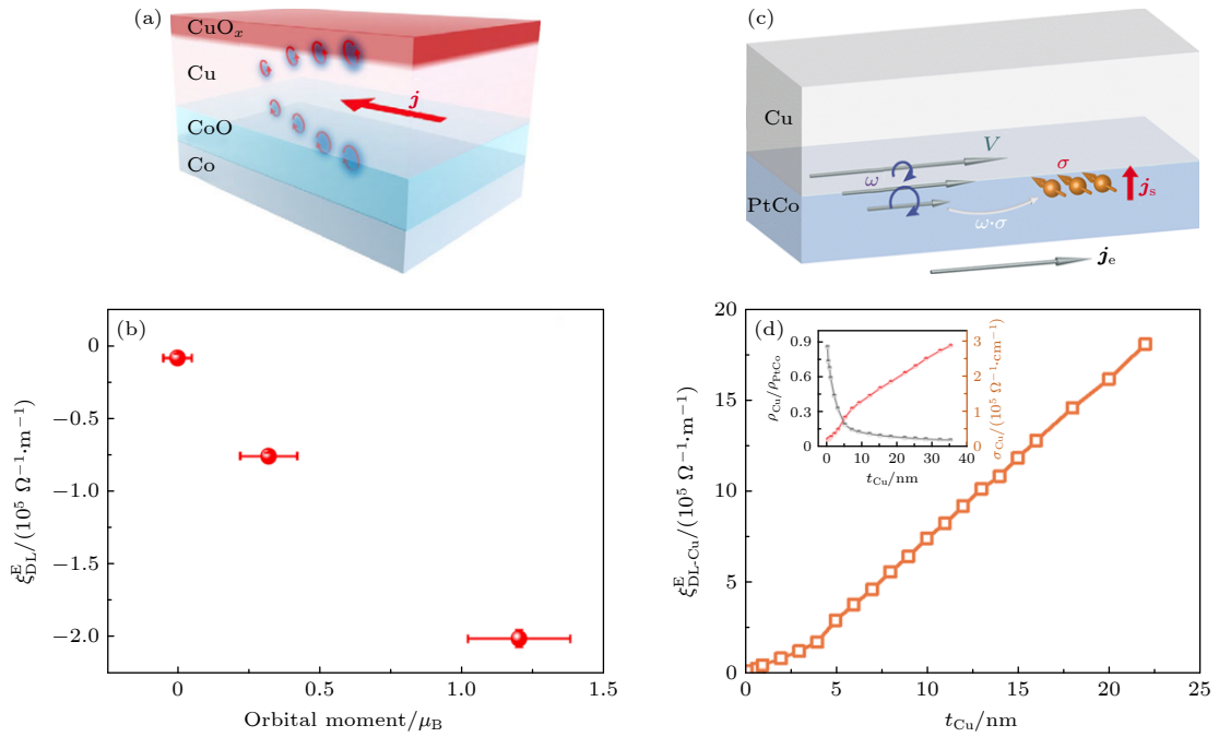
图 8 轨道矩效率的调控 (a), (b) CuO x /CoO/Co 体系中 CoO 的轨道磁矩调控轨道矩效率示意图和轨道矩效率随轨道磁矩变化关系 [83] ; (c), (d) Cu/PtCo 体系中界面自旋-涡度耦合调控轨道矩效率示意图和轨道矩效率随 Cu 厚度变化关系, 插图为 Cu/PtCo 电阻率比随 Cu 厚度变化关系 [84]
