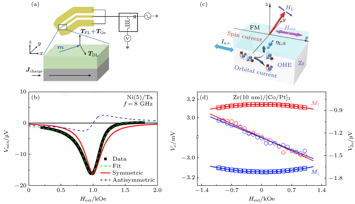
图6 非磁/铁磁异质结中的轨道矩效率测量方法 (a), (b) 利用自旋力矩-铁磁共振方法测量 Ta/Ni 异质结中轨道矩效率示意图及其测量曲线 [37] ; (c), (d) 利用谐波霍尔电压方法测量 Zr/[CoPt] 3 异质结中轨道矩效率示意图及其测量曲线 [10]
