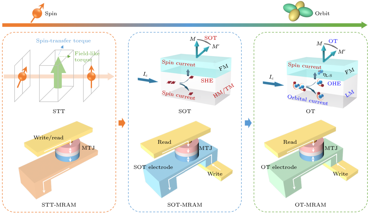
图 1 自旋转移矩、自旋轨道矩和轨道矩磁性随机存储器物理机制和原型器件 [10]
