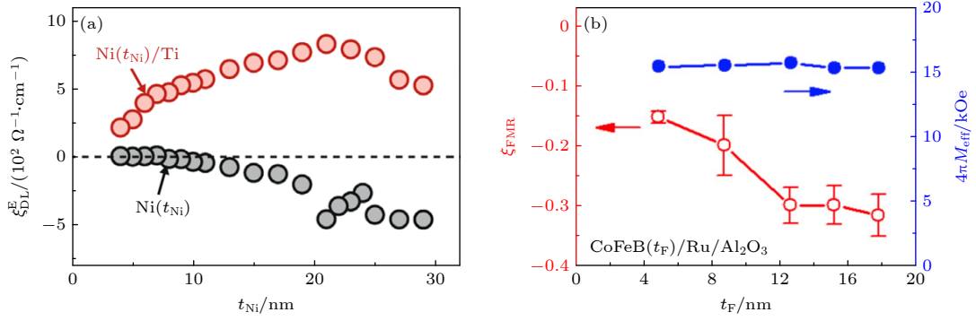
图 7 轨道流在铁磁材料中的长程输运特性 (a) Ti/Ni 体系的轨道矩效率随 Ni 厚度的变化 [21] ; (b) CoFeB/Ru/Al 2 O 3 体系的轨道矩效率随 CoFeB 厚度的变化 [80]
