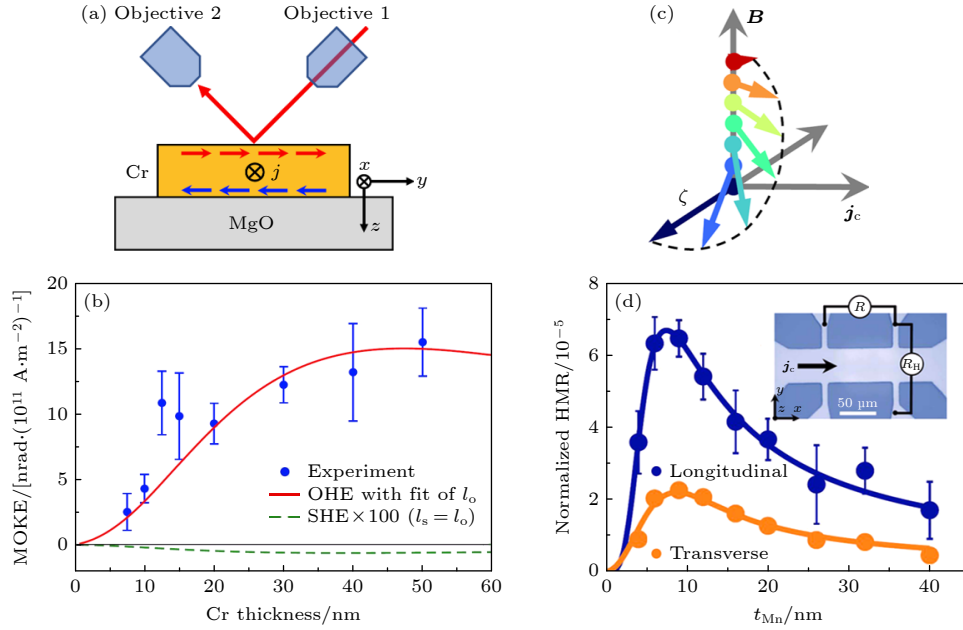
图 5 轨道霍尔材料的轨道霍尔角测量方法 (a), (b) 利用磁光克尔效应方法测量轻金属 Cr 的轨道霍尔效应示意图及磁光克尔角与 Cr 厚度的依赖关系 [63] ; (c), (d) Mn 中 Hanle 磁电阻产生机制和测量示意图以及 Mn 的 Hanle 磁电阻与 Mn 厚度的依赖关系 [31] Fig. 5. Orbital Hall angle and the measurement methods in orbital Hall materials: (a), (b) Schematic of orbital Hall effect measurement in light metal Cr by magneto-optical Kerr effect and the dependence of the magneto-optical Kerr rotation on Cr thickness [63] ; (c), (d) schematic of the generation mechanism and measurement of Hanle magnetoresistance in Mn, and the dependence of Hanle magnetoresistance on Mn thickness [31] .
