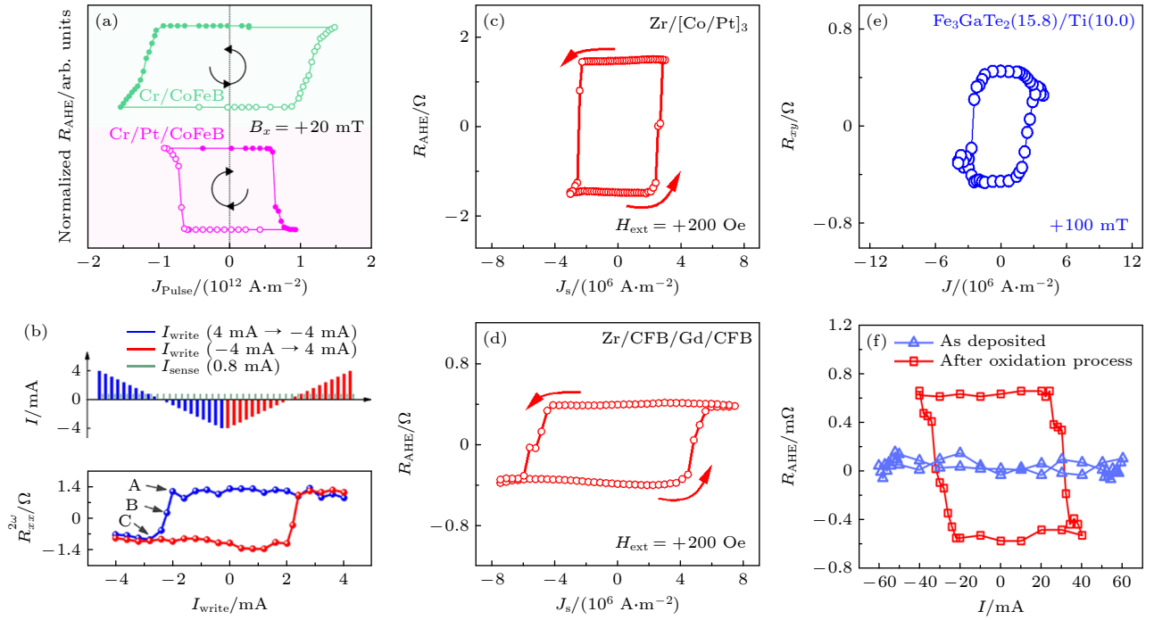
图 9 轨道矩驱动磁化翻转 (a) Cr/Pt/CoFeB [25] ; (b) CuO x /CoFeB [86] ; (c) Zr/[CoPt] 3 [10] ; (d) Zr/CoFeB/Gd/CoFeB [10] ; (e) Ti/Fe 3 GaTe 2 [22] ; (f) CuO x /Cu/Mn 3 Sn [48]
