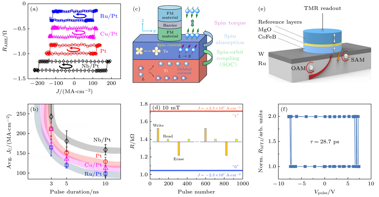
图 10 轨道矩驱动磁隧道结 (a), (b) Ru/Pt/磁隧道结 [43] ; (c), (d) Ti/Ta/磁隧道结 [50] ; (e), (f) Ru/W/磁隧道结 [49]
