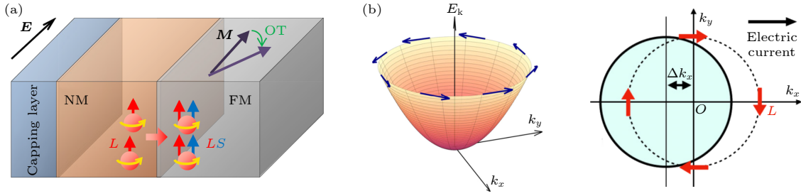
图3 轨道 Rashba-Edelstein 效应机制图 (a) 轨道 Rashba-Edelstein 效应产生轨道流示意图 [56] ; (b) 动量空间轨道 Rashba-Edelstein 效应机制图 [14,56]
