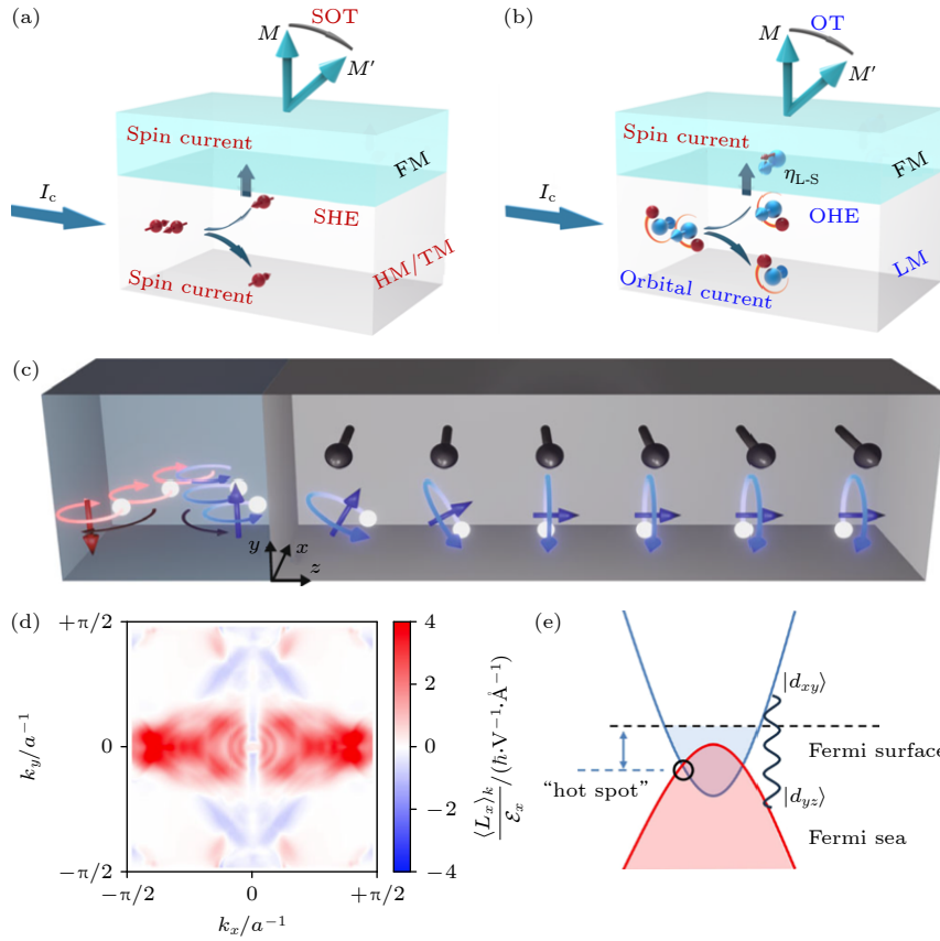
图 4 轨道矩产生机制 (a) 自旋轨道矩和 (b) 轨道矩机制对比 [10] ; (c) 轨道流在铁磁材料中通过轨道热点运输与磁矩作用机制图 [21] ; (d) 动量空间中轨道角动量分布 [57] ; (e) 轨道热点产生示意图 [51]
