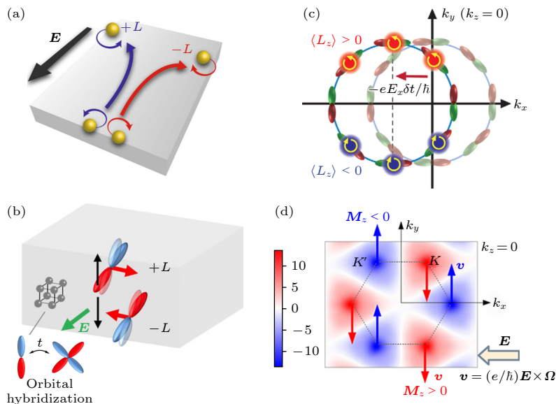
图 2 轨道霍尔效应机制图 (a) 轨道霍尔效应产生轨道流示意图 [14] ; (b) 轨道杂化产生轨道霍尔效应机制图 [51] ; (c) 轨道杂化在动量空间中形成轨道织构机制图 [18] ; (d) 轨道磁矩诱导轨道霍尔效应机制图 [52]
