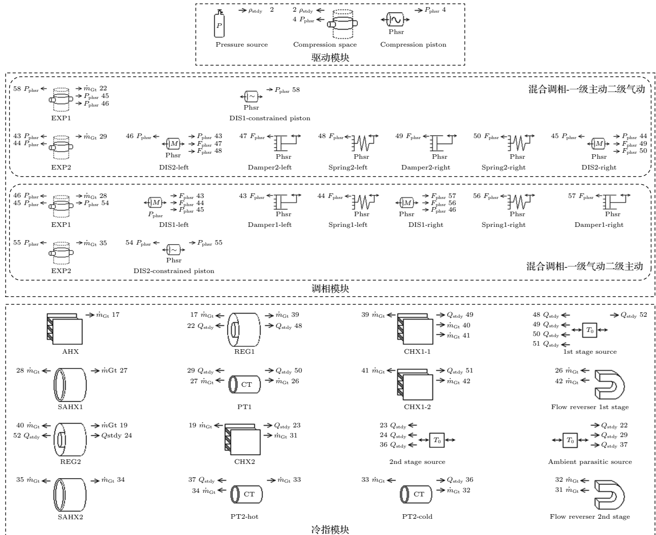
图 2 采用混合调相机结构的斯特林型两级脉管制冷机 Sage 模型
