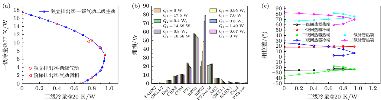
图 3 一级气动-二级主动混合调相模拟结果 (a) 最大冷量调节范围; (b) 各部件焓损; (c) 压力波与体积流相位差
