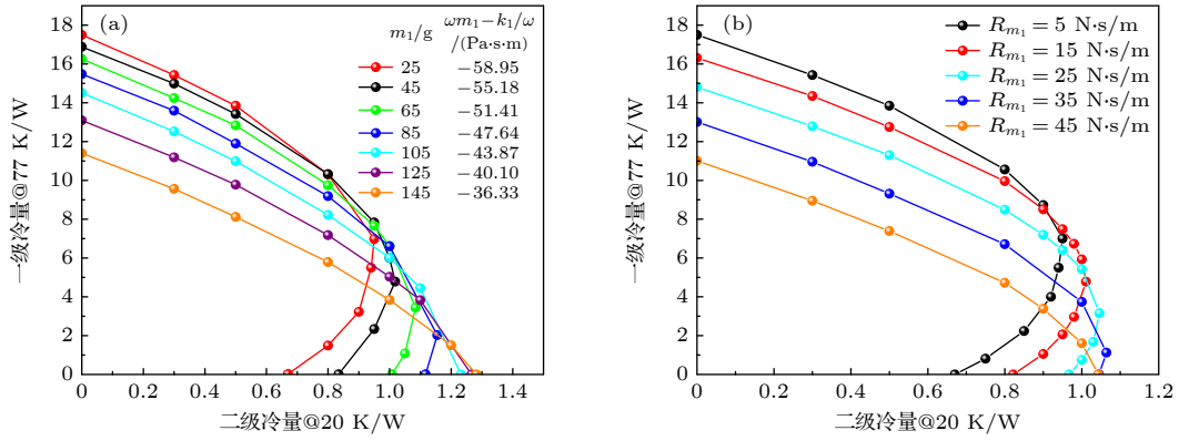
图 4 一级气动排出器参数对系统制冷性能的影响 (a) 动质量; (b) 机械阻尼
