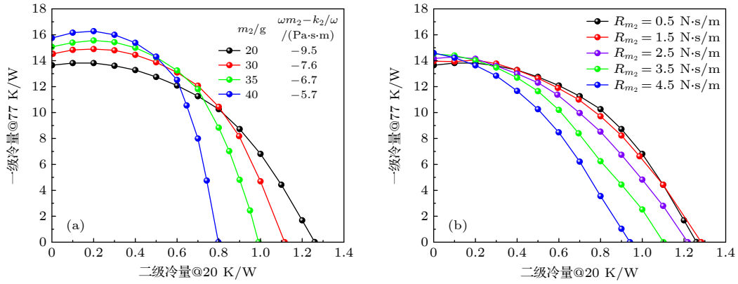
图6 二级气动排出器参数对系统制冷性能的影响 (a) 动质量; (b) 机械阻尼
