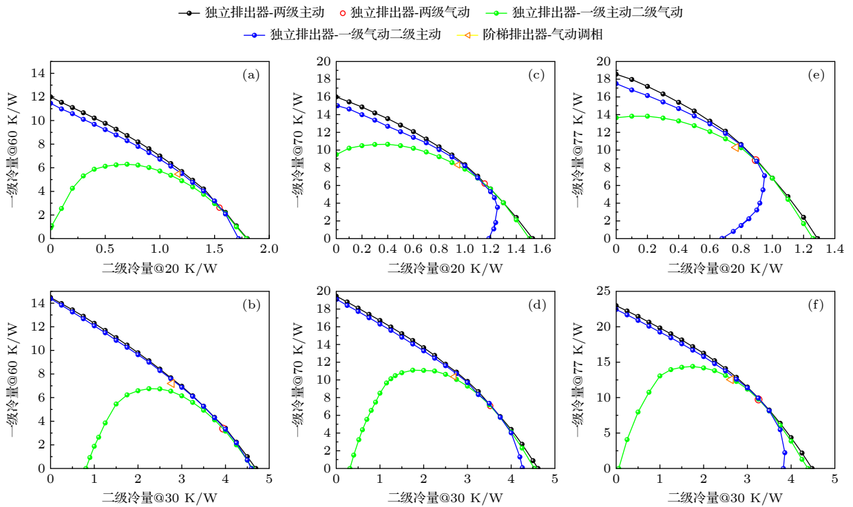
图7 不同调相方式的级间冷量调控范围 (a) 60—20 K; (b) 60—30 K; (c) 70—20 K; (d) 70—30 K; (e) 77—20 K; (f) 77—30 K
