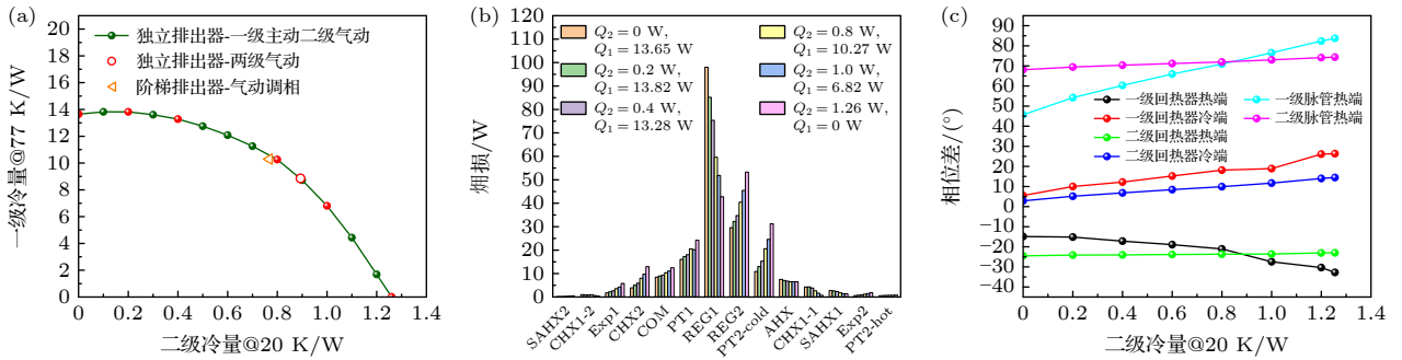
图 5 一级主动-二级气动混合调相模拟结果 (a) 最大冷量调节范围; (b) 各部件熵损; (c) 压力波与体积流相位差
