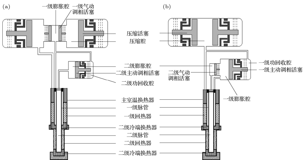
图 1 采用混合调相的两级脉管制冷机结构示意图 (a) 一级气动-二级主动调相; (b) 一级主动-二级气动调相
