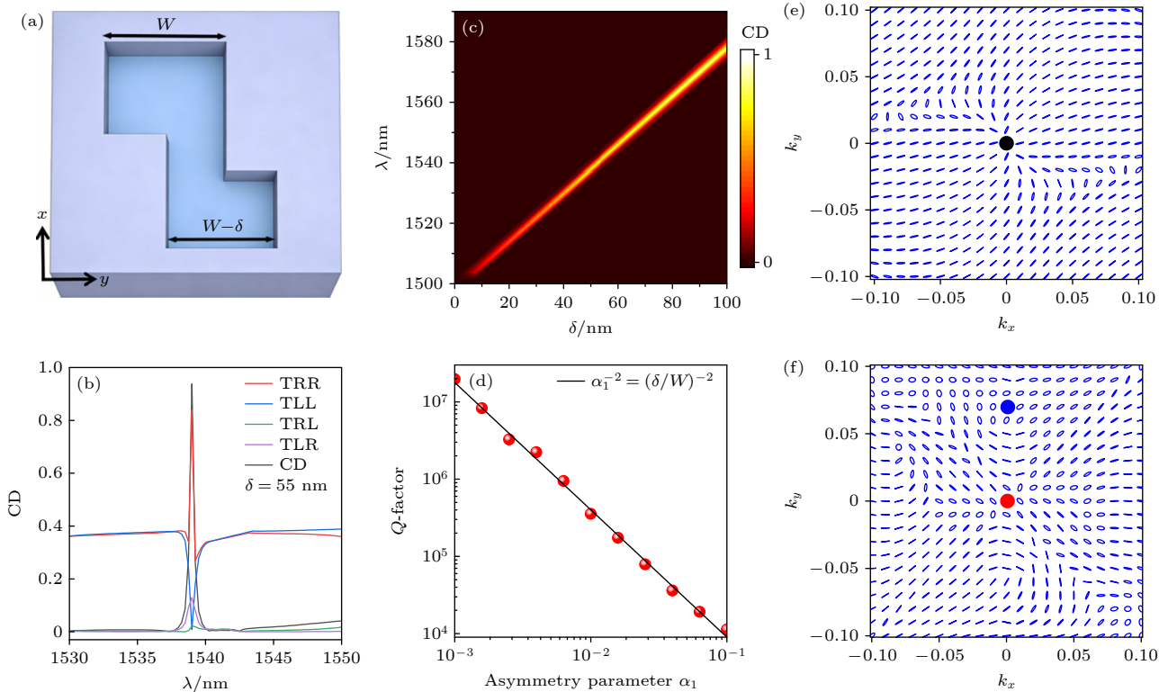
图 3 结构面对称性破缺时超表面的手性响应分析 (a) 单胞俯视图 (引入面内不对称参数 \delta ); (b) \delta = 55 nm 时, 各分量透射率及其圆二色性; (c) 随不对称参数 \delta 连续变化的 CD 演化光谱; (d) 品质因子 (红点) 和对应的拟合曲线 (黑线) 随几何不对称参数 \alpha_1 = \delta/W 的变化; (e), (f) \delta = 0, 55 nm 时的本征偏振图, 其中黑点 ( V 点)、红点 ( C_+ 点)、蓝点 ( C_- 点)
