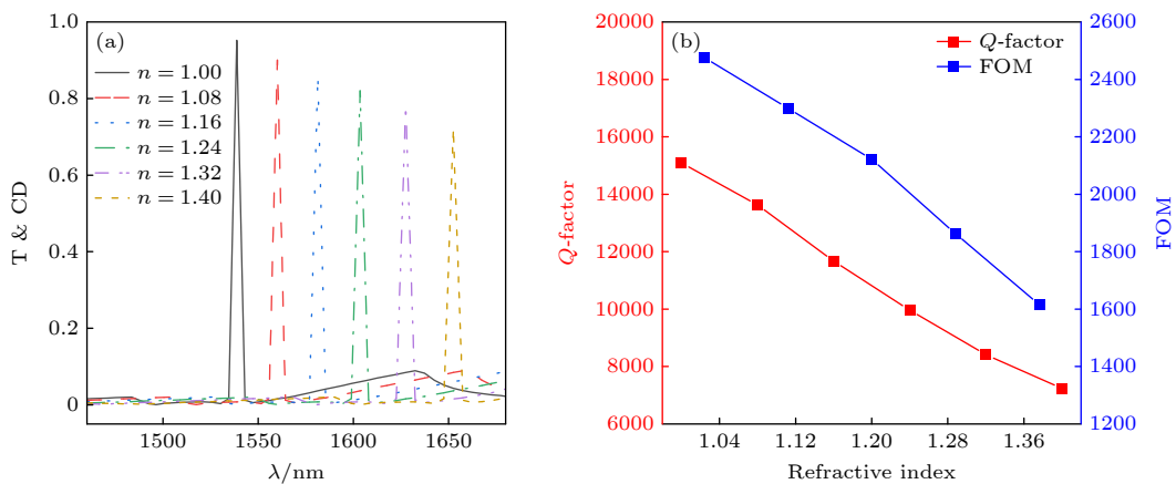
图 7 传感器性能分析 (a) CD 峰位移与折射率的关系; (b) 品质因子 Q 随待测物质折射率变化的演变图以及 FOM 分析
