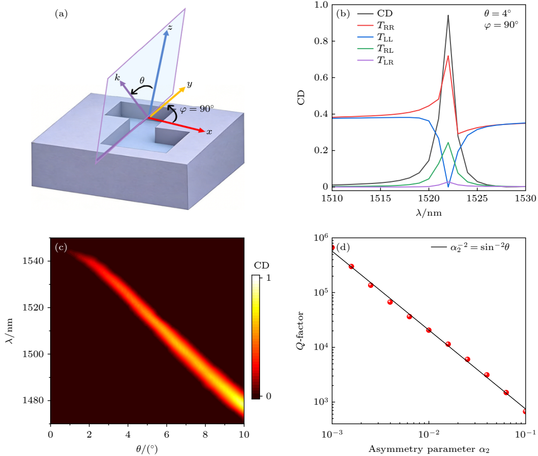
图 5 斜入射时超表面的手性响应分析 (a) 引入光照不对称参数 \theta 且固定 \varphi = 90^\circ 的单晶胞俯视图; (b) \theta = 4^\circ , \varphi = 90^\circ 时的各透射分量及 CD 光谱; (c) 随光照不对称参数 \theta 连续变化的 CD 演化光谱; (d) 品质因子 (红点) 和对应的拟合曲线 (黑线) 随不对称参数 \alpha_2 = \sin\theta 的变化
