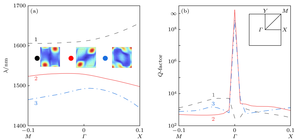
图 2 手性超表面的本征模式分析 (a) 能带结构, 插图显示了各模式的场模式 (颜色: 磁场分布, 箭头: 电矢量); (b) K 空间中 Q 因子, 插图显示的是第一布里渊区
