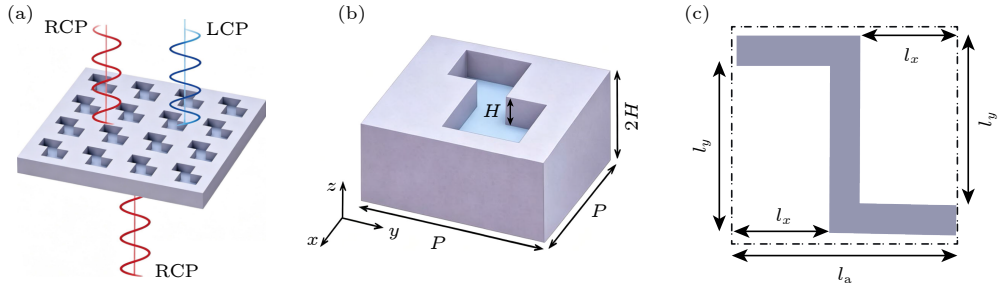
图 1 (a) 支持手性准 BIC 光子晶体硅平板示意图, 红色和蓝色分别表示 RCP 和 LCP 光; (b), (c) 超表面单元胞结构示意图
