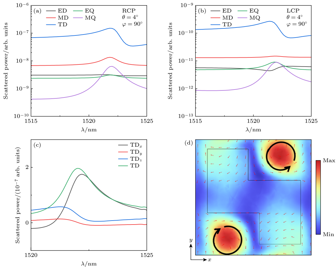
图 6 斜入射时 ( \theta = 4^\circ , \varphi = 90^\circ ) 准 BIC 模式的多极子分解与电磁场分布 (a) RCP 入射下的多极子散射功率; (b) LCP 入射下的多极子散射功率; (c) TD 极子的贡献分量; (d) x - y 平面下的磁场分布, 其中红色箭头代表电场矢量, 黑色箭头表示电流旋向
