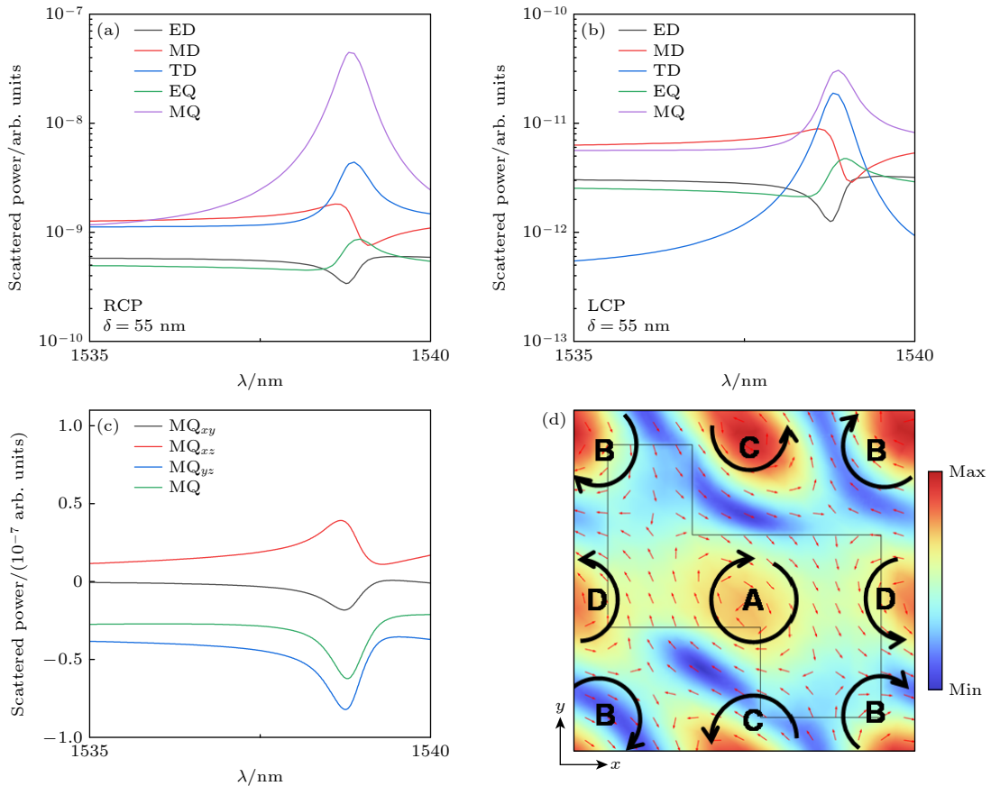
图 4 面内不对称时 ( \delta = 55 nm) 准 BIC 模式的多极子分解与电磁场分布 (a) RCP 入射下的多极子散射功率; (b) LCP 入射下的多极子散射功率; (c) MQ 极子的贡献分量; (d) x - y 平面下的磁场分布, 其中红色箭头代表电场矢量, 黑色箭头表示电流旋向
