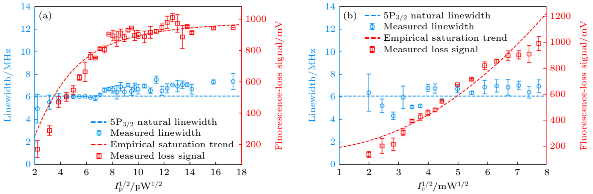
图 3 探测光和耦合光功率变化对冷原子 MOT 荧光损失谱特征参数的影响. 蓝色圆圈为由高斯拟合得到的谱线半高全宽, 蓝色虚线表示 ^{87}\text{Rb} 5P_{3/2} 态自然线宽参考; 红色方块为测得的荧光损失峰强度 (对应右侧纵轴), 红色虚线为经验饱和和趋势曲线 S(P) = S_0 + A\kappa/(1 + 2\kappa) , 其中 \kappa = P/P_s : (a) 固定耦合光功率 I_c = 40 \text{ mW} , 扫描探测光功率 I_p , 并取 P_{s,p}^{\text{th}} \approx 24.0 \mu\text{W} ; (b) 固定探测光功率 I_p = 100 \mu\text{W} , 扫描耦合光功率 I_c , 并取 ARC 计算得到的 5P_{3/2} \rightarrow 46D_{3/2} 本征饱和功率 P_{s,c}^{\text{th}} \approx 6.52 \text{ W} . 误差棒表示多次独立测量的标准差
