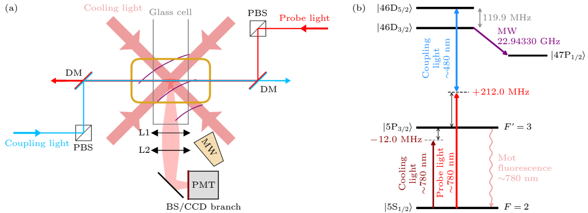
图 1 冷原子 MOT 荧光损失谱测量的实验装置和能级示意图 (a) 实验核心装置示意图. 二维磁光阱制备的长条形冷原子云位于玻璃腔中心, 探测光 (probe light) 和耦合光 (coupling light) 在入射前经偏振分束器 (polarizing beam splitter, PBS) 反射并选定为竖直偏振, 再经双色镜 (dichroic mirror, DM) 合束至原子云轴向; 冷却光 (cooling light) 用于维持 MOT 连续运行. MOT 荧光经由 L_1 , L_2 构成的双透镜成像系统收集后, 由普通分束器 (beam splitter, BS) 分至光电倍增管 (photomultiplier tube, PMT) 和 CCD 成像支路. 微波 (microwave, MW) 天线从侧向辐照原子云. (b) 双光子里德伯激发和微波耦合能级图. 780 nm 探测光 (probe light) 耦合 5S_{1/2}, F=2 \rightarrow 5P_{3/2}, F'=3 跃迁, 480 nm 耦合光 (coupling light) 进一步激发至 46D_{3/2} 或 46D_{5/2} 里德伯态; f_0 = 22.94330 \text{ GHz} 的微波场共振耦合 46D_{3/2} \rightarrow 47P_{1/2} 跃迁; 波浪箭头表示 5P_{3/2}, F'=3 \rightarrow 5S_{1/2}, F=2 的 MOT 荧光辐射
