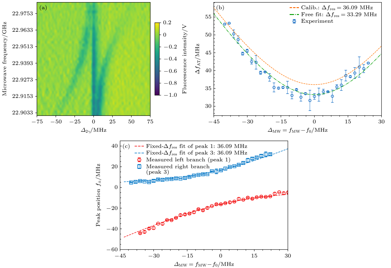
图 5 不同微波频率下的里德伯态 AT 分裂谱及失谐响应 (a) 7.5 dBm 下扫描微波频率得到的荧光损失谱; (b) Peak 1 和 Peak 3 同时可分辨时的 \Delta f_{\text{AT}} = f_3 - f_1 , 橙色虚线采用图 4(b) 标定的 \Delta f_{\text{res}} = 36.09 MHz, 绿色点划线为本图数据自由拟合; (c) Peak 1/ Peak 3 分支轨迹及固定 \Delta f_{\text{res}} 的拟合
