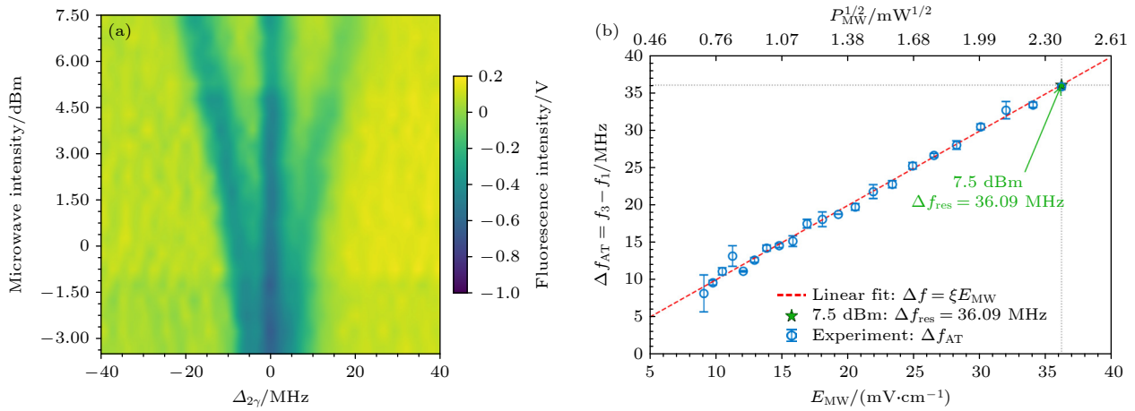
图4 不同微波强度下的 MOT 荧光损失谱与 AT 分裂 (a) 固定微波频率 22.94330 GHz 时的荧光损失谱伪彩图, 左右峰为 AT 缀饰峰, 中心峰为残余未耦合或弱耦合通道; (b) 左右峰间距 \Delta f_{AT} 与微波电场强度 E_{MW} 的关系, 上方坐标为 \sqrt{P_{MW}} , 星号标出 7.5 dBm 工作点及由功率标定得到的 \Delta f_{res} \approx 36.09 MHz, 该值用于图 5(b) 的失谐 AT 模型曲线
