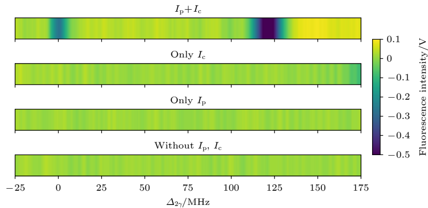
图 2 有无探测光耦合光作用下的 MOT 荧光信号伪彩图. 图中由上至下分别对应四种实验条件: 1) I_p + I_c : 同步开启探测光与耦合光; 2) Only I_c : 仅开启耦合光; 3) Only I_p : 仅开启探测光; 4) Without I_c, I_p : 关闭探测光和耦合光. 典型光功率为 I_p = 100 \mu\text{W} , I_c = 40 \text{ mW} . 横坐标为双光子失谐量 \Delta_{2\gamma} , 零点定义为 46D_{3/2} 双光子共振位置. 右侧色标为 PMT 输出的 MOT 荧光信号强度 (单位: V). 两条暗带对应 46D_{3/2} 和 46D_{5/2} 里德伯态的双光子激发
