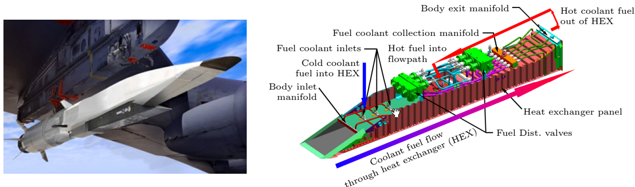
图 1 X-51A 试验飞行器 [1]
