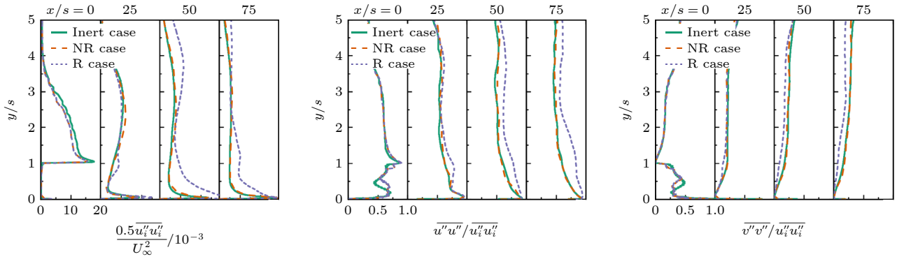
图9 湍动能沿法向分布 (左图) 及其在两个方向分量中的分配情况 [56]
