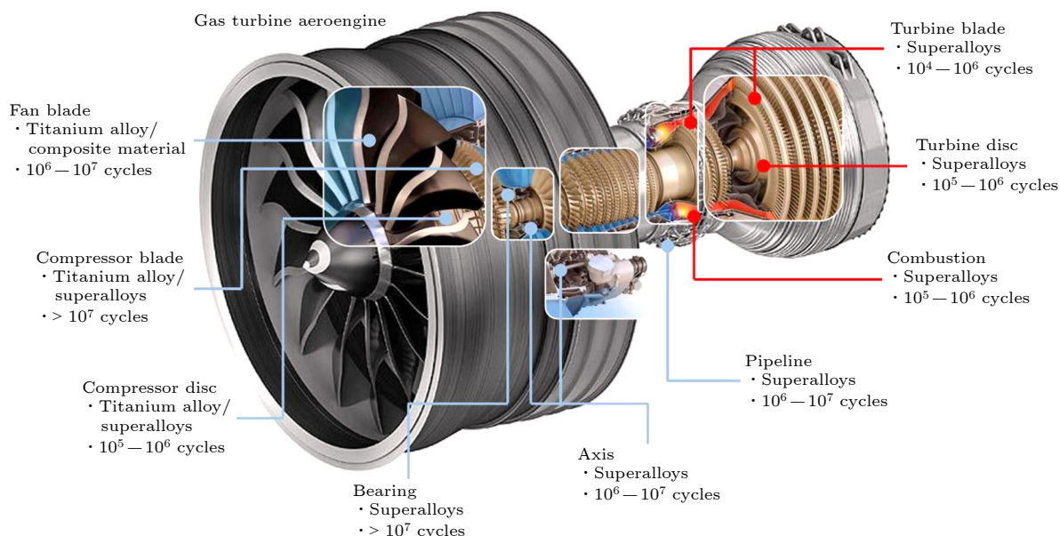
图 17 航空发动机不同零部件及结构的材料类型与疲劳寿命 [109]
