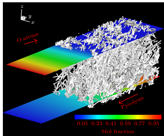
图 15 多孔纤维材料烧蚀介观模拟 [97]
