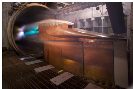
图 2 X-43A 飞行器试验模型 [1]
