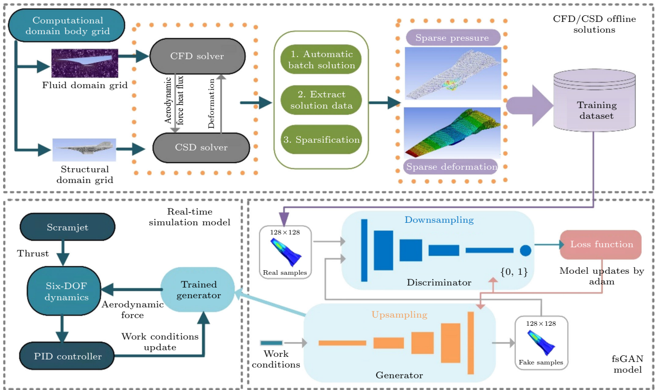
图 25 fsGAN 方法实现飞行器耦合和控制的流程 [172]
