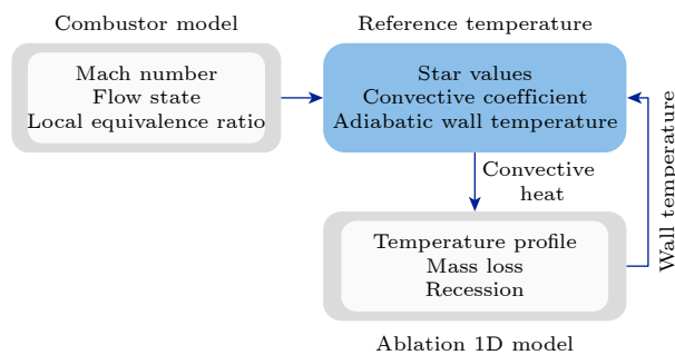
图 16 超燃冲压发动机烧蚀耦合模型 [100]
