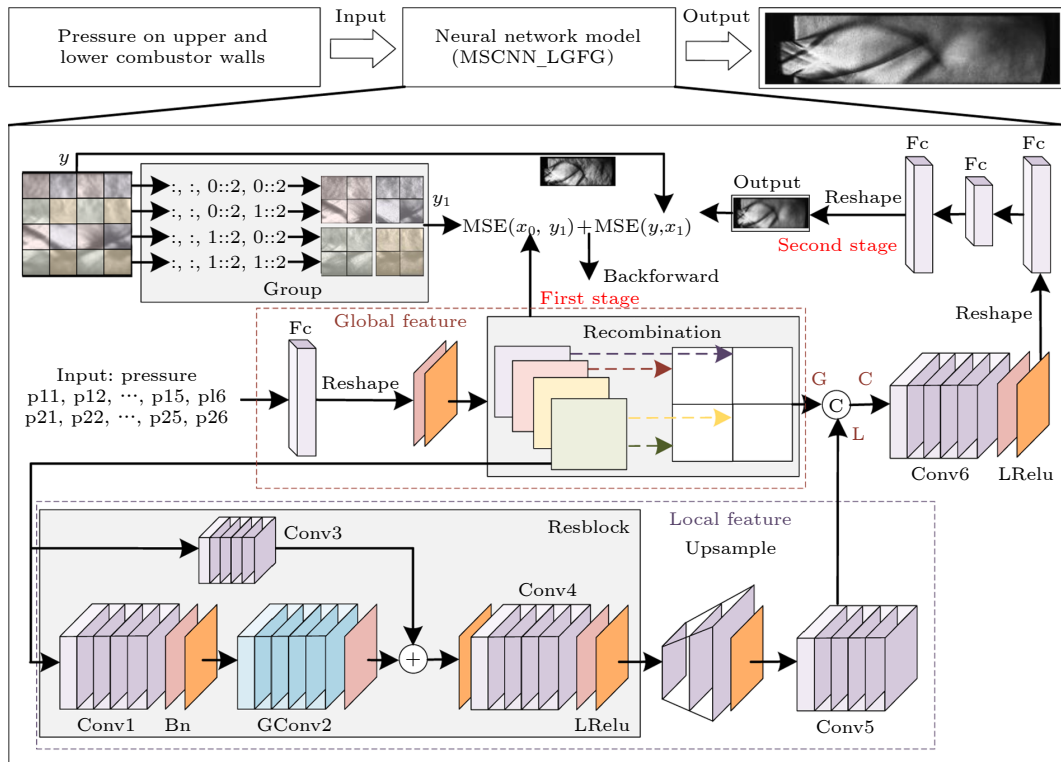
图 23 MSCNN 实现流程 [168]
