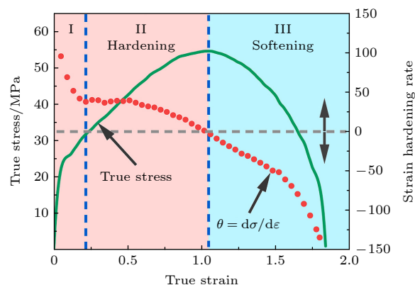
图 12 TNW700 合金的超塑性流动行为及变形机制 [70]
