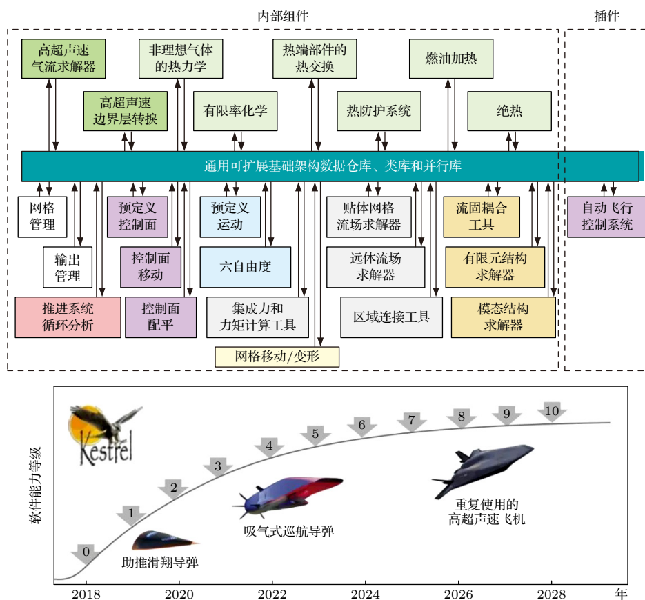
图 3 多物理分析软件 Kestrel 架构 [18]
