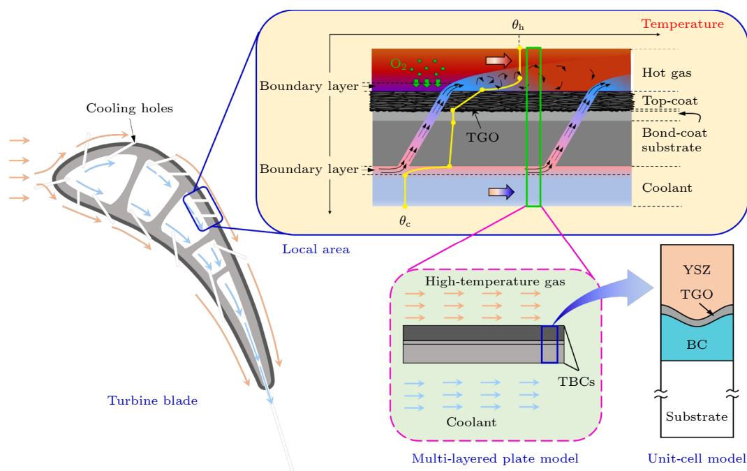
图 13 涡轮叶片热障涂层示意 [79]
