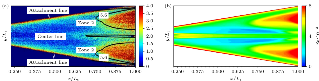
图7 (a) 试验测温的热流分布结果 [37] ; (b) C-\gamma-Re_{\theta_t} 转捩模型预测的热流分布结果 [37]
