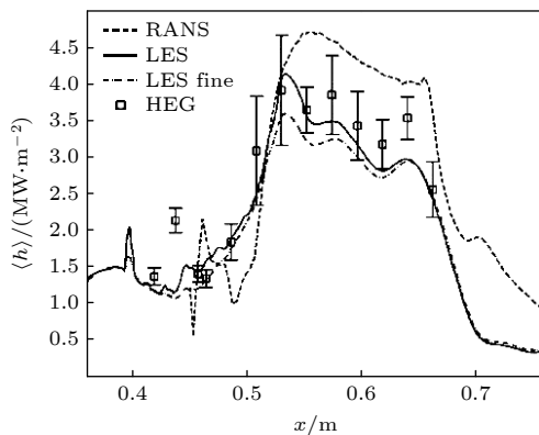
图10 距离喷孔中心线 6 mm 处的热流实验值和仿真值对比 [57]
