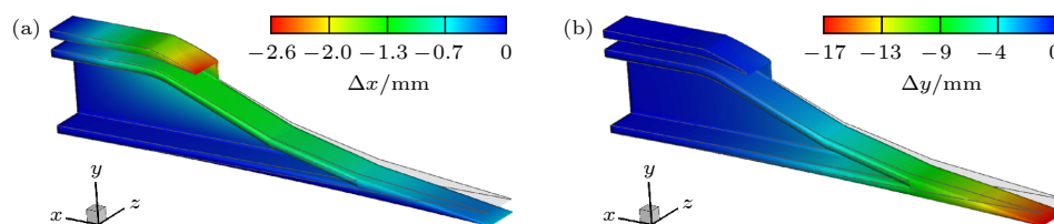
图6 力热耦合下高超声速飞行器进气道的位移形变 [23] (a) x 方向位移; (b) y 方向位移
