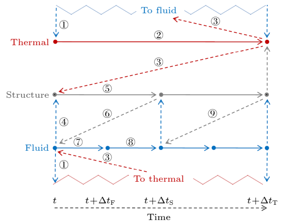
图 21 松耦合策略示意图 [153]
