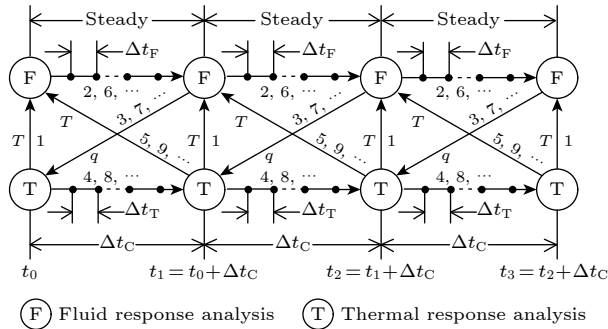
图 22 紧耦合策略示意图 [159]
