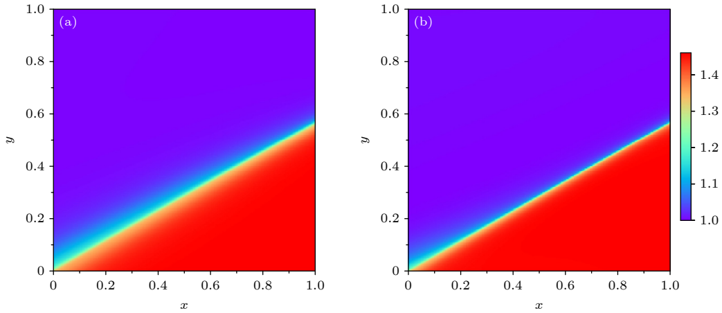
图 24 随机取点 (a) 与间断处取更多点 (b) 还原的密度场 [170]
