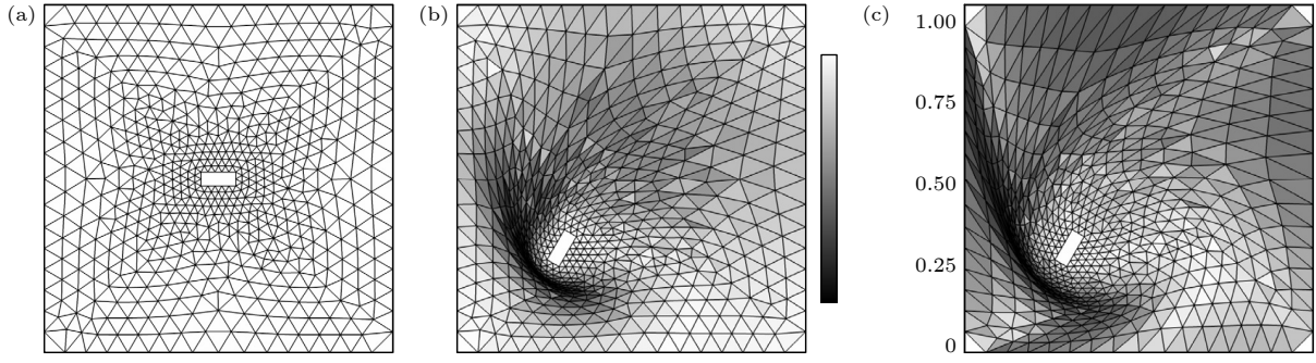
图 19 IDW 与 RBF 方法变形网格质量对比 [146] (a) 原网格; (b) RBF; (c) IDW
