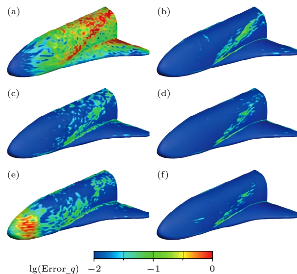
图 18 翼身组合体流体域网格表面热流误差云图 [110] (a) 原始 MQ; (b) 梯度修正 MQ; (c) 原始 TPS; (d) 梯度修正 TPS; (e) 原始紧支 C^2 ; (f) 梯度修正紧支 C^2
