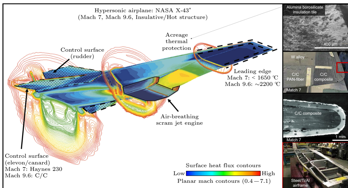
图 11 X-43 热防护结构材料 [61]
