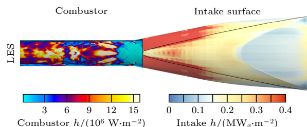
图 8 进气道与燃烧室下壁面的壁面热流密度 [46]
