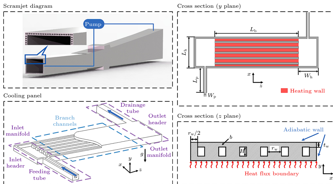
图 14 再生冷却通道示意 [87]
