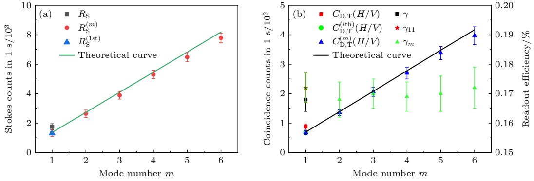
图 3 (a) 不同纠缠源 Stokes 光子数随时间模式数 m 变化关系; (b) Stokes 和 anti-Stokes 光子符合计数和读出效率随时间模式数 m 变化关系
