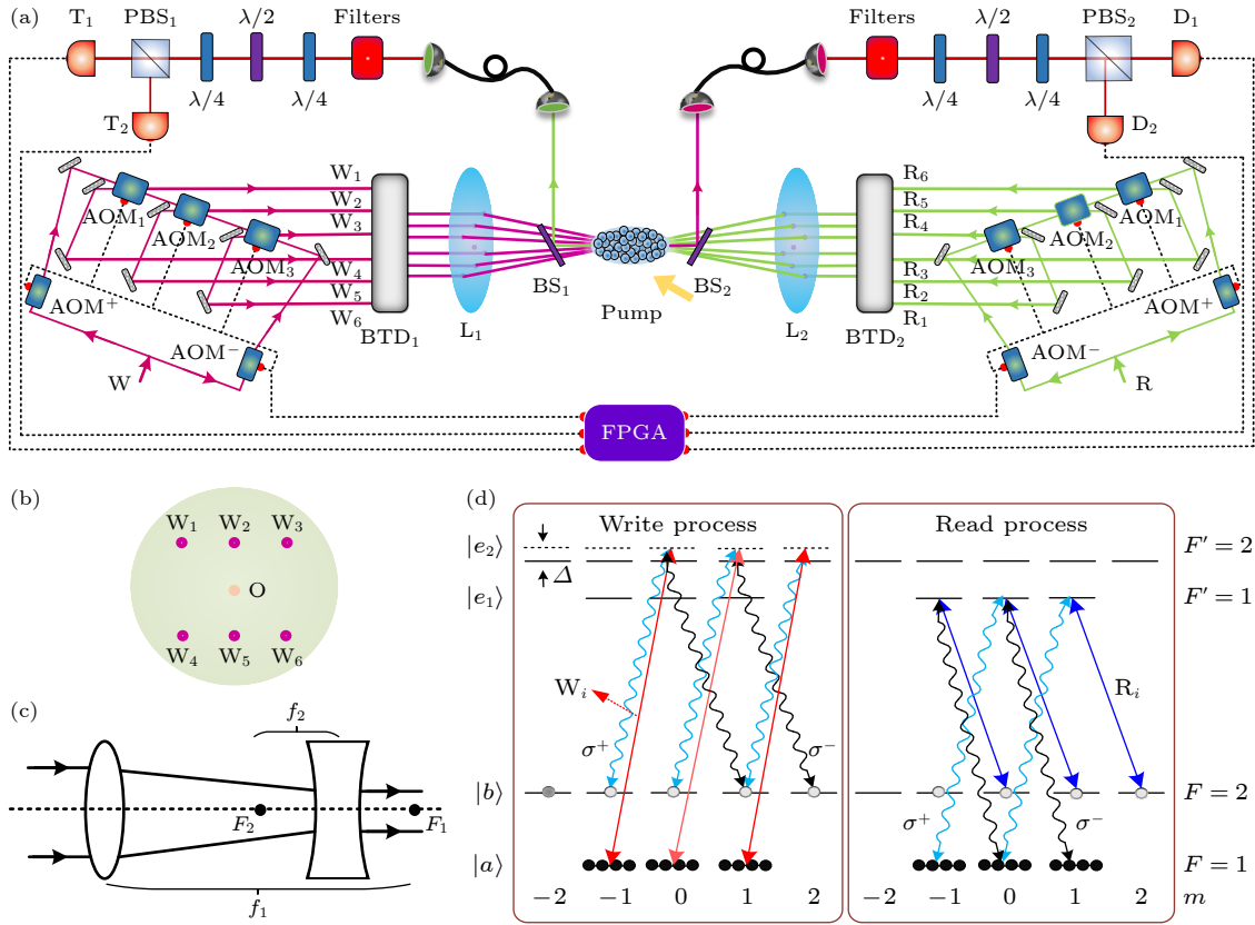
图 1 实验概述 (a) 实验装置图, W_i ( R_i ) 为第 i 路写 (读) 光; AOM 为声光调制器; BTD 为光束变换装置; D(T) 为单光子探测器; Filters 为滤波器组; (b) 光束阵列分布; (c) 光束变换装置结构; (d) 有关原子能级
