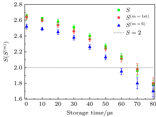
图 4 测量 Bell 参数 S , S^{(m=1st)} , S^{(6)} 与存储时间 \tau 变化关系 Fig. 4. Measurements of the Bell parameter S , S^{(m=1st)} , S^{(6)} as a function of \tau .
