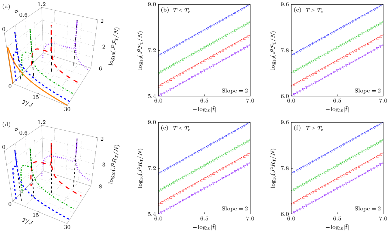
图3 (a) 不同耦合强度下关于温度的量子费舍尔信息 \mathcal{F}_T , 其中橙色实线代表弱耦合近似下的结果, 黑色虚线标注了临界温度; (b), (c) 关系 \mathcal{F}_T \propto |\tilde{t}|^{-2} 相应的对数-对数图, 所有直线均以斜率 2 进行拟合; (d) 不同耦合强度下关于温度的信噪比 R_T , 其中黑色虚线标注了临界温度; (e), (f) 关系 R_T \propto |\tilde{t}|^{-2} 相应的对数-对数图, 所有直线均以斜率 2 进行拟合. 图中, 均取 N = 10^3 , 其余参数与图 1(a) 一致
