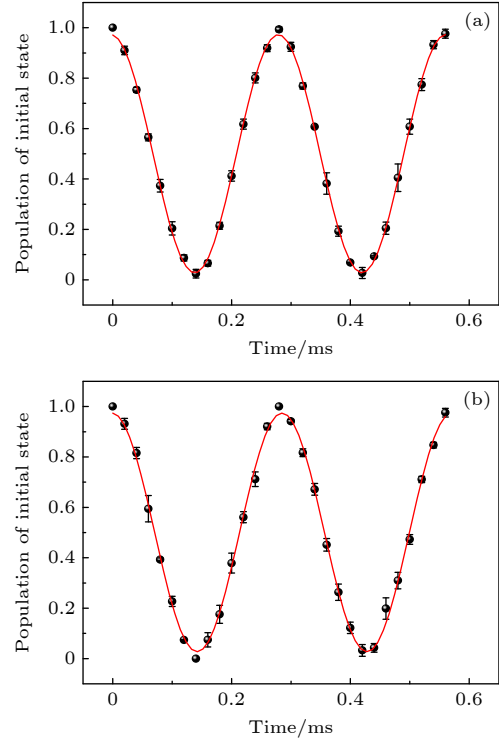
图 5 单个射频时的耦合强度测量 (a) 射频 1, 3.552(8)\pi kHz; (b) 射频 2, 3.498(3)\pi kHz; 黑色点为实验数据, 红色实线为拟合曲线, 实验数据为 3 次测量的平均结果
