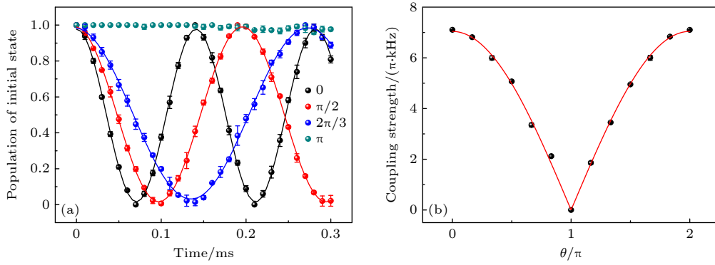
图 7 不同相位差下的耦合强度测量 (a) \theta 为 0, \pi/2, 2\pi/3 和 \pi 时的原子动力学演化过程, 圆点为实验数据, 实线为拟合曲线, 实验数据为 3 次测量的平均结果; (b) \theta 与耦合强度的关系, 圆点为拟合得到的耦合强度, 实线为理论曲线
