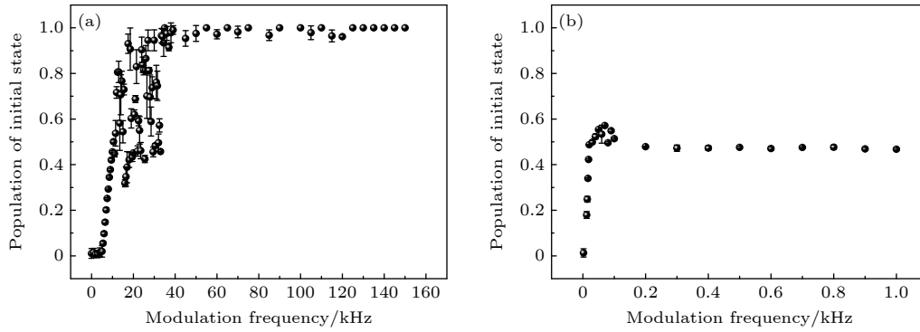
图 8 功率调控与相位调控的响应测量 (a) 功率调控响应测量; (b) 相位调控响应测量; 圆点为实验数据, 实验数据为 3 次测量的平均结果
