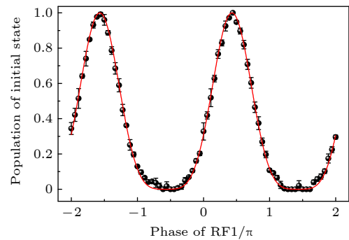
图 6 原子初态布居数与 \theta_{\text{ext}} 的关系, 射频作用时间为 0.07 ms, 黑色点为实验数据, 红色实线为拟合曲线, 实验数据为 3 次测量的平均结果
