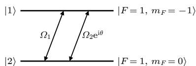
图 1 能级示意图
