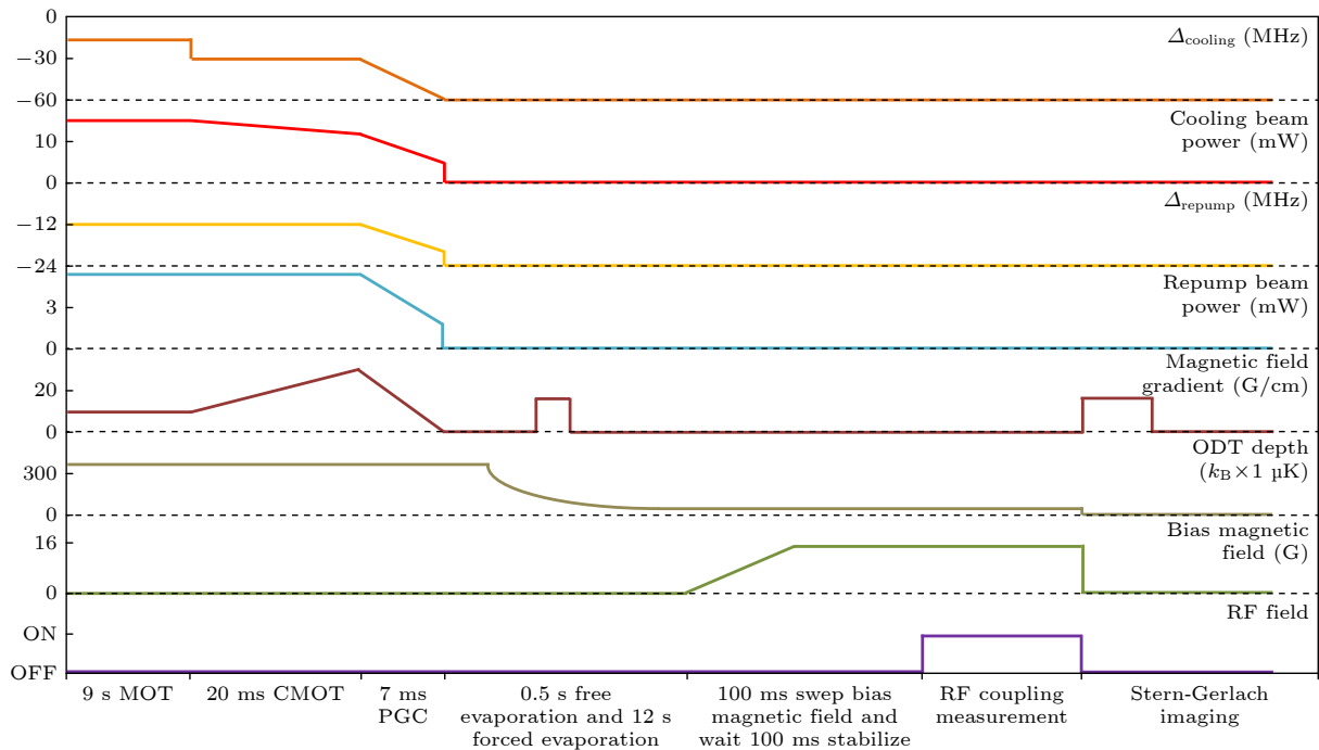
图 4 实验时序
