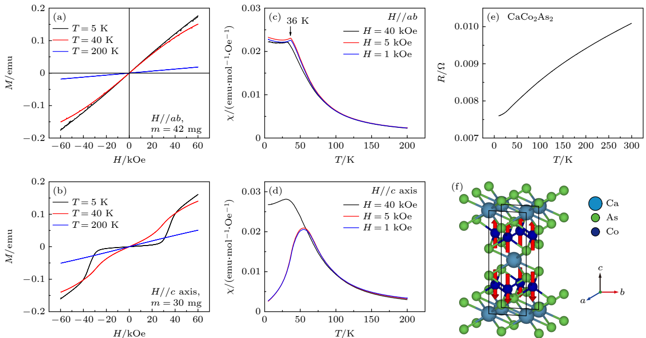
图 1 \text{CaCo}_2\text{As}_2 单晶样品的电输运、磁性表征与磁结构示意图 (a), (b) 分别为 H//ab 和 H//c 时不同温度下的等温磁化曲线; (c), (d) 分别为 H//ab 和 H//c 时不同磁场下的温度依赖磁化率曲线; (e) 电阻 R 随温度 T 的变化; (f) A 型反铁磁结构示意图, Co 磁矩沿 c 轴取向, 在 ab 面内铁磁排列, 沿 c 轴反铁磁排列
