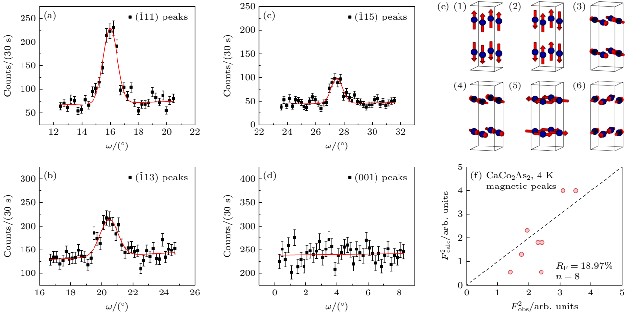
图 3 \text{CaCo}_2\text{As}_2 单晶的低温磁衍射峰、候选磁结构模型与磁结构精修结果 (a)–(c) 4 K 下代表性磁衍射峰 ( \bar{1}\bar{1}1 ), ( \bar{1}\bar{1}3 ) 和 ( \bar{1}\bar{1}5 ) 的 \omega 扫描, 红线为高斯峰与线性背景的拟合结果; (d) 4 K 下 (001) 位置的 \omega 扫描, 未观察到可分辨磁衍射峰; (e) MAXMAGN 给出的 6 种候选磁空间群模型: (1) P14/nnc , (2) P14_2/mnm , (3) C_{Amca} , (4) C_{Amcm} , (5) P1mmn , (6) P1nnm ; (f) P14/nnc 模型下 8 个磁衍射峰的实验积分强度 F_{\text{obs}}^2 与计算强度 F_{\text{calc}}^2 的比较
