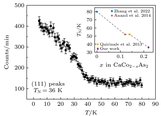
图 4 (111) 磁衍射峰强度随温度的变化. 该磁衍射峰在约 36 K 处消失, 对应奈尔温度 T_N . 插图给出了 Co 缺位浓度 x 与 T_N 的关系, 包括 Zhang 等 [26]、Quirinale 等 [16]、Anand 等 [17] 和本工作的结果. 其中, Zhang 等 [26] 的数据点对应名义满占位的化学计量比 \text{CaCo}_2\text{As}_2 ( x = 0 ), 实际 Co 占位率未经过结构精修准确测定
