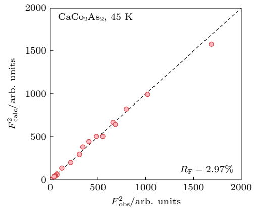
图 2 45 K 单晶中子衍射晶体结构精修质量. 实验积分强度 F_{\text{obs}}^2 与计算积分强度 F_{\text{calc}}^2 相比较, 图中给出了可靠性因子 R_F
