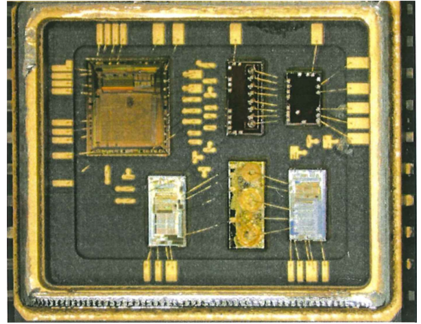
图 3 六裸芯混合封装样品实物图
