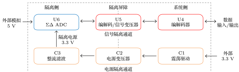
图 1 隔离 \Sigma\Delta ADC 系统结构示意图
