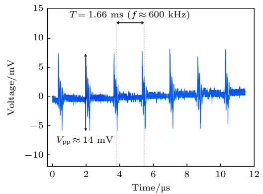
图 6 C_3 芯片整流输出端隔离电源纹波的实测波形
