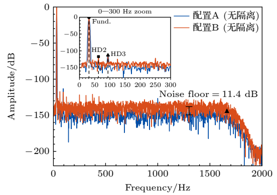
图 5 配置 A 和配置 B 的 ADC 输出频谱对比
