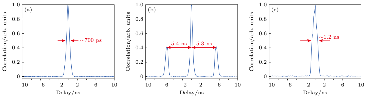
图 3 二阶关联函数特征图 (a) 理想同步状态, 关联函数呈现单峰; (b) 固定延时下, 关联函数呈现清晰的三峰结构 (主峰+对称边带); (c) 脉冲占空比增大, 使关联函数峰形加宽
