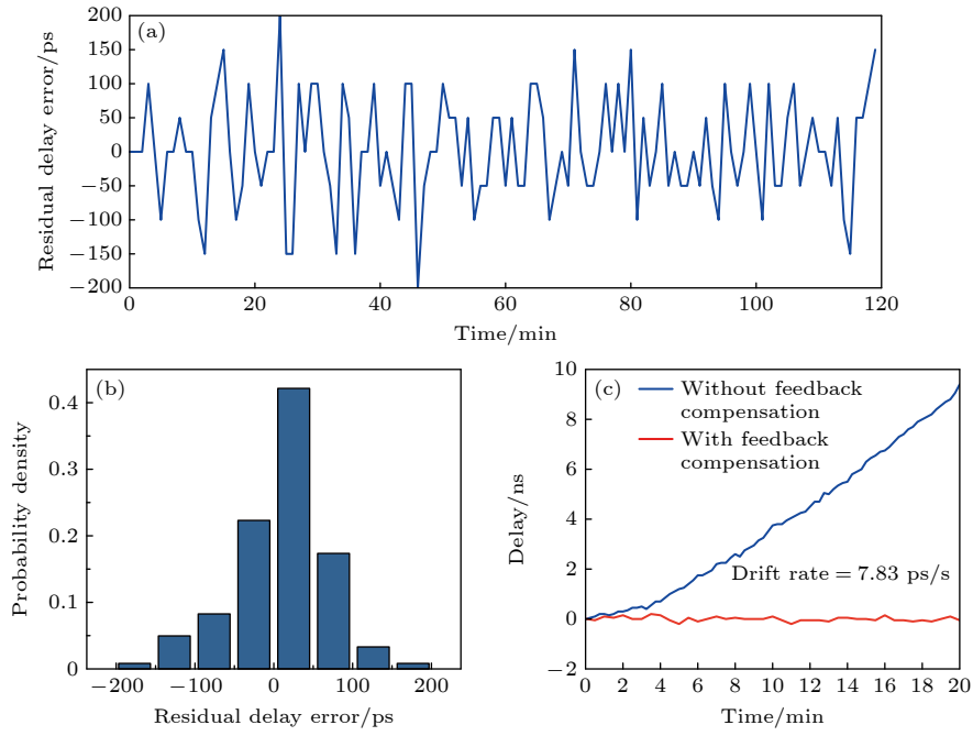
图4 同步性能核心结果图 (a) 静态同步2 h内残余同步误差 \Delta t_{\text{residual}} 的时间序列; (b) 静态同步误差统计直方图; (c) 动态漂移跟踪曲线. 在受控线性温度漂移下, 有/无反馈补偿时, 系统测得的路径延时差 \Delta t 随时间的变化曲线
