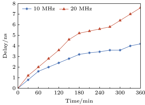
图 2 时钟漂移测试 Fig. 2. Clock drift test.
