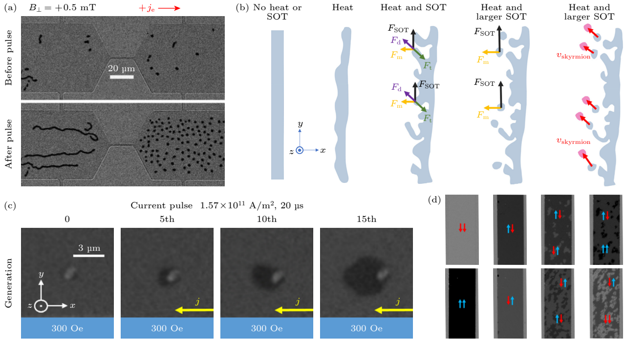
图1 电流诱导磁斯格明子的产生 (a)“吹泡泡模型”产生磁斯格明子泡 [41] ; (b)在表面张力 F_t 、退磁力 F_d 、自旋轨道矩力 F_{\text{SOT}} 和马格努斯力 F_m 作用下条状磁畴转变为斯格明子的示意图 [42] ; (c)利用材料本征缺陷在电流驱动下产生SAF斯格明子泡 [43] ; (d)磁场与电流协同作用实现磁斯格明子与多种磁畴态的相互转换 [44]
