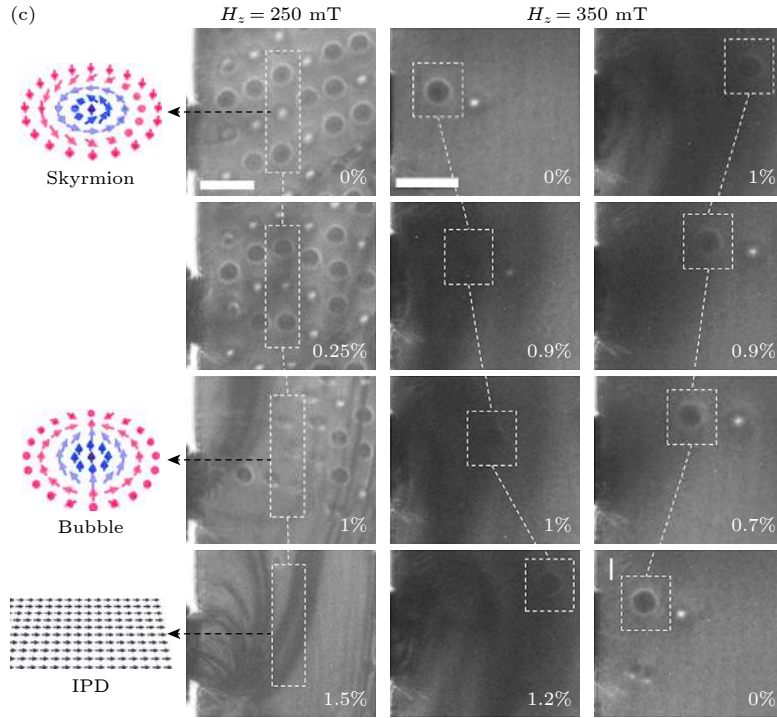
图 4 几何约束、材料工程、局域磁场与力学写入斯格明子 (a) 300 K 时不同宽度的 \text{Fe}_3\text{Sn}_2 纳米带在各自对应临界场下的欠焦洛伦兹透射电镜图像, \text{Fe}_3\text{Sn}_2 纳米带自旋结构随磁场与宽度变化的实验相图, 几何受限效应对 \text{Fe}_3\text{Sn}_2 磁畴演化影响的原理示意图 [62] ; (b) MFM 针尖施加局域磁场在 [\text{Pt}/\text{Co}/\text{Ta}]_n 多层膜中写入能在零磁场和室温下稳定存在的斯格明子晶格 [63] ; (c) 室温洛伦兹透射电镜观测到单轴应变驱动斯格明子由高应变区向低应变区迁移 [33]
