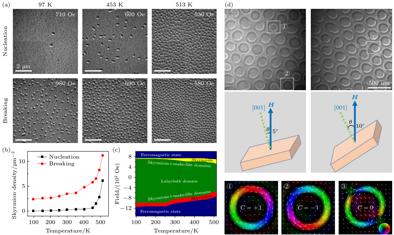
图2 热效应对斯格明子形成的影响 (a) 在 97, 453 和 513 K 温度下, 斯格明子在形核过程与破碎过程中达到最大值时的洛伦兹透射电子显微镜图像 [56] ; (b) 形核过程与破碎过程中斯格明子最大密度随温度的变化关系 [56] ; (c) 磁场降低过程中, 磁畴结构随温度与磁场变化的相图, 黄色区域与红色区域分别代表形核过程和破碎过程中的斯格明子状态 [56] ; (d) 经场冷调控后, 室温下不同倾斜角度下拓扑磁有序状态的变化规律 [57]
