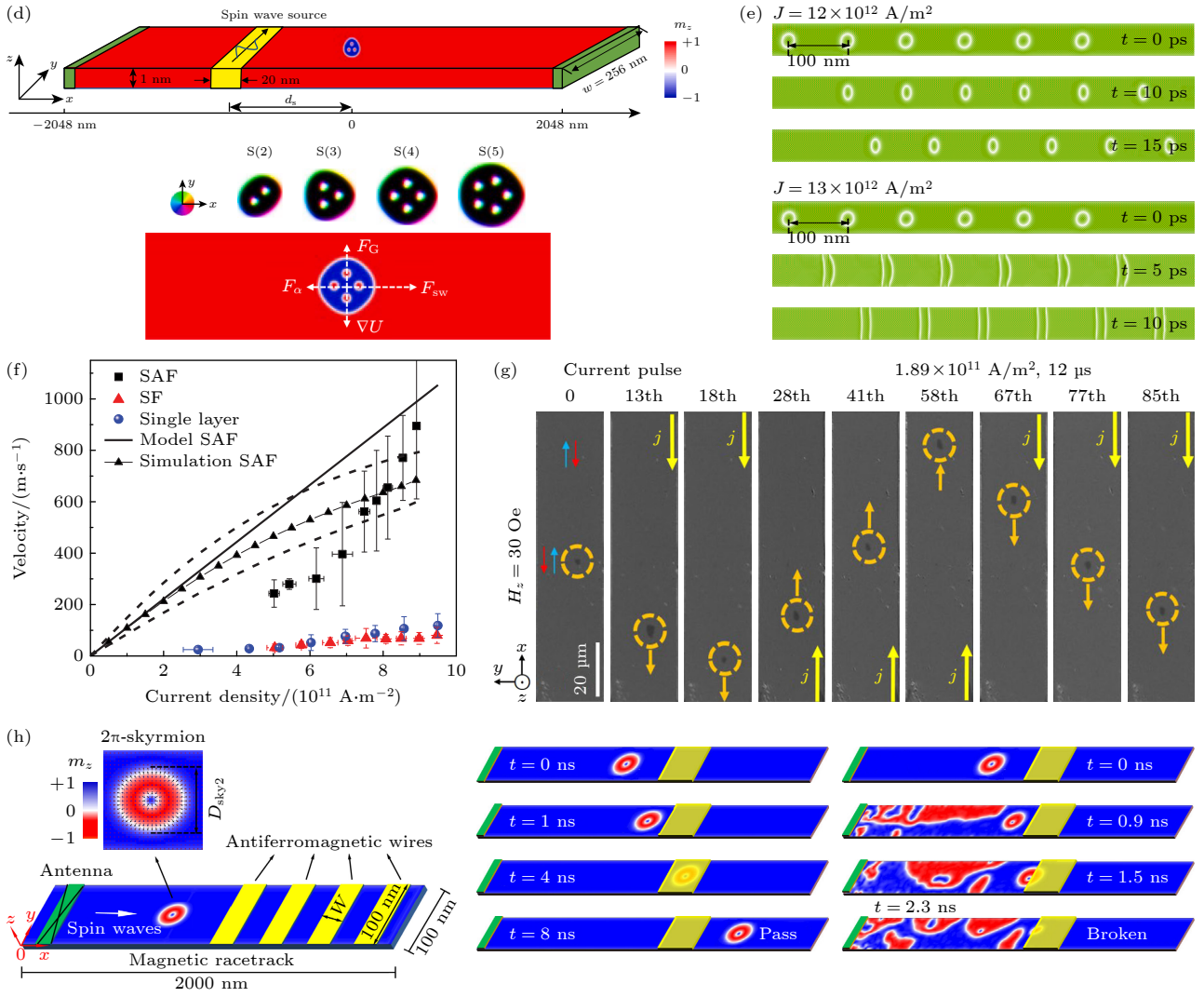
图 9 斯格明子赛道存储器 (a) 基于斯格明子的赛道存储器结构示意图 [94] ; (b) 有限宽度的纳米带中电流驱动斯格明子包的微磁学模拟 [97] ; (c) 斯格明子包在 VCMA 梯度下动力学的微磁学模拟 [98] ; (d) 自旋波驱动斯格明子包的微磁学模拟 [99] ; (e) 电流驱动 AFM 斯格明子链的微磁学模拟 [100] ; (f) SAF 斯格明子、单层铁磁斯格明子、双层人工合成斯格明子速度随电流密度的变化实验测量及 SAF 斯格明子的微磁学模拟 [72] ; (g) 电流驱动 SAF 斯格明子长距离直线往复运动 [43] ; (h) 自旋波驱动 2\pi 斯格明子的微磁学模拟 [101]
