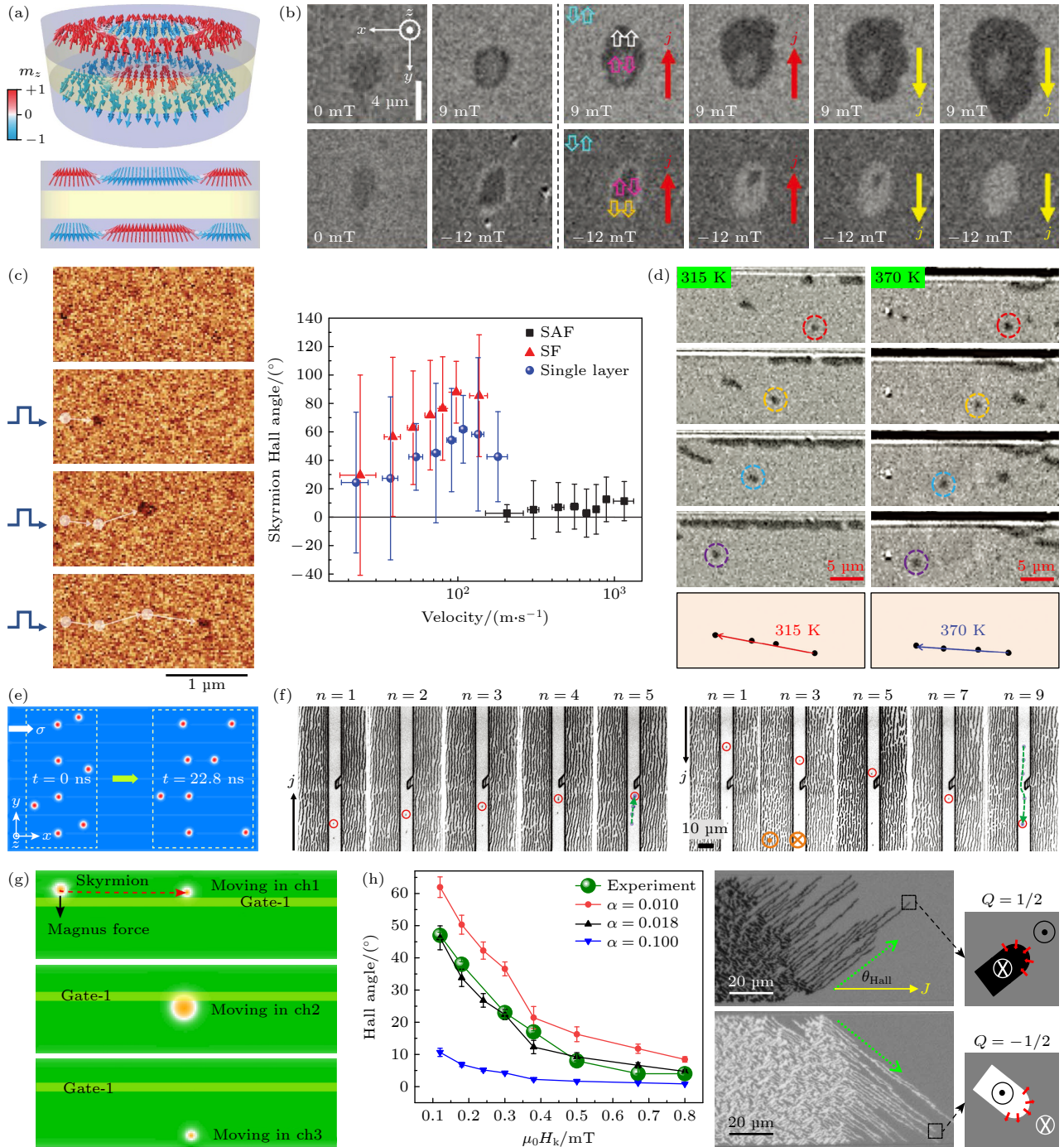
图6 斯格明子霍尔角的控制 (a) 双层人工反铁磁斯格明子结构示意图 [28] ; (b) SAF 斯格明子的验证与磁场解耦时电流驱动动力学 [48] ; (c) MFM 观测到电流驱动 SAF 斯格明子直线运动 [72] ; (d) 热效应调控螺旋度来减小斯格明子霍尔角 [73] ; (e) 基于心形斯格明子直线运动的赛道存储器微磁学模拟 [74] ; (f) 类二极管逻辑器件中带凹槽的辐照赛道内电流驱动的斯格明子运动 [75] ; (g) 在栅极施加电场时多通道赛道中斯格明子运动状态的微磁学模拟 [76] ; (h) 半斯格明子霍尔角的调控 [77]
