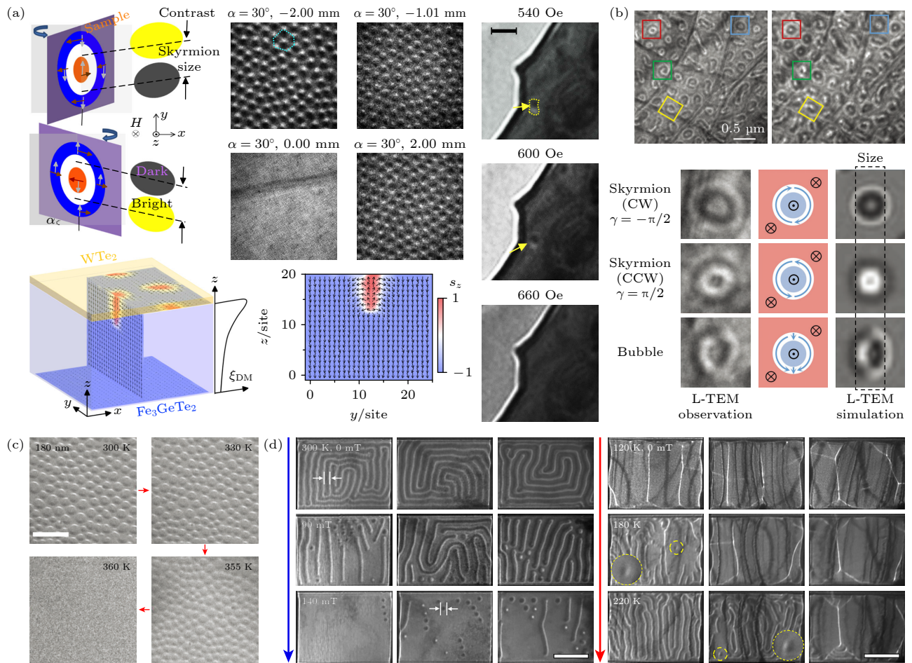
图 7 新型斯格明子载体材料 (a) \text{WTe}_2/\text{Fe}_3\text{GeTe}_2 范德瓦耳斯异质结中 Néel 型斯格明子的 L-TEM 图像 [38]; (b) 92 K 温度下 \text{Fe}_{5-\delta}\text{GeTe}_2 剥离薄片不同类型自旋结构的 L-TEM 实验图和模拟图 [37]; (c) 180 nm 厚度 \text{Fe}_3\text{GaTe}_2 纳米薄片中的零场斯格明子晶格 [39]; (d) 薄片厚度调控下偶极磁泡与半子-反半子对之间的相变规律 [40]
