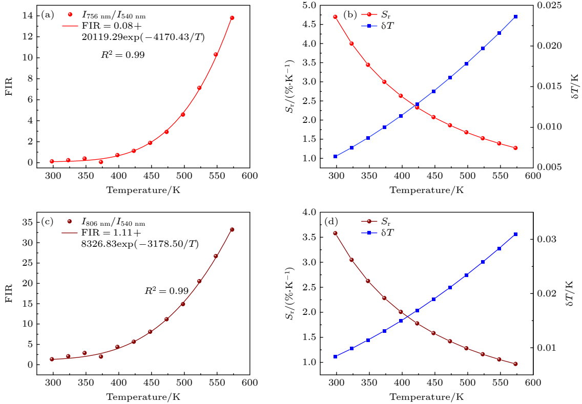
图 10 (a) \text{FIR}(I_{756 \text{ nm}}/I_{540 \text{ nm}}) 的温度依赖性实验值及其拟合曲线; (b) \text{FIR}(I_{756 \text{ nm}}/I_{540 \text{ nm}}) 的 S_r (左侧纵轴) 及 \delta T (右侧纵轴) 随温度变化的关系曲线; (c) \text{FIR}(I_{806 \text{ nm}}/I_{540 \text{ nm}}) 的温度依赖性实验值及其拟合曲线; (d) \text{FIR}(I_{806 \text{ nm}}/I_{540 \text{ nm}}) 的 S_r (左侧纵轴) 及 \delta T (右侧纵轴) 随温度变化的关系曲线
