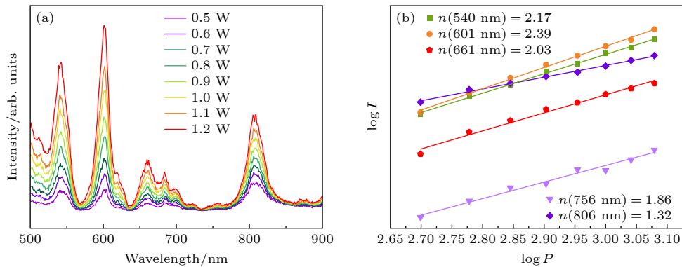
图 5 (a) 980 nm 激发下的 \text{ZnO}:\text{Nd}^{3+}/\text{Yb}^{3+} 上转换发光光谱随激发功率的变化关系 (激光功率: 0.5–1.2 W, 对应功率密度: 5–12 \text{W}/\text{cm}^2 ); (b) 540, 601, 661, 756 及 806 nm 处发射峰的 \log I 对 \log P 的依赖性关系
