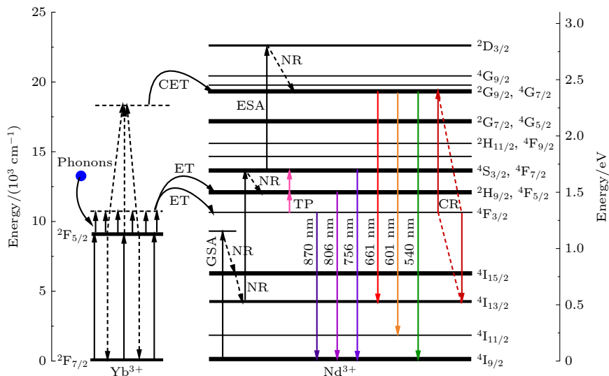
图 6 \text{Nd}^{3+} 和 \text{Yb}^{3+} 的激发和发射机理 ( \lambda_{\text{ex}} = 980 \text{ nm} )
