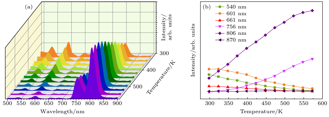
图 7 (a) 980 nm 激发下 ZnO:Nd 3+ /Yb 3+ 的温度依赖性三维发射光谱; (b) 540, 601, 661, 756, 806 及 870 nm 处发射峰强度对温度的依赖性关系
