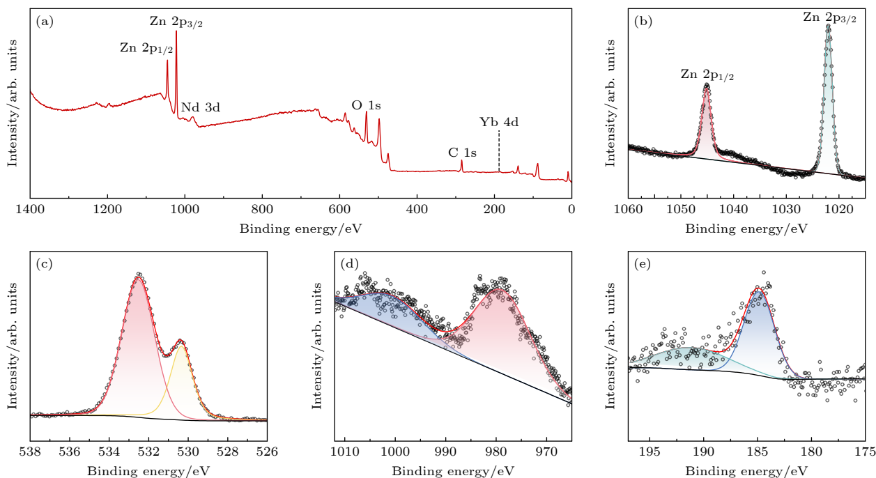
图 2 (a) ZnO:Nd 3+ /Yb 3+ 花状分级微米结构的 XPS 全扫描谱图; (b) Zn 2p, (c) O 1s, (d) Nd 3d 和 (e) Yb 4d 峰的 XPS 高分辨率图谱 Fig. 2. (a) XPS full scan spectrum of ZnO:Nd 3+ /Yb 3+ flower-like hierarchical microstructures; high-resolution XPS spectra of (b) Zn 2p, (c) O 1s, (d) Nd 3d, and (e) Yb 4d peak.
