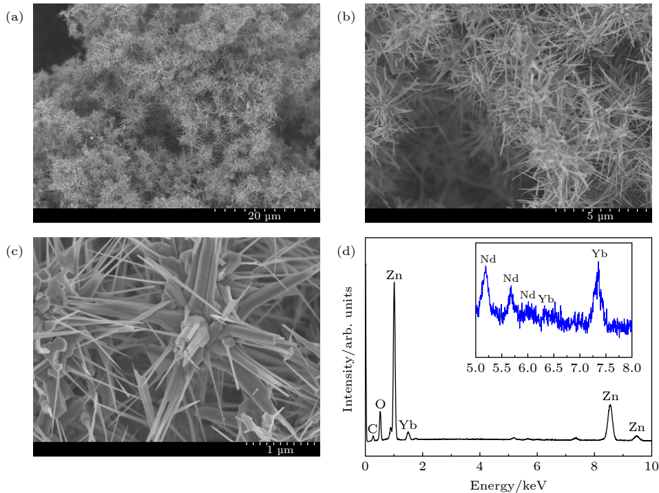
图 3 \text{ZnO:Nd}^{3+}/\text{Yb}^{3+} 花状分级微米结构 SEM 图像 (a) 低倍率; (b) 中倍率; (c) 高倍率. (d) EDS 能谱, 插图为 5.0—8.0 eV 范围的放大图
