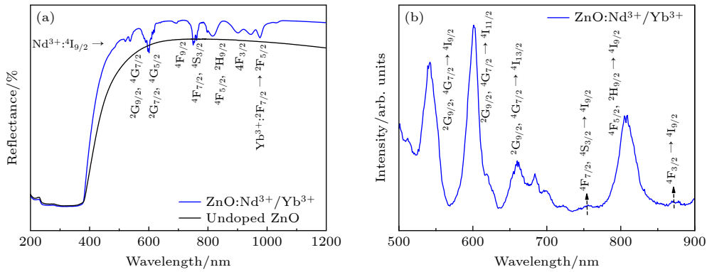
图 4 (a) 未掺杂的 ZnO 和 \text{ZnO}:\text{Nd}^{3+}/\text{Yb}^{3+} 花状分级微米结构的漫反射光谱; (b) 980 nm 激光激发下 \text{ZnO}:\text{Nd}^{3+}/\text{Yb}^{3+} 花状分级微米结构的上转换发光光谱
