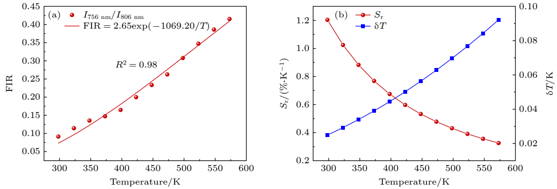
图 8 (a) FIR ( I_{756 \text{ nm}}/I_{806 \text{ nm}} ) 的温度依赖性实验值及其拟合曲线; (b) S_r (左侧纵轴) 及 \delta T (右侧纵轴) 随温度变化的关系曲线
