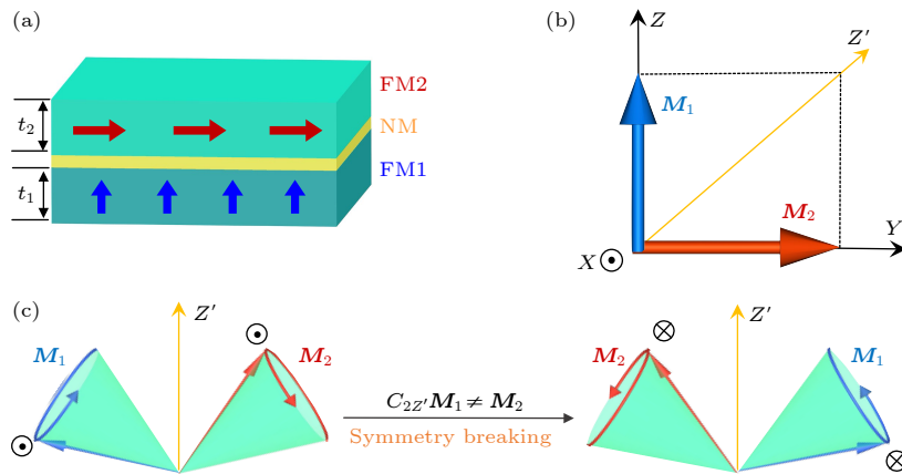
图 1 T 型构型和对称性破缺示意图 [41] (a) 非共线磁性多层膜的结构示意图; (b) 在 XYZ 坐标系中 FM1 和 FM2 的宏自旋平衡态示意图, \mathbf{M}_1 沿 Z 轴, \mathbf{M}_2 沿 Y 轴, 黄色箭头代表旋转轴的方向, Z' // (\mathbf{M}_1 + \mathbf{M}_2) ; (c) 对称性破缺示意图, 施加一个沿 Z' 轴的旋转对称性操作 C_{2Z'} , 旋转后的系统与旋转前的系统不等价, 即 C_{2Z'}\mathbf{M}_1 \neq \mathbf{M}_2
