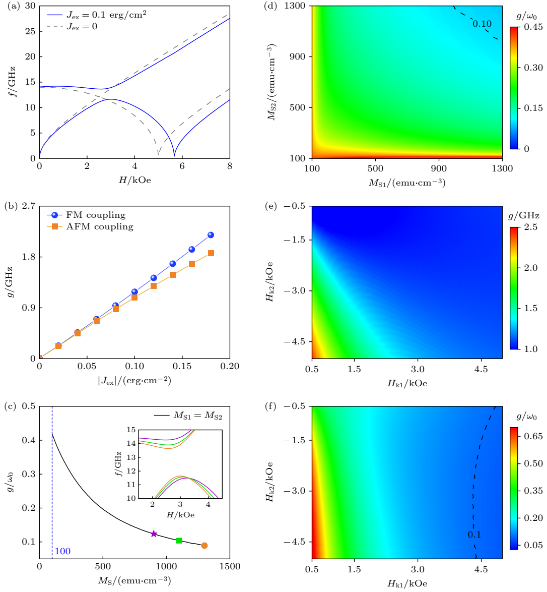
图 2 J_{\text{ex}} , M_s 和 H_k 对耦合强度和耦合率的影响 [41] (a) 非共线磁结构的频率色散关系; (b) 耦合强度与交换能密度的关系; (c) M_{s1} = M_{s2} 时, 耦合率随 M_s 的变化, 插图显示了色散关系中频率带隙的变化; (d) 耦合率的等高线图, 虚线 ( g/u_0 = 0.1 ) 表示超强耦合区的边界; (e) 耦合强度和 (f) 耦合率随 H_{k1} 和 H_{k2} 变化的等高线图
