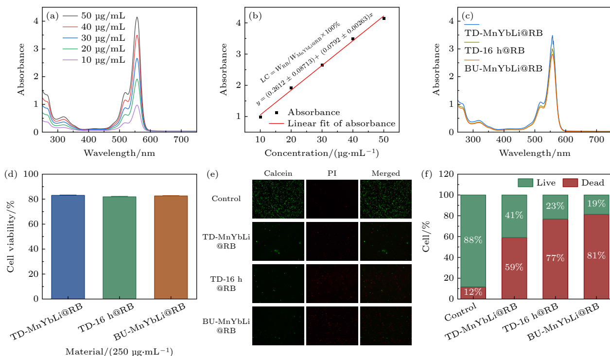
图5 光动力性能表征 (a) 不同浓度RB溶液的紫外-可见吸收光谱 [8] ; (b) 根据(a)图547 nm吸收峰强度描绘其随RB浓度变化的线性拟合曲线 [8] ; (c) TD-MnYbLi, TD-16 h及BU-MnYbLi负载RB过程中离心洗涤后的上清液(稀释10倍)的吸收光谱; (d) CCK-8法测得的细胞活力; (e) 经254 nm紫外光照射10 min后与HeLa细胞共培养12 h的Calcein-AM/PI活-死染色共聚焦图像; (f) 对应细胞存活率与死亡率统计结果
