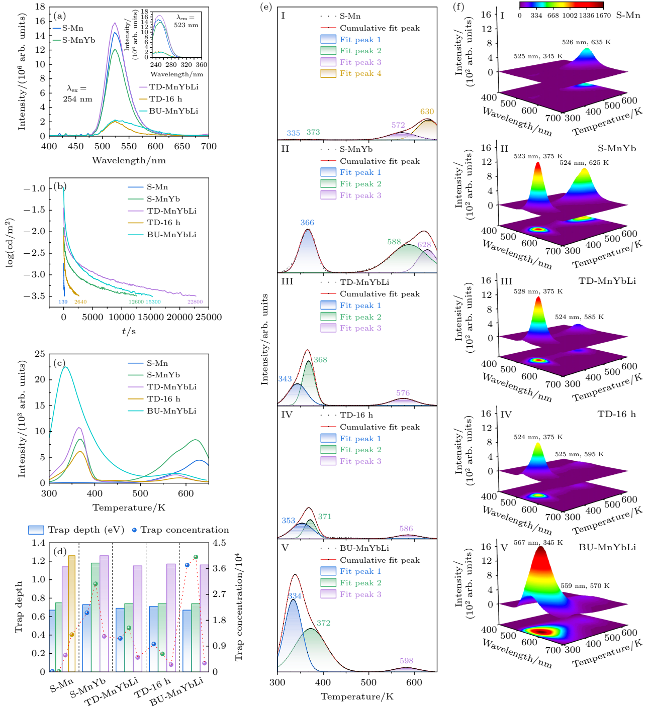
图 3 S-Mn, S-MnYb, TD-MnYbLi, TD-16 h 及 BU-MnYbLi 样品的发光与陷阱行为 (a) 发射光谱 ( \lambda_{\text{ex}} = 254 nm) 及激发光谱 ( \lambda_{\text{em}} = 523 nm); (b) 余辉亮度衰减曲线 (254 nm 紫外光预激发 5 min); (c) 热释光谱 (254 nm 紫外灯预激发 5 min); (d) 由热释光分峰拟合得到的陷阱深度与陷阱浓度; (e) 热释光谱高斯分峰拟合结果; (f) 三维热释光谱 (254 nm 紫外灯预激发 5 min)
