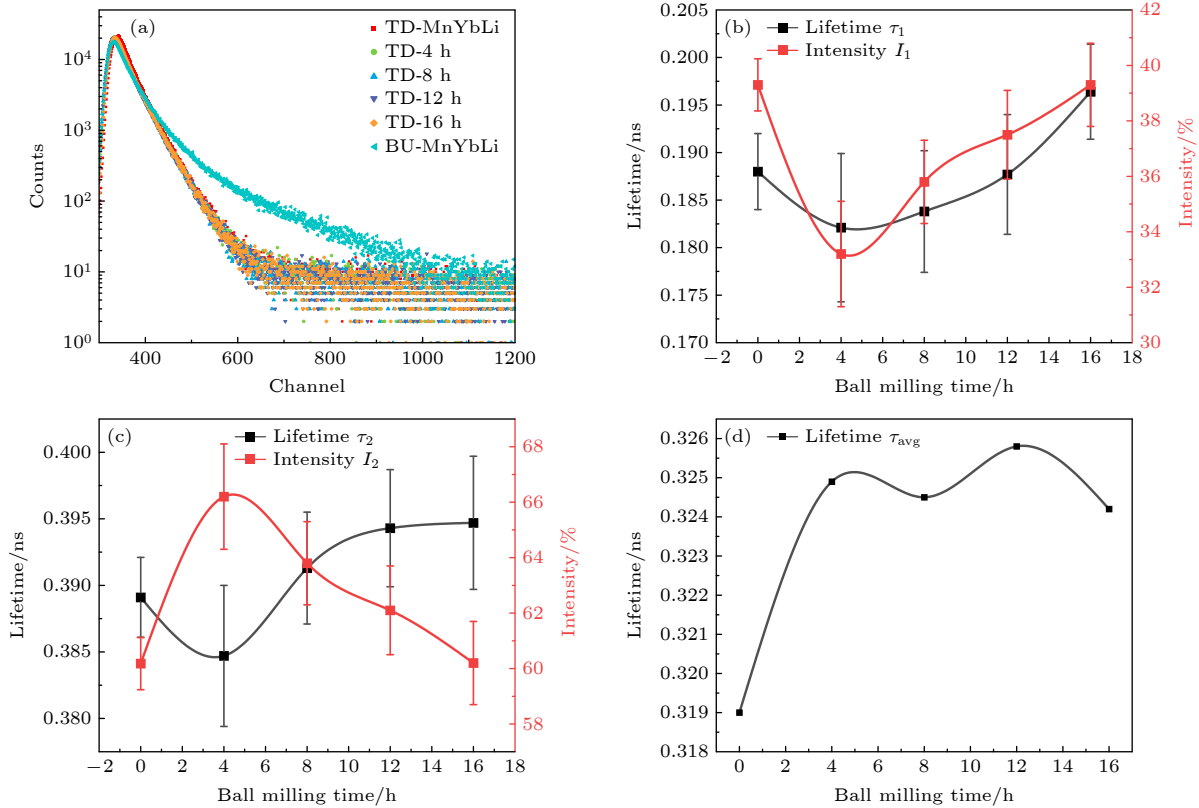
图4 TD-MnYbLi, TD-4 h, TD-8 h, TD-12 h, TD-16 h 及 BU-MnYbLi 样品的正电子湮没寿命谱及解谱结果 (a) 正电子湮没寿命谱; (b) \tau_1 与 I_1 随球磨时间的变化; (c) \tau_2 与 I_2 随球磨时间的变化; (d) 平均寿命 \tau_{avg} 随球磨时间的变化
