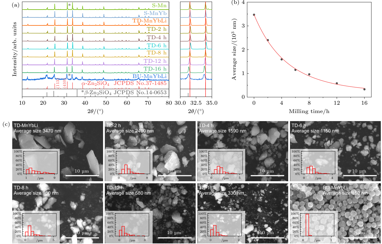
图 1 (a) S-Mn, S-MnYb, TD-MnYbLi, TD-2 h–16 h 及 BU-MnYbLi 样品的 XRD 图谱, 右侧为 (113) 与 (410) 晶面的局部放大图; (b) TD-MnYbLi 样品平均粒径随球磨时间的变化关系; (c) TD-MnYbLi, TD-2 h–16 h 及 BU-MnYbLi 样品的 SEM 形貌图及对应粒径分布统计图
