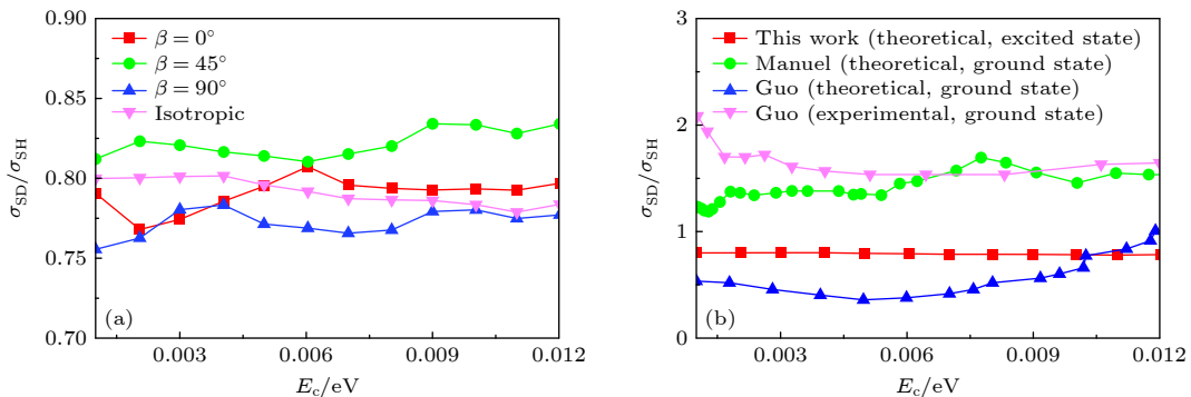
图 3 (a) 不同初始 HD 取向 ( \beta = 0^\circ, 45^\circ, 90^\circ 及各向同性) 下, 反应通道的 \sigma_{SD}/\sigma_{SH} 随碰撞能的变化关系; (b) 各向同性下的 \sigma_{SD}/\sigma_{SH} 与文献结果对比
