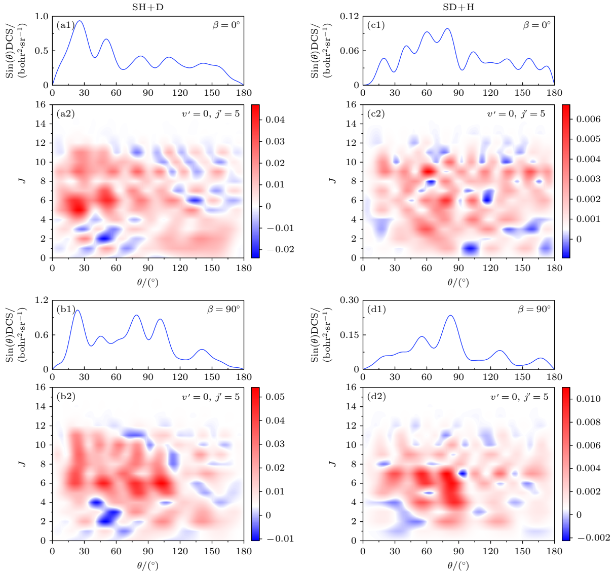
图 8 E_c = 0.001 eV 时, 两产物的态分辨 DCS 与量子广义偏转函数 (a), (b) 属于 SH 产物; (c), (d) 属于 SD 产物
