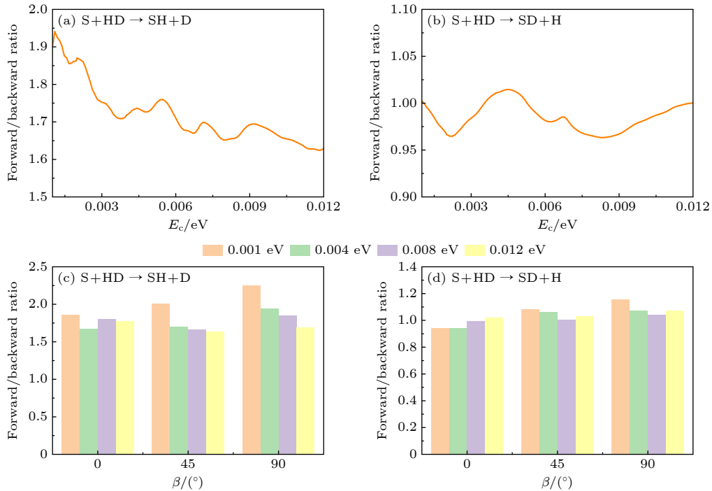
图 6 (a) S(^1D) + HD \rightarrow SH + D 反应总 DCS 的 F/B 比值随碰撞能量的变化关系; (b) S(^1D) + HD \rightarrow SD + H 反应总 DCS 的 F/B 比值随碰撞能量的变化关系; (c) 不同初始 HD 取向下的 S(^1D) + HD \rightarrow SH + D 反应总 DCS 的 F/B 比值于多个碰撞能量下的结果; (d) 不同初始 HD 取向下的 S(^1D) + HD \rightarrow SD + H 反应总 DCS 的 F/B 比值于多个碰撞能量下的结果
