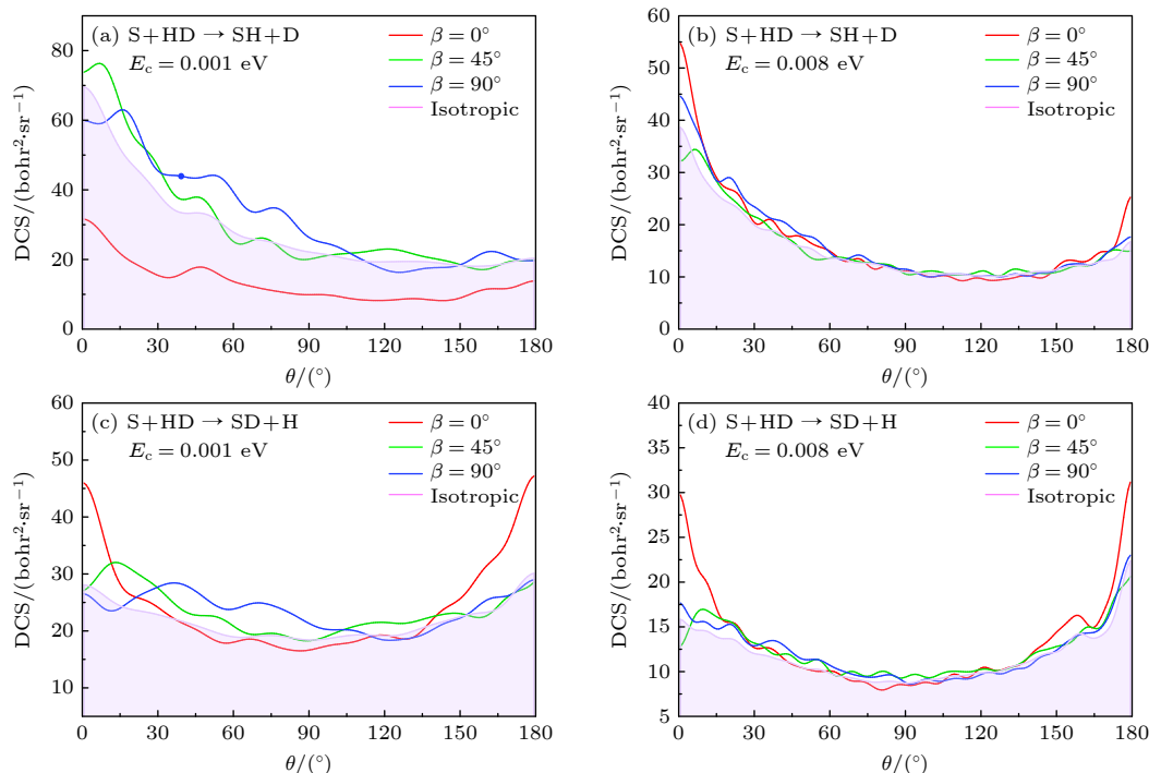
图 5 在两个特定碰撞能下, 不同初始 HD 取向时, S(^1D) + HD 反应的总 DCS 随散射角的变化关系 (a) 在 E_c = 0.001 eV 时, SH 通道; (b) 在 E_c = 0.008 eV 时, SH 通道; (c) 在 E_c = 0.001 eV 时, SD 通道; (d) 在 E_c = 0.008 eV 时, SD 通道
