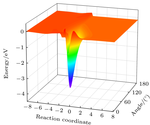
图 1 S( 1 D) + HD ( v=1, j=2 ) → SH + D/SD + H 反应的最低能量路径
