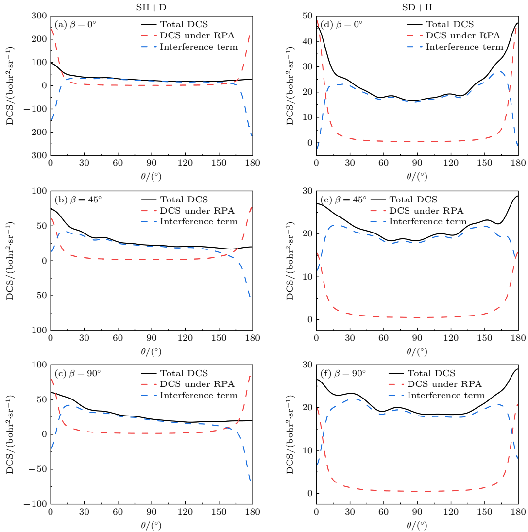
图 7 E_c = 0.001 eV 时, 不同初始 HD 取向, 两个反应通道的总 DCS (黑色实线)、RPA 下的 DCS (红色虚线) 以及干扰项 (蓝色虚线) 随散射角的变化关系 (a)–(c) 属于 SH 通道; (d)–(f) 属于 SD 通道
