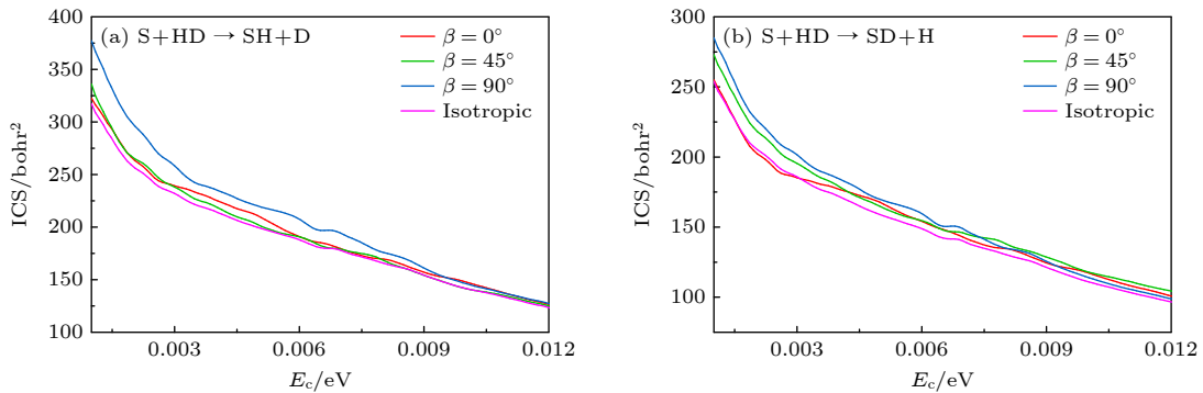
图 2 不同初始 HD 取向, S( 1 D) + HD 反应的总 ICS 随碰撞能的变化关系 (a) 属于 SH 通道; (b) 属于 SD 通道
