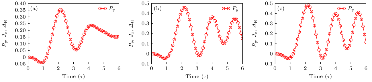
图6 不同系统尺寸下, 横向自旋极化 P_y(\tau) 随时间的变化 (a) L = 20 ; (b) L = 40 ; (c) L = 60 ; 其他参数 \lambda_R = 0.6 , \Delta_\mu = 0.2 和 N = 4
