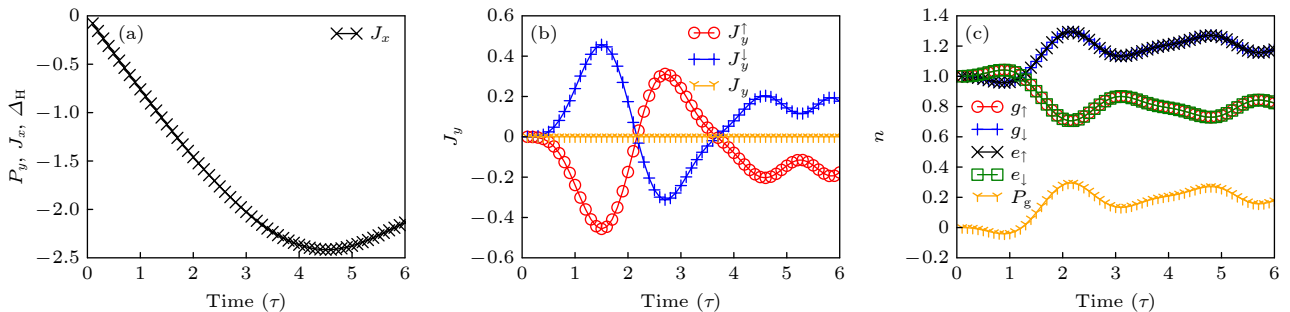
图 3 (a) 纵向原子流 J_x 随时间的变化; (b) 横向自旋流 J_y 随时间的变化; (c) 不同自旋分量的粒子数 n 及横向自旋极化 P_y 随时间的变化; 参数为 \lambda_R = 0.6 , \Delta_\mu = 0.2 , K = 0.0002 , L = 20 和 N = 4
