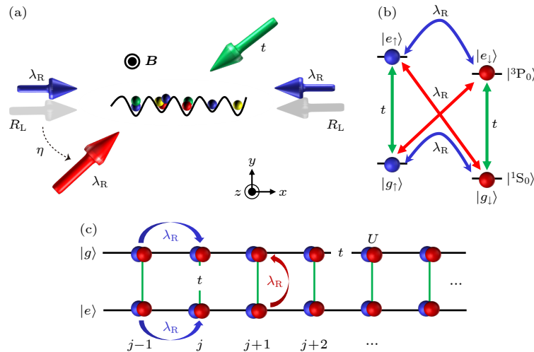
图 1 理论方案及有效模型示意图 (a) 灰色箭头 R_L 表示两束沿 x 方向反向传播的光, 用于形成一维光学晶格; B 表示外加磁场, 用于定义自旋量子化轴; 红色、绿色和蓝色箭头表示耦合原子内态的激光; (b) |g\rangle 和 |e\rangle 表示两个长寿命轨道态, \uparrow 和 \downarrow 表示自旋态; 绿色箭头 t 诱导轨道态间的自旋不变跃迁, 红色箭头 \lambda_R 表示单光子拉比震荡诱导的轨道态间的自旋翻转跃迁, 蓝色箭头 \lambda_R 表示双光子拉曼过程诱导的同轨道态的自旋翻转跃迁; (c) 准一维格点模型, 其中灰色和绿色连线分别表示 x 和 y 两个方向的近邻跃迁 t , 蓝色和红色箭头分别表示 Rashba 自旋轨道耦合的两个方向的自旋翻转跃迁 \lambda_R , U 表示同格点的接触型相互作用
