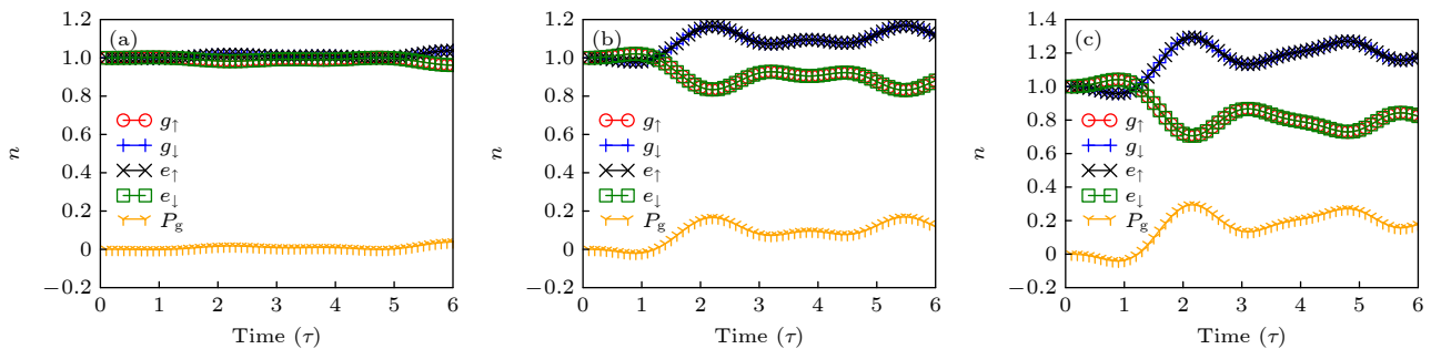
图5 不同线性势强度 \Delta_\mu 下,各组分的原子数 n 和横向极化 P_y 随时间的变化 (a) \Delta_\mu = 0.01 ; (b) \Delta_\mu = 0.1 ; (c) \Delta_\mu = 0.2 ; 其他参数为 \lambda_R = 0.6 , L = 20 和 N = 4
