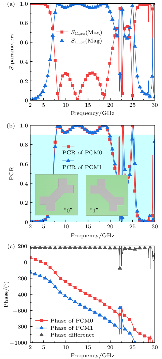
图 7 极化转换超表面单元仿真结果 (a) 状态“0”单元 S 曲线; (b) 两种状态单元极化转换率; (c) 两种单元反射波相位
