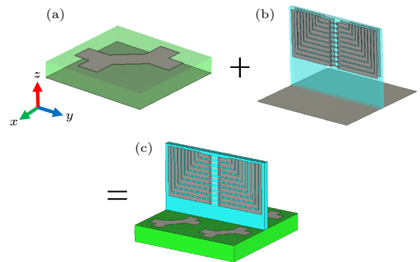
图 9 复合超表面结构 (a) PCM 单元; (b) SSPP 吸波器单元; (c) 复合超表面单元
