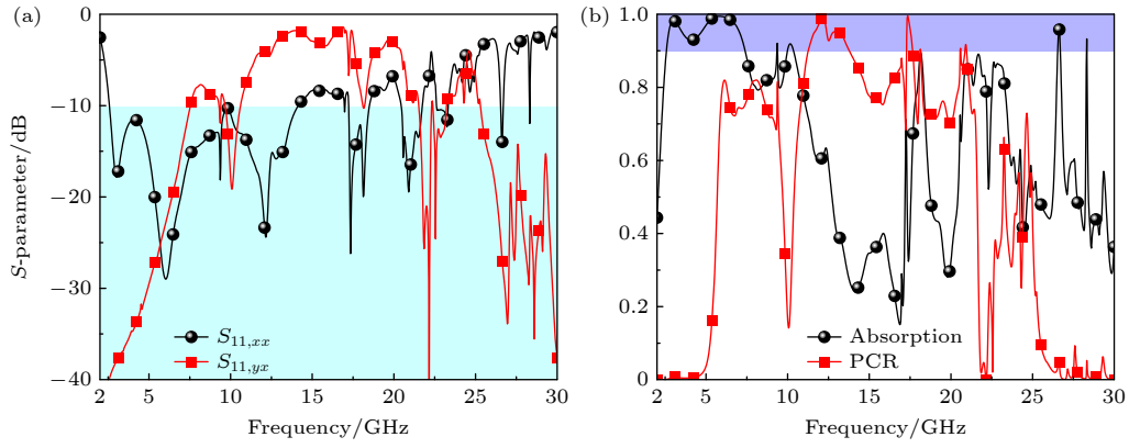
图 10 复合超表面单元仿真结果 (a) S 曲线; (b) 吸波率和 PCR
