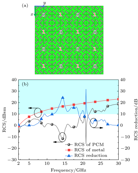
图 8 棋盘 PCM 阵列示意图及 RCS 仿真结果 (a) 阵列结构; (b) RCS 结果
