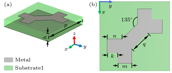
图 6 极化转换超表面示意图 (a) 三维示意图; (b) 俯视图 Fig. 6. Schematic of the polarization conversion metasurface: (a) 3D view; (b) top view.
