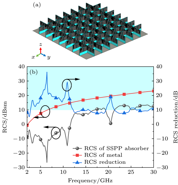
图 5 SSPP 吸波器阵列示意图及 RCS 仿真结果 (a) 阵列示意图; (b) RCS 结果
