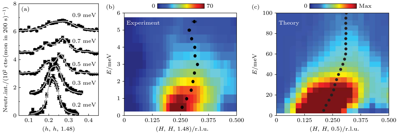
图 17 (a) A 型 \text{CeCu}_2\text{Si}_2 在 0.4 K 下恒定能量的中子散射扫描 [62] ; (b) S 型 \text{CeCu}_2\text{Si}_2 在 1.6 K 下 1.38 < L < 1.58 范围内数据对应的能量-动量谱 [56] ; (c) 结合 LDA + U 能带结构, 通过 RPA (随机相位近似) 计算得到的能量-动量谱 [56] Fig. 17. (a) Constant-energy neutron scattering scans of A-type \text{CeCu}_2\text{Si}_2 at 0.4 K [62] ; (b) energy-momentum spectrum of S-type \text{CeCu}_2\text{Si}_2 at 1.6 K obtained from the data within 1.38 < L < 1.58 [56] ; (c) energy-momentum spectrum calculated within the random phase approximation (RPA) using the LDA + U band structure [56] .
