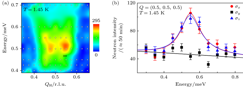
图 4 (a) CeCoIn 5 超导态 ( T = 1.45 K) 中沿 Q = (Q_H, Q_H, 0.5) 方向的非弹性中子散射强度分布 [35] ; (b) Q_{AF} = (0.5, 0.5, 0.5) 处 3 个极化通道 ( \sigma_x, \sigma_y, \sigma_z ) 的极化中子散射谱 [35]
