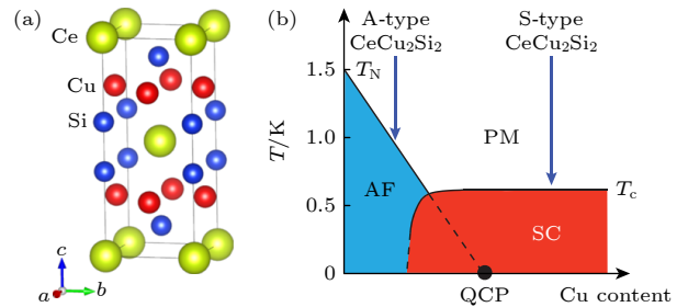
图 13 (a) CeCu 2 Si 2 的四方 ThCr 2 Si 2 型晶体结构; (b) CeCu 2 Si 2 的相图示意图, 其中标出了 A 型 (反铁磁) 与 S 型 (超导) 区域 [22,56] Fig. 13. (a) Tetragonal ThCr 2 Si 2 -type crystal structure of CeCu 2 Si 2 ; (b) schematic phase diagram of CeCu 2 Si 2 , where the A-type (antiferromagnetic) and S-type (superconducting) regions are indicated [22,56] .
