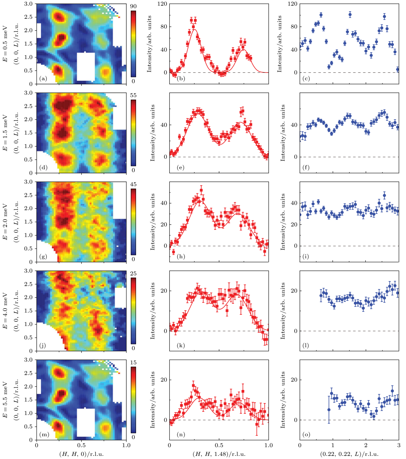
图 16 \text{CeCu}_2\text{Si}_2 正常态 ( T = 1.6 K) 不同能量的 HHL 切片, E = 0.5, 1.3, 2.0, 3.1, 4.0, 5.5 meV [56] , 低能 ( E \lesssim 1.5 meV) 激发表现出显著的 L 依赖, 高能 ( E \gtrsim 2 meV) 激发变得不依赖 L , 即演化为了准二维磁激发
