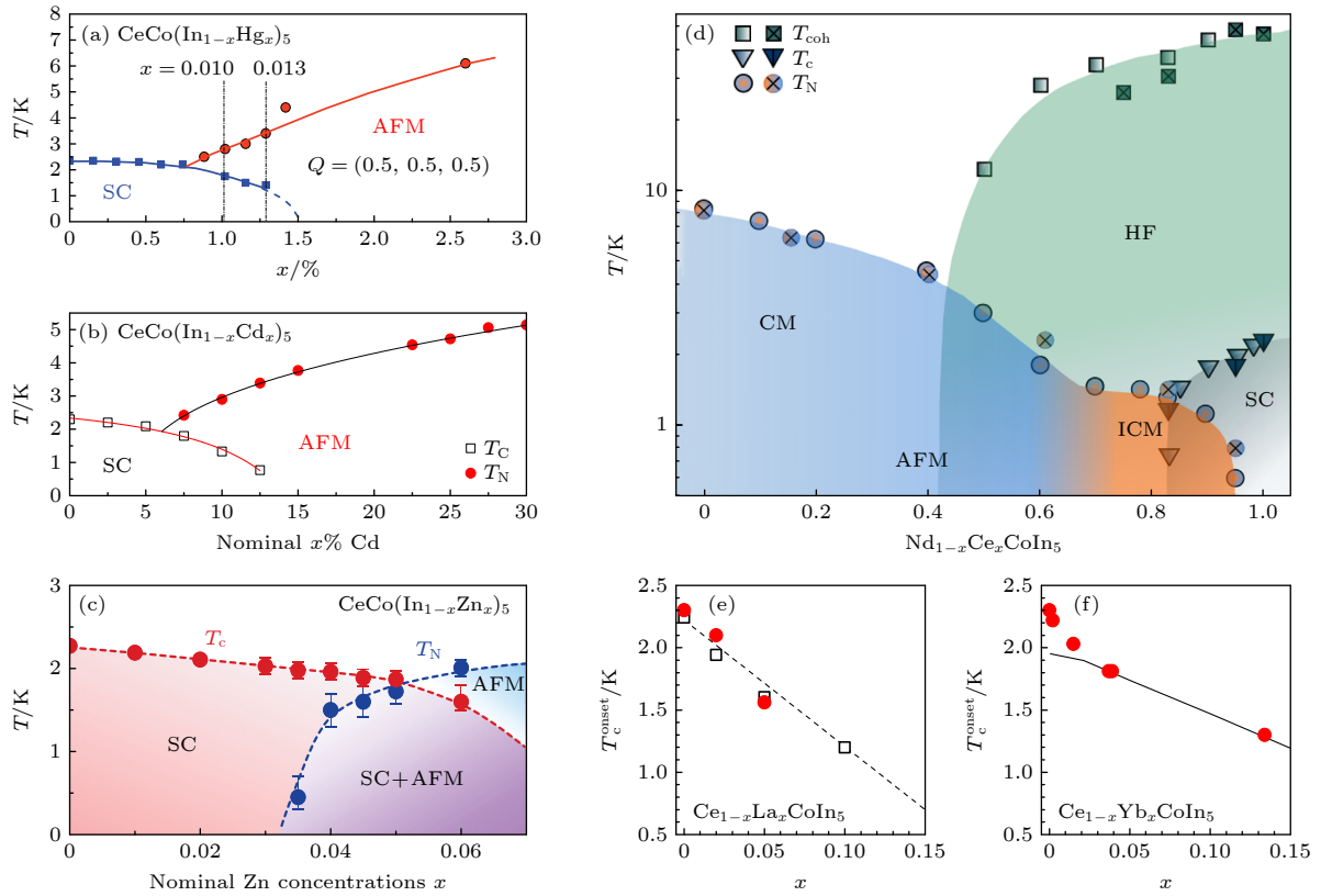
图 8 \text{CeCoIn}_5 在 (a) Hg [28] , (b) Cd [26] , (c) Zn [44] , (d) Nd [45] , (e) La [46] , (f) Yb [46] 掺杂下的相图; 其中 Yb 的组分为实际掺杂 x_{\text{act}} , 其对 T_c 的抑制速率与 La 掺杂相似; Nd 掺杂相图中包括调制波矢为 (0.5, 0, 0.5)/(0, 0.5, 0.5) 的公度 (commensurate, CM) 反铁磁相和调制波矢为 (q, q, 0.5) 的非公度 (incommensurate, ICM) 反铁磁相, 其中 q \approx 0.44 [45] ; Hg, Cd, Zn 掺杂相图中反铁磁序的调制波矢均为 (0.5, 0.5, 0.5)
