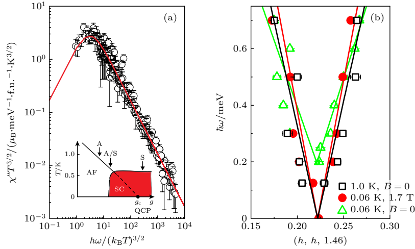
图 15 (a) S 型 \text{CeCu}_2\text{Si}_2 正常态 ( B = 1.7 T) 在 Q_{\text{AFM}} 处的动态磁化率, \chi''(E, T) \cdot T^{3/2} 作为 E/T^{3/2} 的函数塌缩到一条线上 [61] ; (b) 超导态与正常态色散的对比如 [61]
