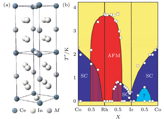
图 1 (a) CeCoIn_5 的四方 HoCoGa_5 型晶体结构; (b) CeMIn_5 ( M = Co, Rh, Ir ) 体系的温度-元素替换相图 [3]
