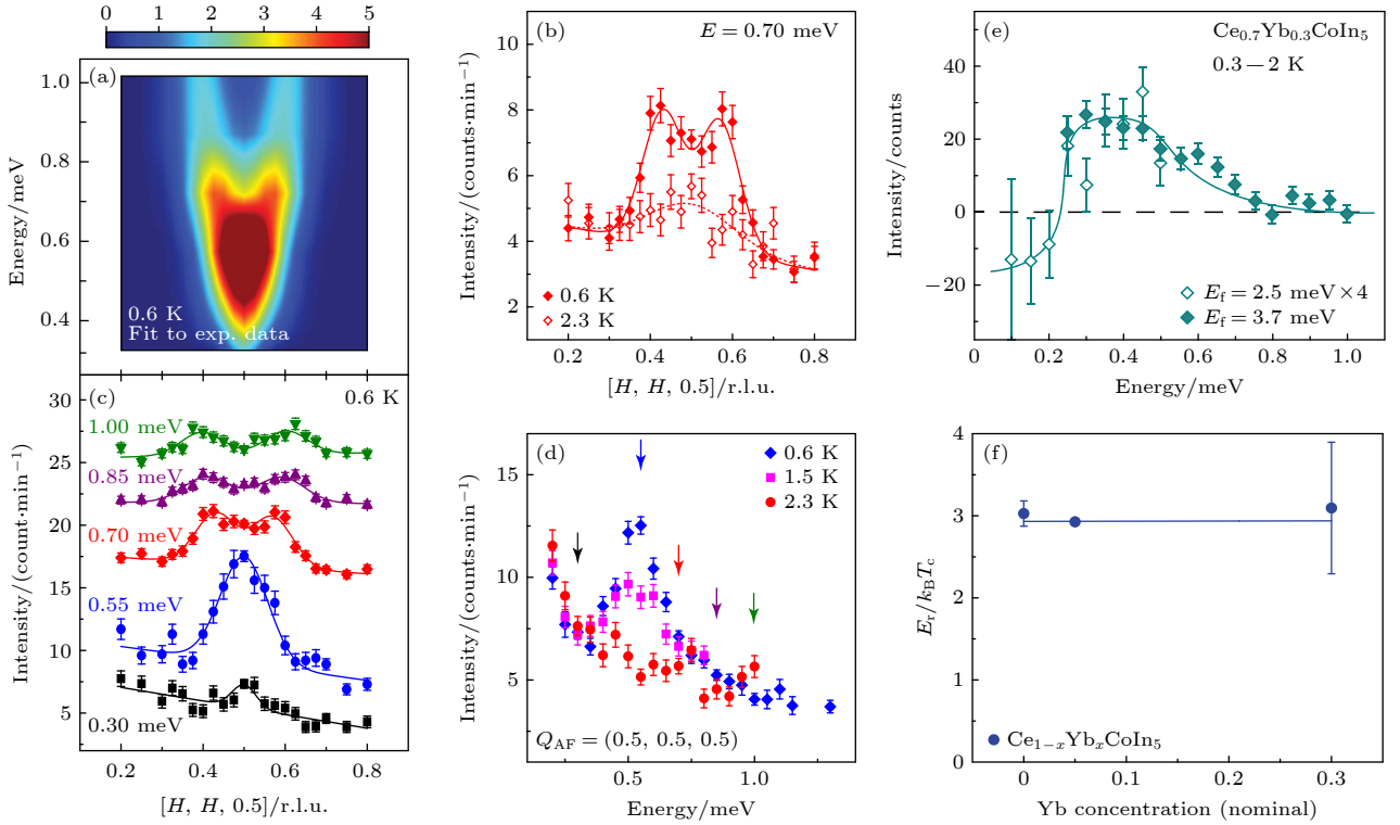
图 11 \text{Ce}_{1-x}\text{Yb}_x\text{CoIn}_5 中的自旋共振模 [39] , 名义组分 x = 0.05 样品 (a) 对图 (c) 中数据的拟合结果; (b) 0.6 K 和 2.3 K 下 E = 0.70 meV 的 (H, H, 0.5) 方向散射强度对比; (c) 0.6 K 下 E = 0.30 meV, 0.55 meV, 0.70 meV, 0.85 meV, 1 meV 的 (H, H, 0.5) 方向散射强度; (d) 0.6 K, 1.5 K 和 2.3 K 下 (0.5, 0.5, 0.5) 处沿着能量的散射强度; 名义组分 x = 0.3 样品 (e) 自旋共振模能谱; (f) E_r/k_B T_c 随 Yb 掺杂的变化
