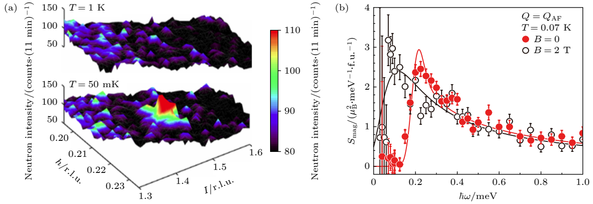
图 14 (a) A 型 \text{CeCu}_2\text{Si}_2 在 T = 50 mK 和 1 K 倒空间 (HHL) 平面的中子衍射强度图 [57] ; (b) S 型 \text{CeCu}_2\text{Si}_2 在 Q_{\text{AFM}} 处超导态 ( T = 0.07 K, B = 0 ) 与正常态 ( B = 2 T) 的磁激发谱 [58]
