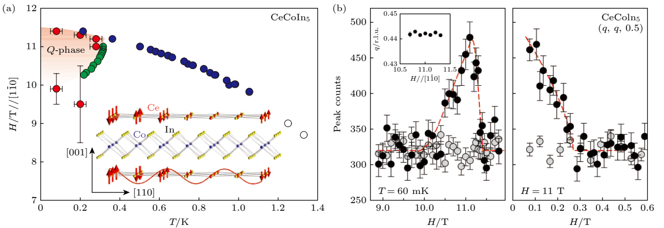
图3 (a) CeCoIn 5 的温度-磁场相图; (b) (q, q, 0.5) 位置中子散射的磁场和温度依赖, 其中 q \approx 0.44 [14]
