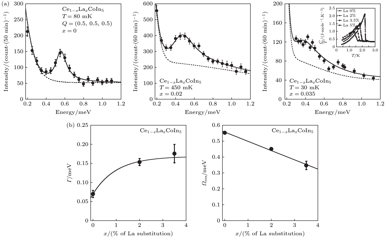
图 10 (a) \text{Ce}_{1-x}\text{La}_x\text{CoIn}_5 在 Q_{\text{AF}} = (0.5, 0.5, 0.5) 处的非弹性中子散射谱; (b) 拟合得到的自旋共振弛豫率和能量随掺杂的变化 [50]
