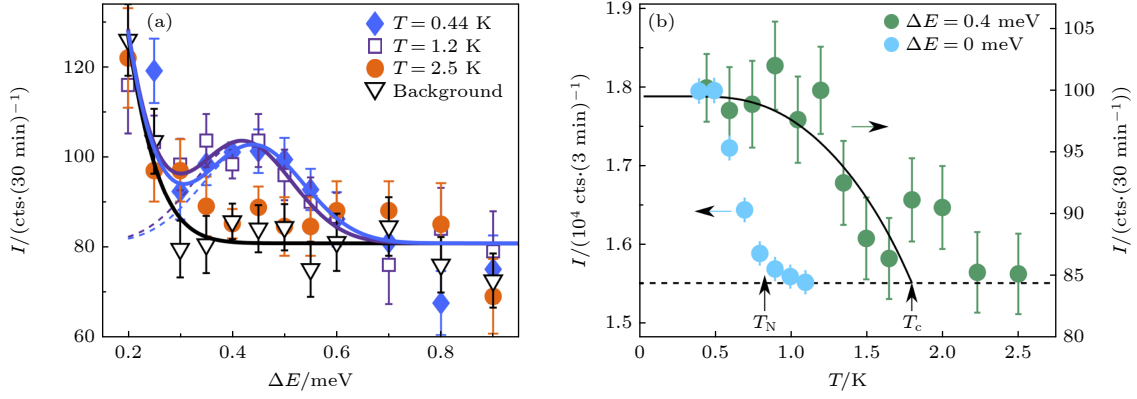
图 9 (a) \text{Ce}_{0.95}\text{Nd}_{0.05}\text{CoIn}_5 在 Q = (0.5, 0.5, 0.5) 处, T = 0.44 K, 1.2 K 和 2.5 K 下的非弹性中子散射谱; (b) 非公度磁序的弹性散射 ( 0 meV) 和自旋共振模在 0.4 meV 处的温度依赖 [48]
