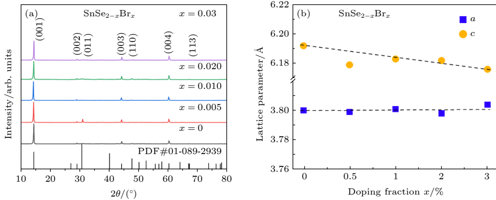
图 S1 \text{SnSe}_{2-x}\text{Br}_x ( x = 0, 0.005, 0.01, 0.02, 0.03 ) 的 (a) 室温 XRD 和 (b) 晶格常数
