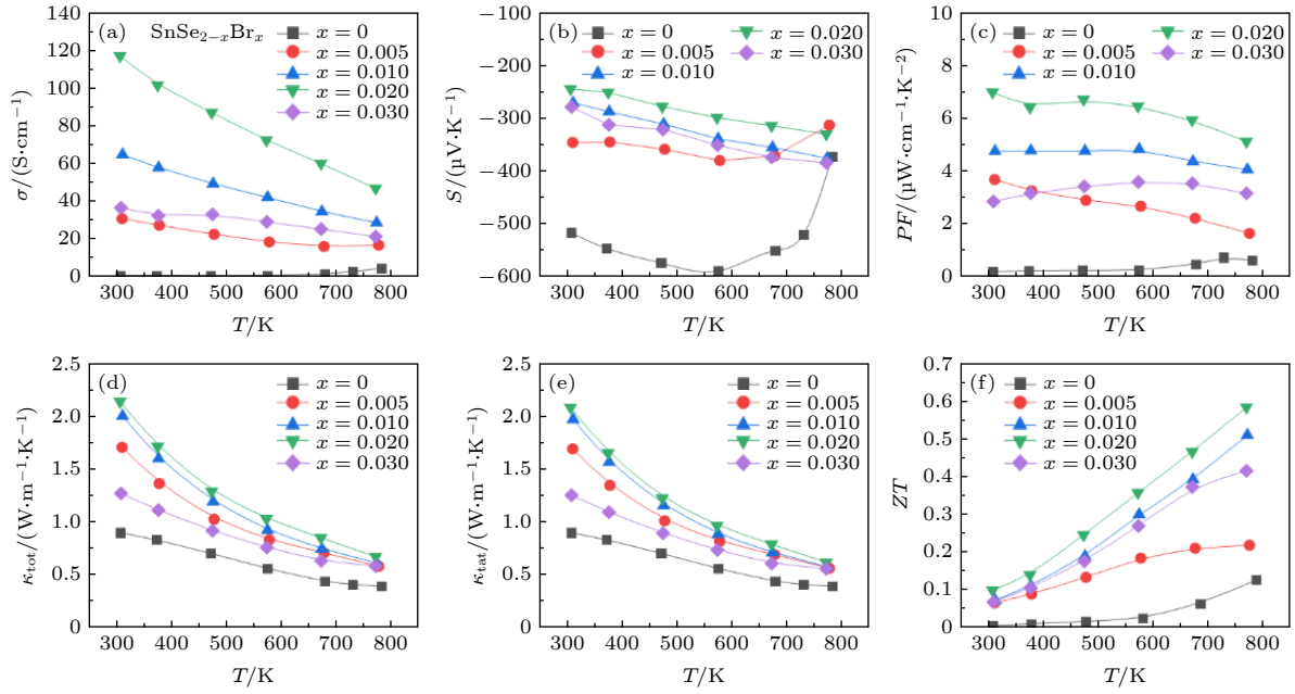
图 S3 样品 \text{SnSe}_{2-x}\text{Br}_x 沿 // P 方向的 (a) 电导率; (b) Seebeck 系数; (c) 功率因子; (d) 总热导率; (e) 晶格热导率和 (f) ZT 值随温度的变化
