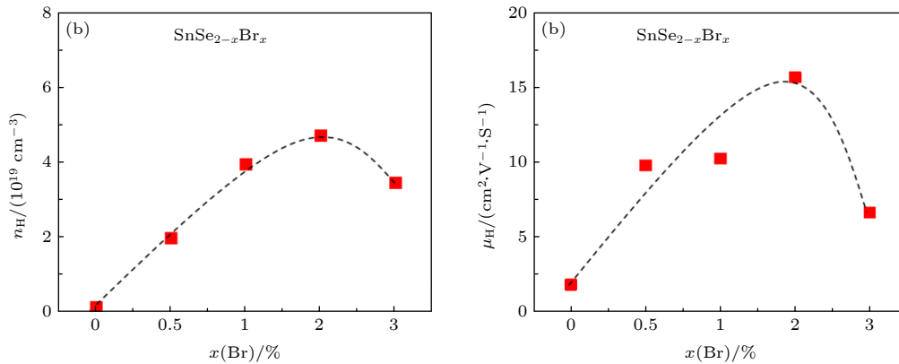
图 S2 样品 \text{SnSe}_{2-x}\text{Br}_x 沿 // P 方向的 (a) 载流子浓度和 (b) 载流子迁移率随掺杂浓度的变化
