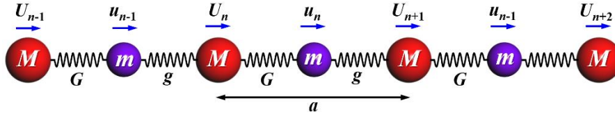
图 S1 一维双原子链
