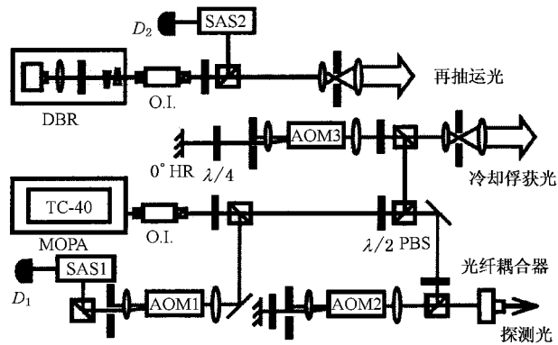
图 2 铯原子磁光阱的光路系统示意图( DBR 为分布布拉格反射式半导体激光器; OI 为光隔离器; SAS 为饱和吸收装置; AOM 为声光调制器; D 为光电探测器; PBS 为偏振分光棱镜; HR 为高反镜)
