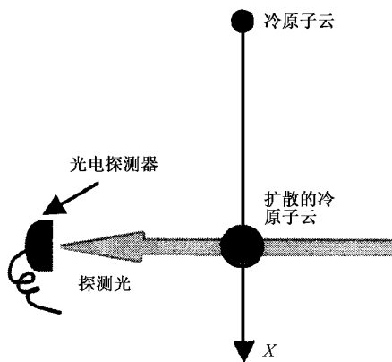
图 1 短程飞行时间吸收谱方案示意图
