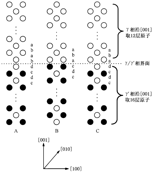
图 2 \gamma/\gamma' 相界面上的三种界面构型
