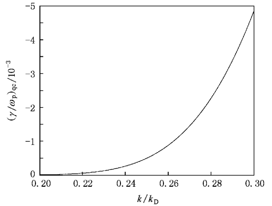
图3 量子效应对电子朗道阻尼的修正 (\gamma/\omega_p)_q 随 k/k_D 的变化曲线
