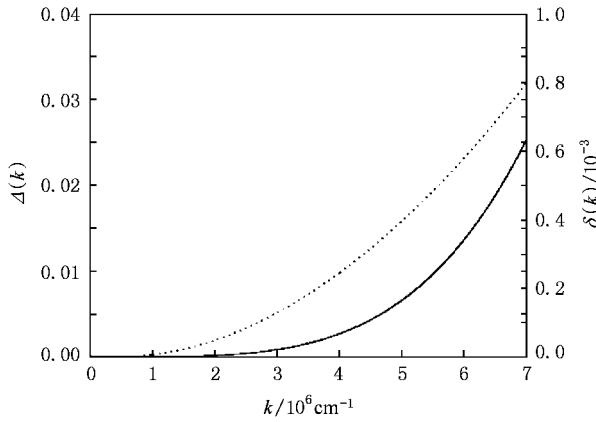
图1 实线表示量子效应对电子等离子体波频率的修正 \Delta(k) , 虚线表示量子效应对光子朗道阻尼的修正 \delta(k) . 等离子体参数为: 电子数密度 n_0 \sim 10^{19} \text{ cm}^{-3} , 温度 T = 300\text{K}
