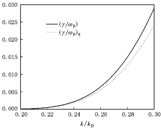
图2 实线表示经典的电子朗道阻尼曲线,虚线表示考虑量子效应后电子朗道阻尼曲线
