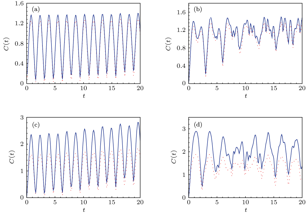
图 2 concurrence (实线) 和约化 Neumann 熵 (点线) 的时间演化, 其中 g = 1, p = 1: \gamma = 0.02 ((a),(c)); \gamma = 0.25 ((b),(d)); N = 3 ((a),(b)); N = 6 ((c),(d))
